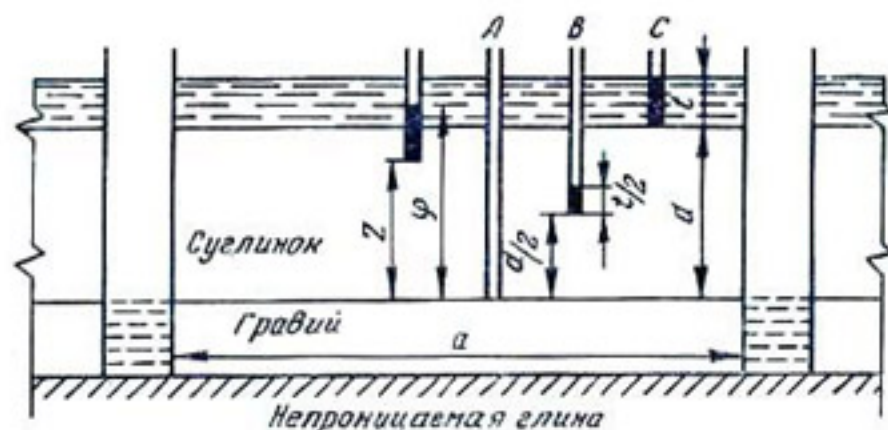
Рис. 70. Прямолинейное вертикальное просачивание воды в гравий, перерезанный дренажными каналами; пьезометры показывают давление воды и гидравлический напор.
