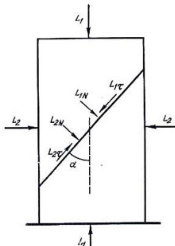
Рис. 14. Схема разрушения почвенной колонки под действием сил L_1 и L_2 .
