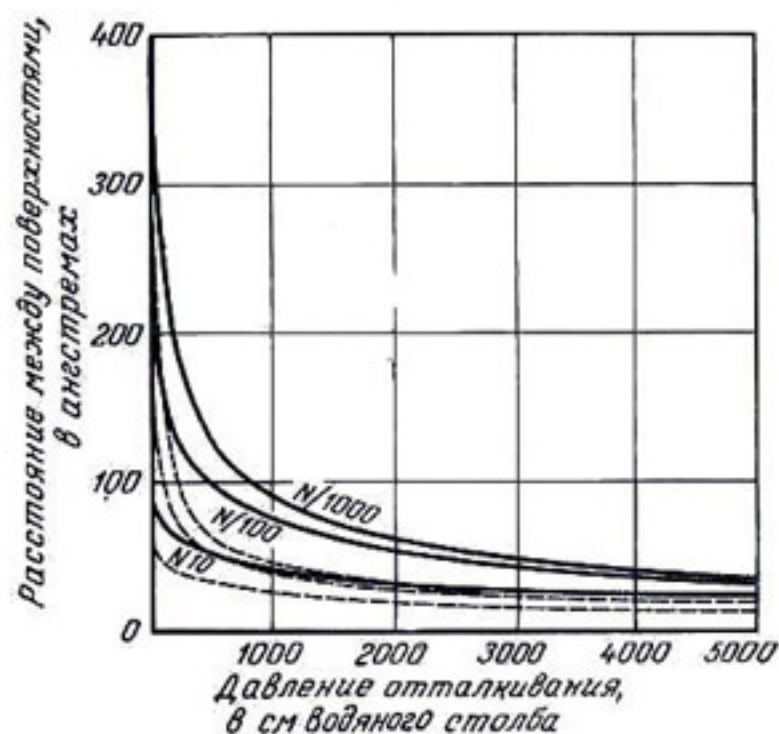
Рис. 8. Давление отталкивания между монтмориллонитовыми пластинками, показанными на рисунке 7, как функция расстояния между этими пластинками. Сплошные кривые построены для кристаллов в растворах одновалентных ионов указанных концентраций. Штриховые кривые — для двухвалентных ионов таких же трех концентраций. Во избежание путаницы показатели концентраций опущены, но они расположены в том же порядке, как и на кривых для одновалентных ионов.
