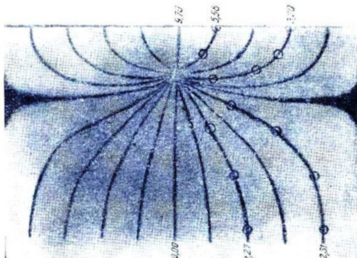
Рис. 90. Линии токов, полученные Хардингом и Будом (1942) в резервуаре с песком, сравниваются с теоретическими линиями тока (обведенные кружками точки), полученными Киркхеном (1945). На рисунке показано просачивание как скопившейся, так и артезианской воды в одну из трубок, находящихся на равном расстоянии друг от друга.
