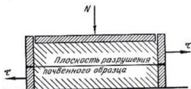
Рис. 12. Действие силы сдвига \tau и сжимающего усилия N . Металлическая коробка, в которой находится образец почвы, заштрихована частой штриховкой.
