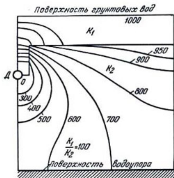
Рис. 86. Эквипотенциали для дренажной трубки в двухслойном подшертом грунте с коэффициентами фильтрации k_1 и k_2 , когда поверхностная почва с k_1 используется для обратной засыпки траншей. Буквой Д обозначена дрена. По Лютину и Гаскеллу (1950).
