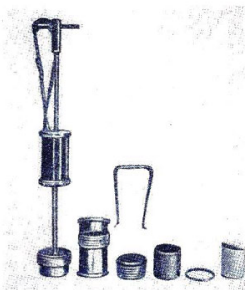
Рис. 181. Оборудование для взятия почвенного моно- лита. По Уланду (1950).
