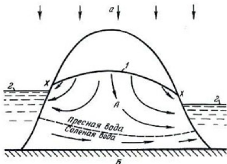
Рис. 29. Поверхность грунтовых вод в условиях устойчивых осадков a , когда пресные грунтовые воды оттесняют соленые грунтовые воды морского происхождения (линза Гиббен-Герцберга):
