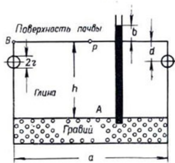
Рис. 88. Изображение ряда дренажных трубок, находящихся в грунте, лежащем на артезианском гравии. Напора воды в гравии достаточно, чтобы поддерживать столб воды в вертикальной трубке (пьезометре) на высоте b над поверхностью почвы.
