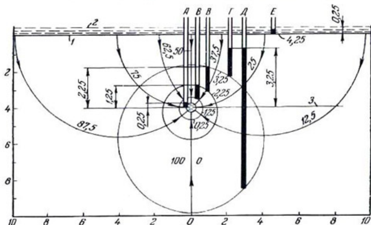
Рис. 77. Эквипотенциали и линии тока, построенные для дренажной трубы, проложенной в грунте, поверх которой находится скопившаяся вода. Грунт простирается неопределенно далеко как в горизонтальном, так и в вертикальном направлениях. Непроницаемый слой находится на большой глубине: 1 — поверхность грунта; 2 — скопившаяся вода; 3 — пьезометр; 4 — уровень отсчета.
