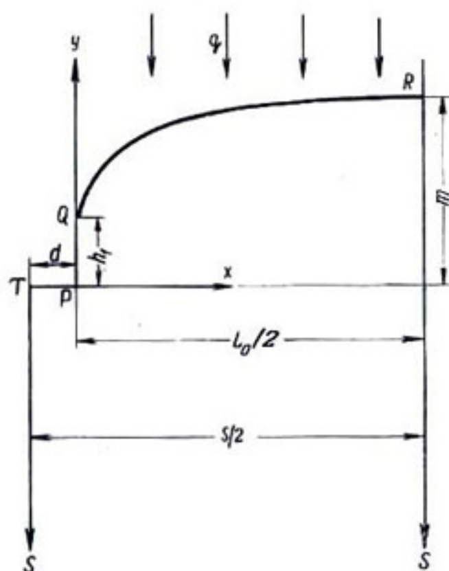
Рис. 124. Установившийся поток к открытым дренам прямоугольного сечения в среде, ограниченной с одной стороны. Непроницаемый слой находится ниже дрен на очень большой глубине или отсутствует совсем. Ширина траншей равна 2d . По ван Демтеру (1950).
