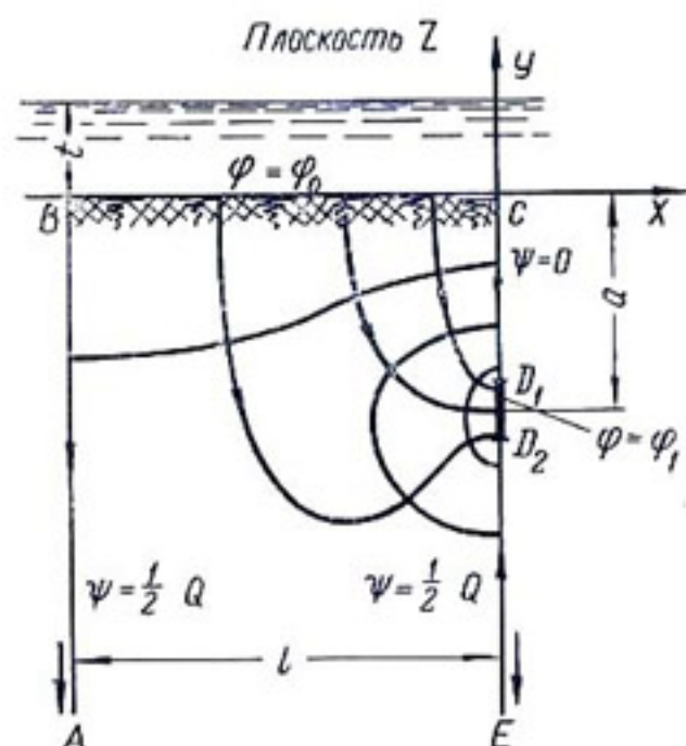
Рис. 129. Поток скопившейся воды к полосовому стоку, вокруг которого вычерчены эквипотенциали, имеющие форму, близкую к эллиптической. По Энгелунду (1951).
