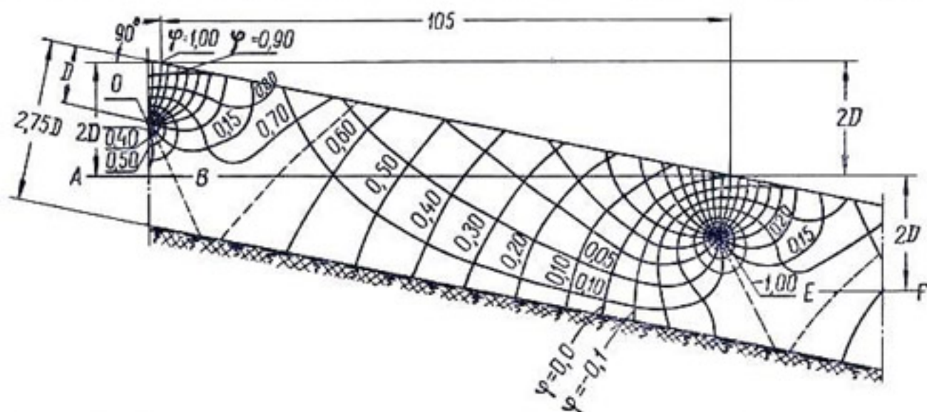
Рис. 94. Гидродинамическая сетка для дренажных труб, находящихся на равных расстояниях друг от друга в водонасыщенном слое почвы, лежащем на водоупоре на склоне холма. По Густафсону (1946).
