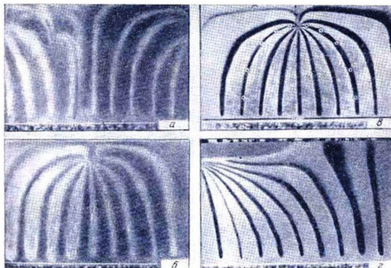
Рис. 89. Испытания на моделях в резервуаре с песком со стеклянной передней стенкой. Линии токов обусловлены артезианским давлением в водоносном пласте (галька ниже песка). По Киркхему (1940а).
