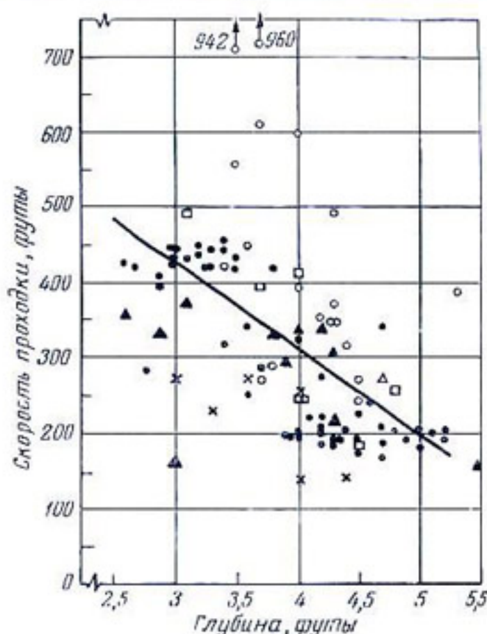
Рис. 142. Зависимость скорости проходки [фут/час] от глубины траншей. По данным Бича (1948), де Фриса (1951), Швэба и др. (1956). Разные обозначения точек на поле графика соответствуют разным машинам.
