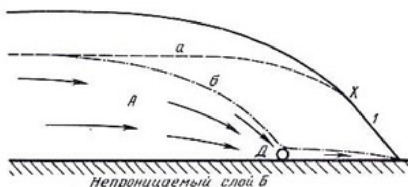
Рис. 28. Поверхность грунтовых вод в случае притока слева, обуславливающего необходимость дренажа у поверхности выклинивания I : a — поверхность грунтовых вод до установки дрены D ; б — поверхность грунтовых вод после установки дрены D .
