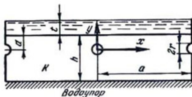
Рис. 78. Ряд труб, расположенных на одинаковом расстоянии друг от друга в грунте со скопившейся водой, который залегает на непроницаемом слое (водоупоре).
