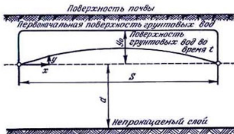
Рис. 38. Схема и обозначения, используемые при выводе уравнения Гловера.
