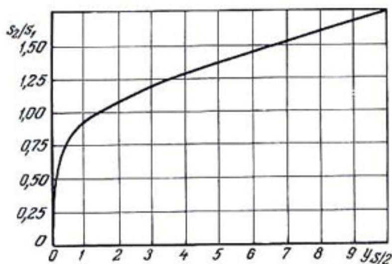
Рис. 39. График изменения отношения расстояний, определенных по двум уравнениям Гловера, в случае расположения дрен на непроницаемом слое и при падении уровня грунтовых вод на один фут (0,3 м).
