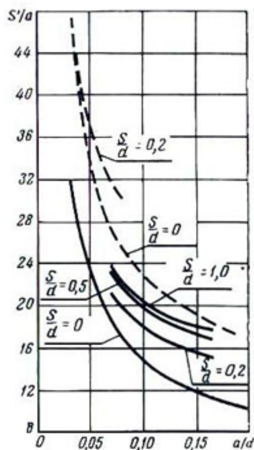
Рис. 191. Графики зависимости расстояния S' от отношения a/d , построенные для различных соотношений s/d (по Киркхему и ван Бейвелу, 1949): пунктирные линии — скважина наполовину заполнена водой ( h=d/2 , t=0 ); сплошные линии — скважина пустая ( h=d , t=0 ).
