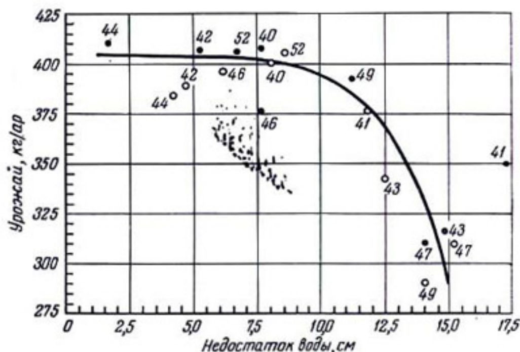
Рис. 208. Зависимость урожая картофеля от недостатка воды. По ван Дуину и Шолте Убингу (1955). Цифры около точек указывают годы опыта (1941—1952). Недостаток влаги определяется как разность между величиной P , E и количеством доступной влаги.
