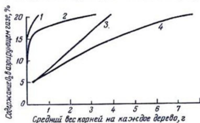
Рис. 225. Зависимость среднего веса корней растений, выращенных на питательном растворе, от содержания кислорода в аэрирующем газе.
