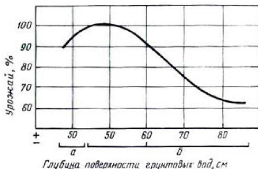
Рис. 235. Урожай гнацинта Невишность в зависимости от уровня грунтовых вод. По Блаву (1938b): а — мелкий дюнный песок; б — крупный дюнный песок.
