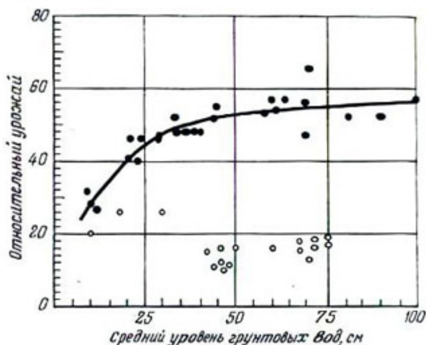
Рис. 218. Зависимость между урожаем пастбищной травы на песчаной почве и средней глубиной поверхности грунтовых вод. Светлые точки соответствуют участкам, которые зимой затапливались. Урожай с этих участков заметно ниже урожая с участков, где уровень грунтовых вод постоянно находился ниже поверхности почвы (черные точки).
