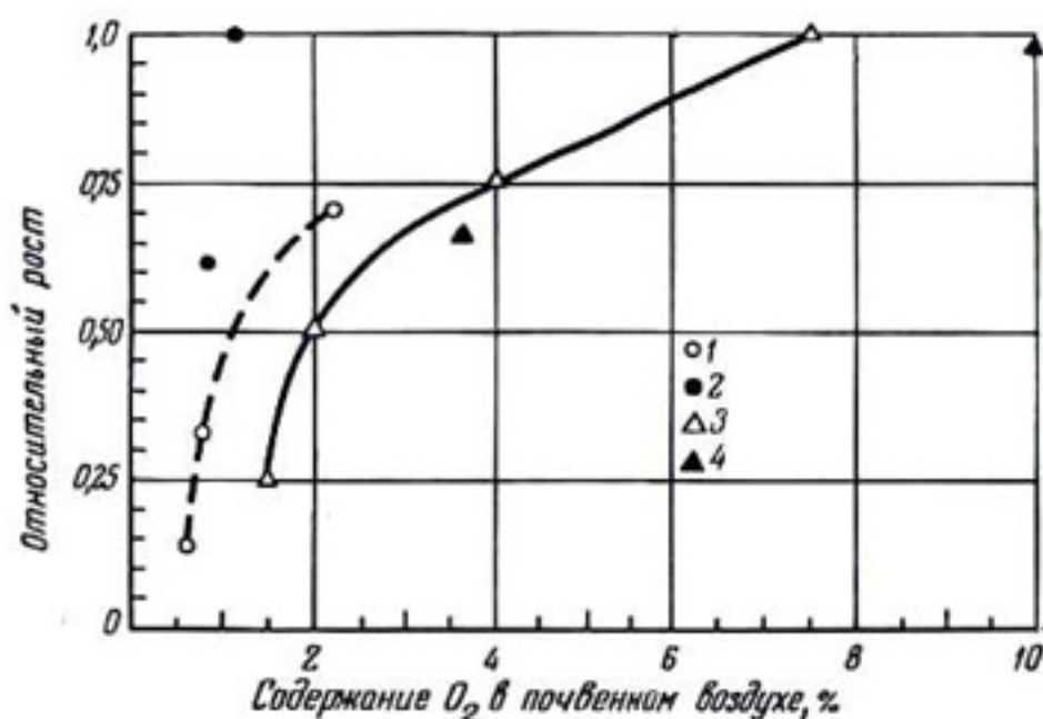
Рис. 204. Зависимость скорости роста различных видов растений от парциального давления кислорода при постоянной температуре. По Кэннону (1925): 1— Prosopis velutina , 20°; 2— Citrus sinensis , 27°; 3— Gossypium barbadense ; 4— Zea mays , 17°.
