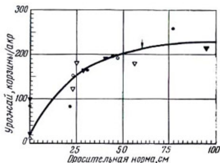
Рис. 212. Урожай сортов сахарной кукурузы Орегон Евергрин ( \nabla ) и Золотой Бен-там ( \circ ) в 1940 г. (светлые значки) и в 1941 г. (темные значки) в зависимости от количества оросительной воды. По Ричардсу и Уодлею (1952). Если принять, что эффективность орошения составляет 50%, то стрелка указывает «полезное водопотребление» (Блайни и Кридл, 1950).
