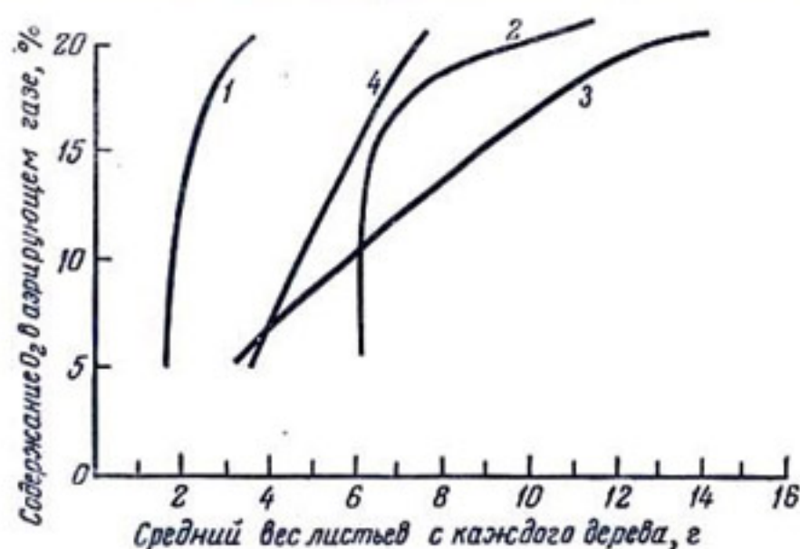
Рис. 226. Зависимость среднего веса листьев с растений, выращенных на питательном растворе, от содержания кислорода в аэрирующем газе:
