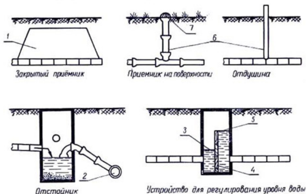
Рис. 141. Специальные устройства для гончарных дренах:
