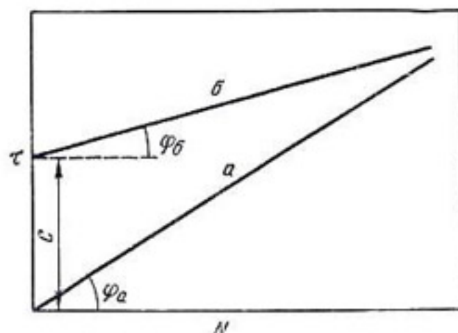
Рис. 13. Зависимость силы сдвига от нормальной нагрузки:
