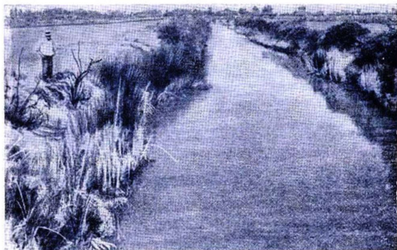
Рис. 164. Коллектор для отвода больших количеств поверхностной и подпочвенной дренажной воды.
