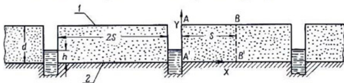
Рис. 92. Чертеж к задаче просачивания воды из водонасыщенной почвы в канавы, расположенные на одинаковом расстоянии друг от друга и врезающиеся в непроницаемый слой. По Киркхему (1950b): 1 — поверхность почвы; 2 — поверхность водоупора.
