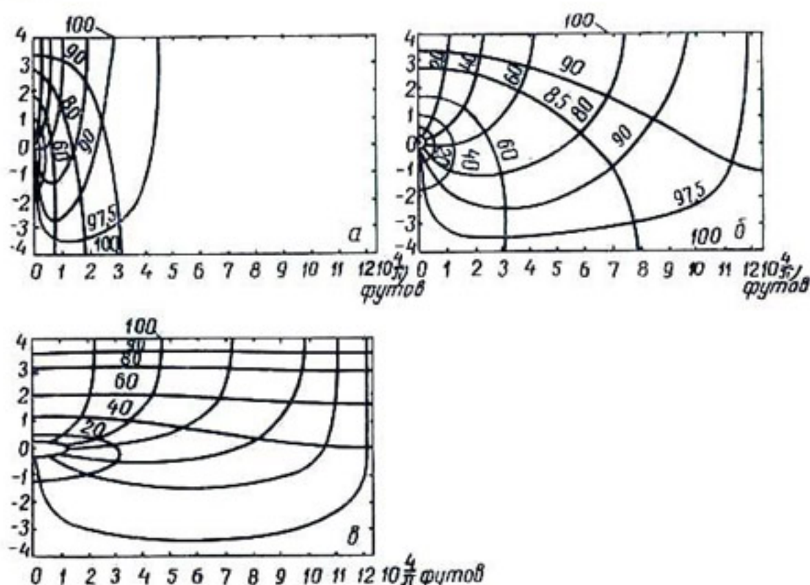
Рис. 127. Линии токов и эквипотенциали в анизотропном грунте, построенные для потока скопившейся воды в дренах эллиптической формы. Расстояние между дренами составляет 20 ( 4/\pi ) футов (7,75 м). Непроницаемый слой находится в 8 футах (2,44 м), а центр голицарной дрены — в 4 футах (1,22 м) от поверхности почвы. Для графиков а, б и в отношение (k_h/k_v)^{1/2} = 1/4 , 1 и 4 соответственно.
