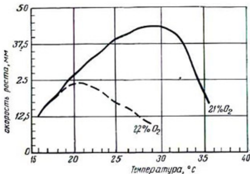
Рис. 203. Зависимость скорости роста корней хлопчатника от температуры (Кэннон, 1925).
