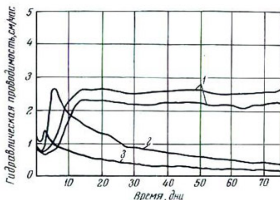
Рис. 180. Влияние микроорганизмов на гидравлическую проводимость суглинка при продолжительном затоплении. По Аллисону (1947):
