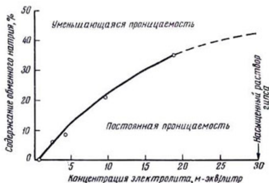
Рис. 178. Концентрация электролитов в пригационной воде, требующаяся для сохранения постоянной почвенной проницаемости при различной степени насыщения обменным натрием. По Квирку и Скофилду (1955).
