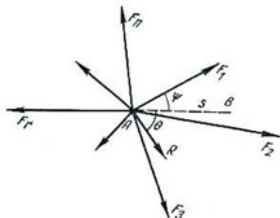
Рис. 16. Изображение сил, поясняющее обусловленный ими потенциал.
