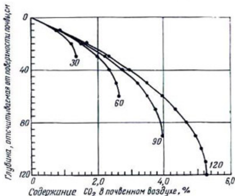
Рис. 207. Максимальное процентное содержание \text{CO}_2 на различных глубинах, подсчитанное по формуле p = p_0 - \alpha H(-Lz + z^2/2)^2 . По ван Бейвелу (1951).
