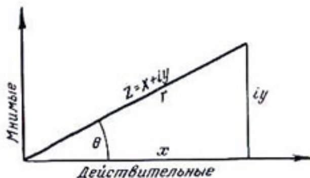
Рис. 75. Представление комплексного числа z .
