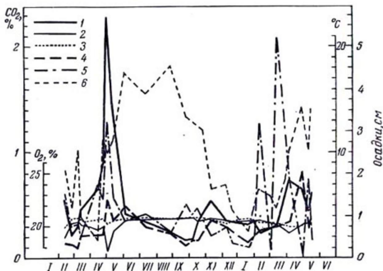
Рис. 205. Изменение содержания CO_2 и O_2 в течение года на глубине 15 см на участках, которые были засеяны пшеницей. По Расселу и Апплейярду (1913):
