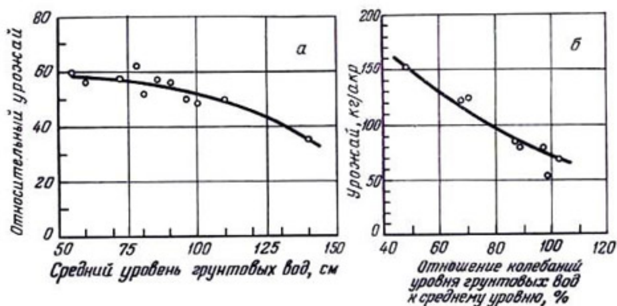
Рис. 217. Зависимость урожая земляники (кг/агр), полученного на песчаной почве, от положения поверхности грунтовых вод (по Виссеру, 1948):
