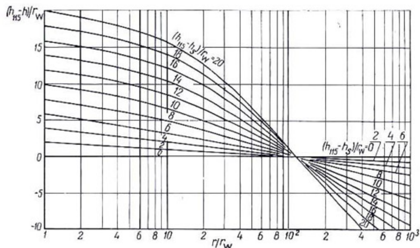
Рис. 100. Обобщенные кривые профиля свободной поверхности для колодцев в непiezометрическом бассейне грунтовых вод.
