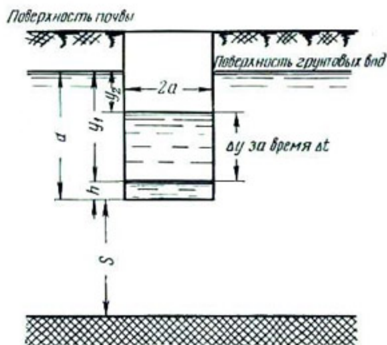
Рис. 157. Скважина в однородном грунте, используемая при определении водопроницаемости.
