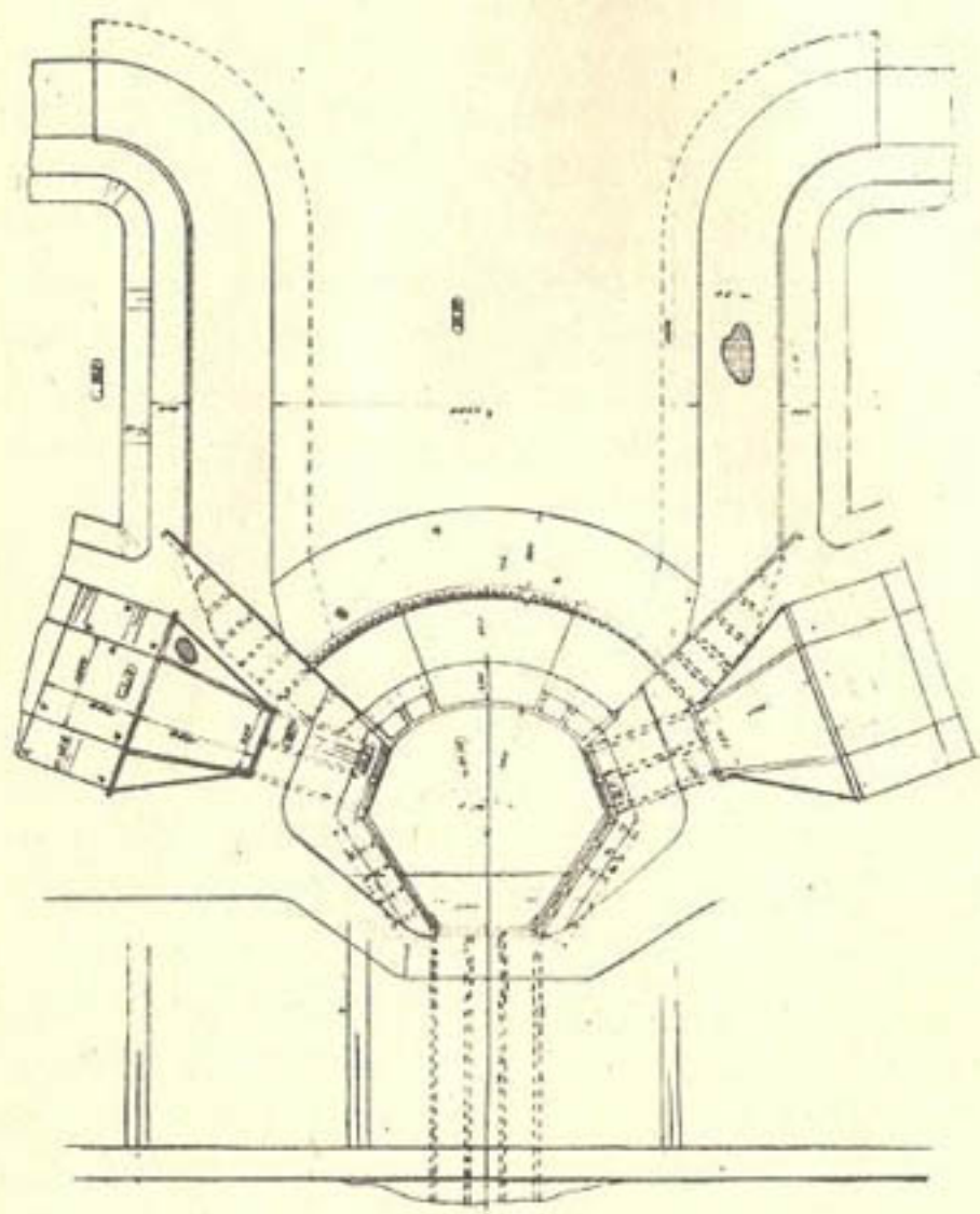
Рис. I. План концевой части Чимкурганского гидроэлектрического сброса и принятого к исследованию варианта
