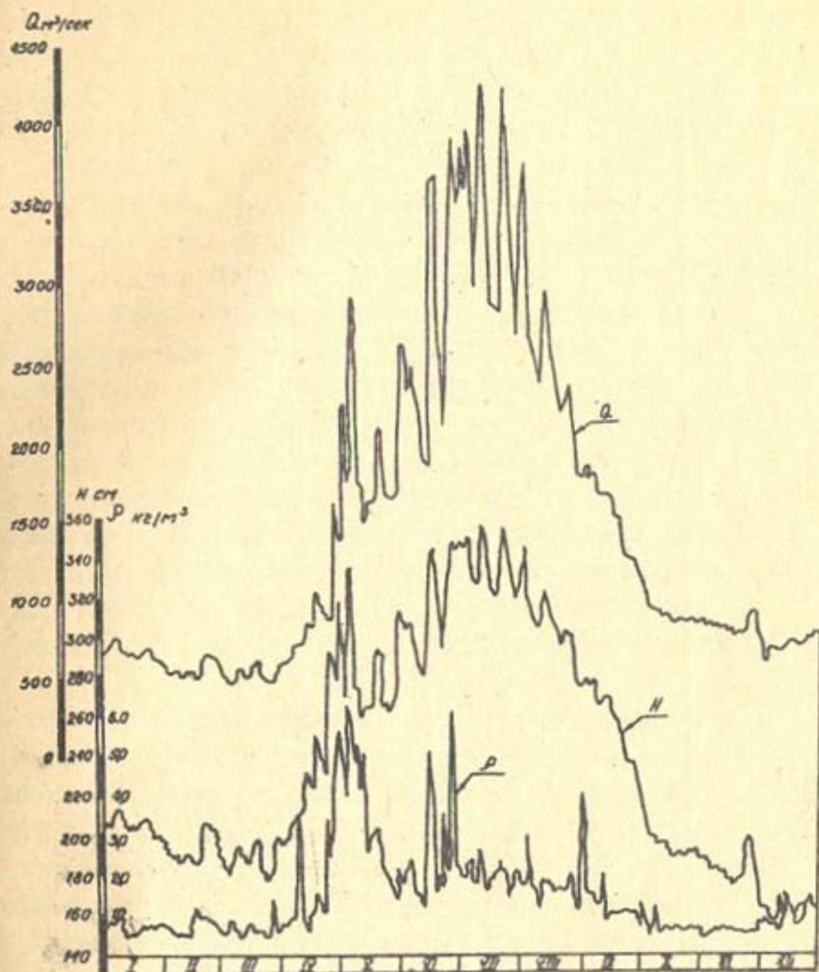
Рис. I График колебания расхода и горизонта воды р.
