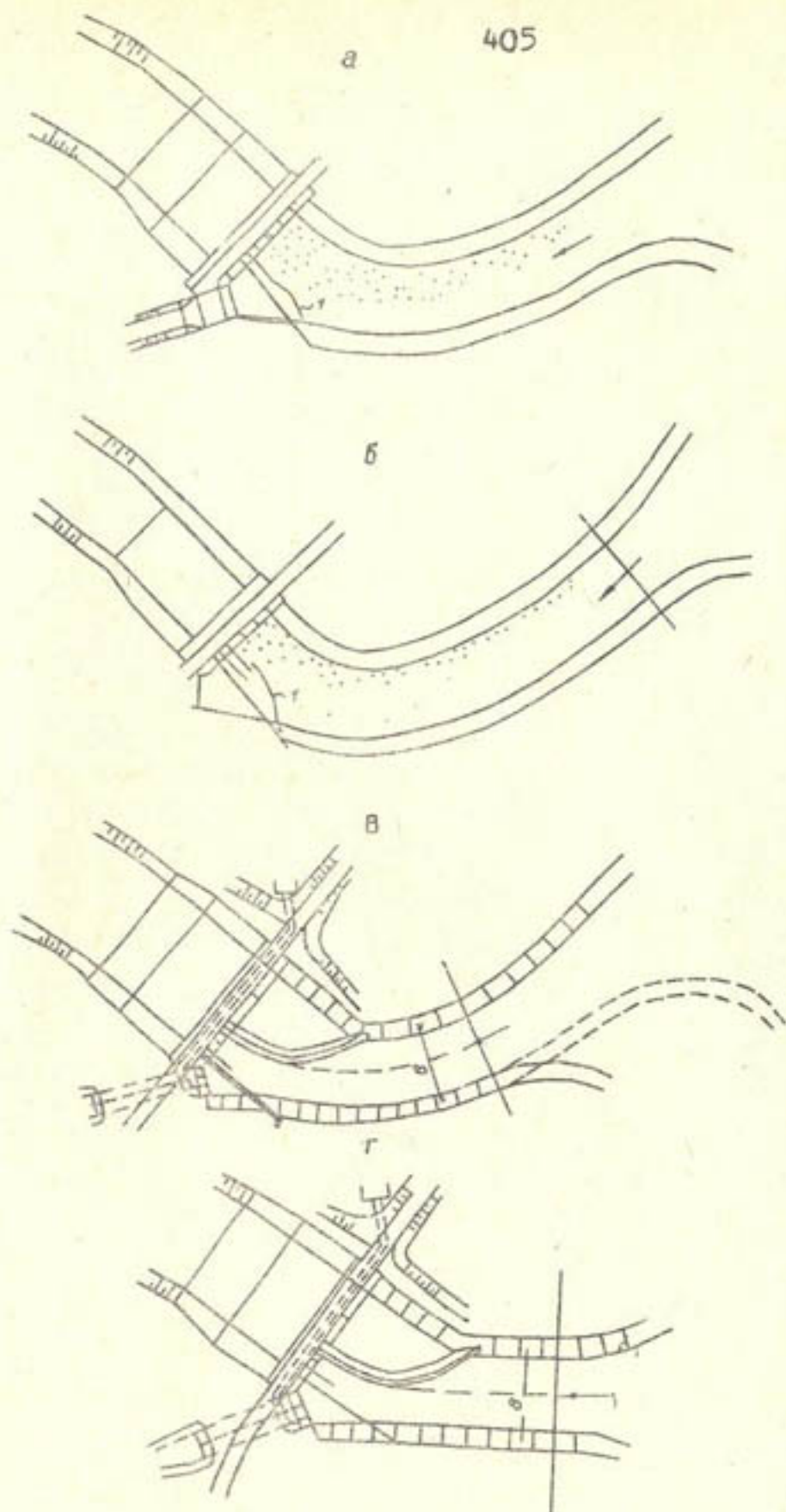
Рис. 2. Возможные схемы водозабора с открытой поперечной галереей: а) одиночная галерея; б) двойная галерея; в) при наличии катастрофического водослива с криволинейным подводящим руслом; г) при наличии катастрофического водослива с прямолинейным подводящим руслом; Г-линия гряды наносных отложений.
