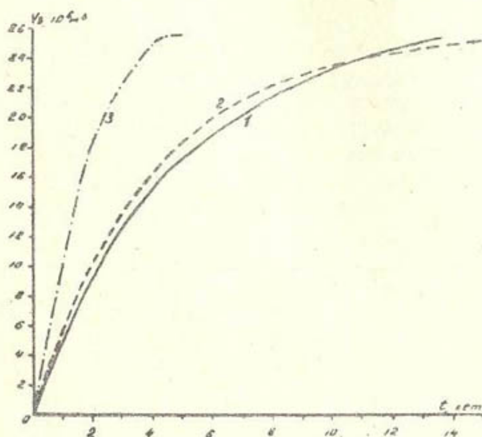
Рис. 3 Объемы заполнения верхнего бьефа на р. Нарын: 1—расчет по уравнению (5); 2—расчет по методу В.С.Лапшенкова; 3—то же И.А.Шне- ера.
