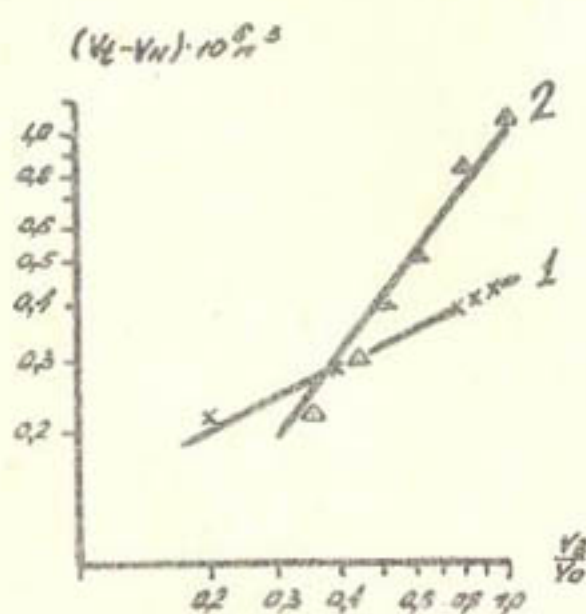
Рис. 5. График зависимости V_t - V_H = f\left(\frac{V_2}{V_0}\right) по натурным данным: 1— кампырраватский бьеф, 2— газалкентский.
