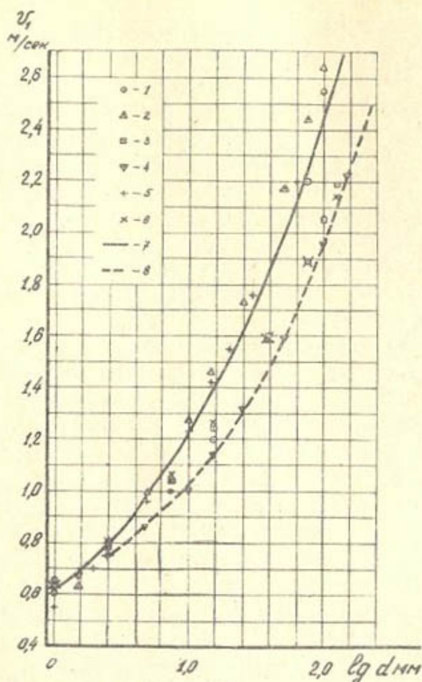
Рис. I. Зависимости размывающей и несдвигающей скоростей от крупности зерен грунтов русла при глубине 1 м: 1- по А.А.Черкасову; 2- В.Н.Гончарову; 3- Г.С.Чекулаеву; 4- В.Н.Гончарову; 5- Ц.Е.Мирцхулаве; 6- Б.И.Студеничкинову; 7- по формуле (Б); 8- огибающая несдвигающих скоростей.
