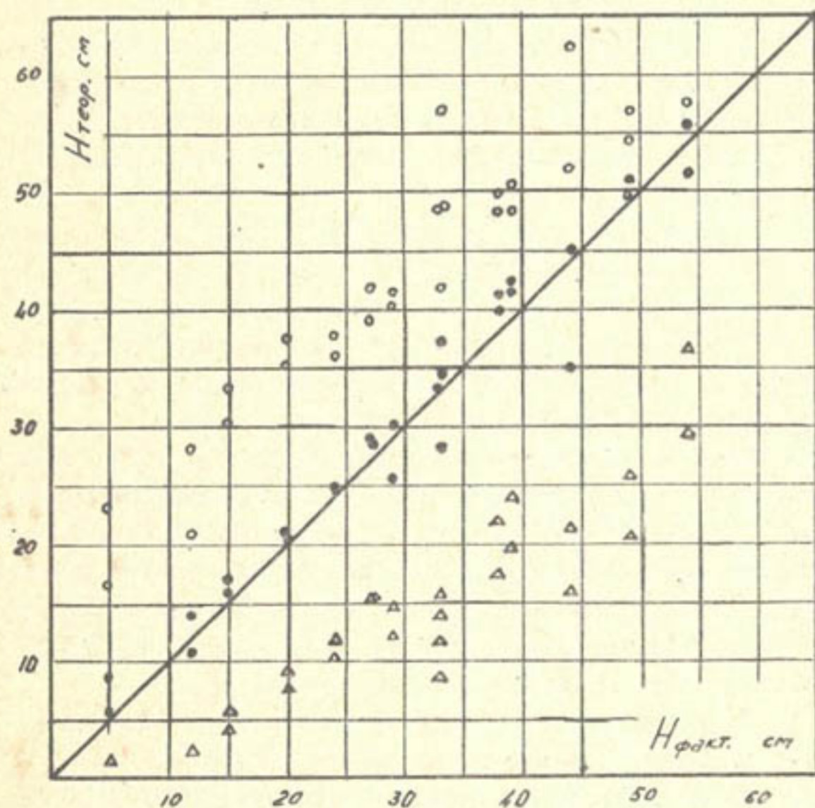
Рис. I Сопоставление прогнозируемой и фактической глубины размыва:
