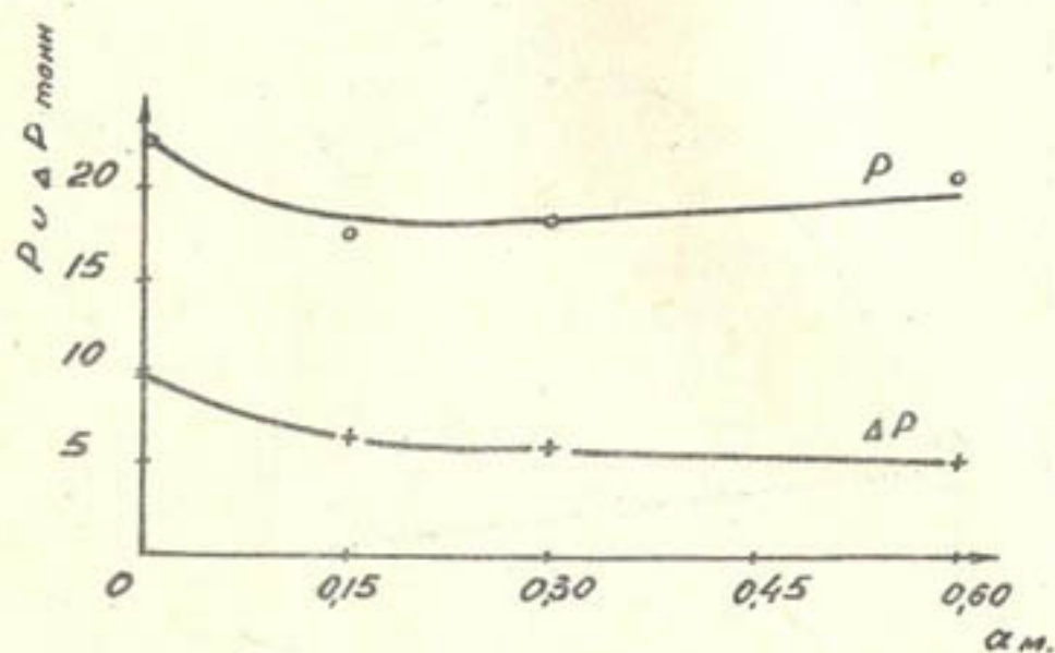
Рис.3 График зависимости \bar{P} и \bar{\Delta P} от ширины щели между плитой пола и концевой плитой сброса.
