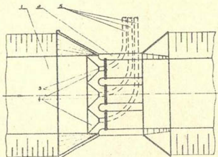
Рис. I Наносоуловитель для каналов: 1-канал; 2-наносоуловитель; 3-наносоулавливающее отверстие; 4-входная воронка; 5-галерея.
