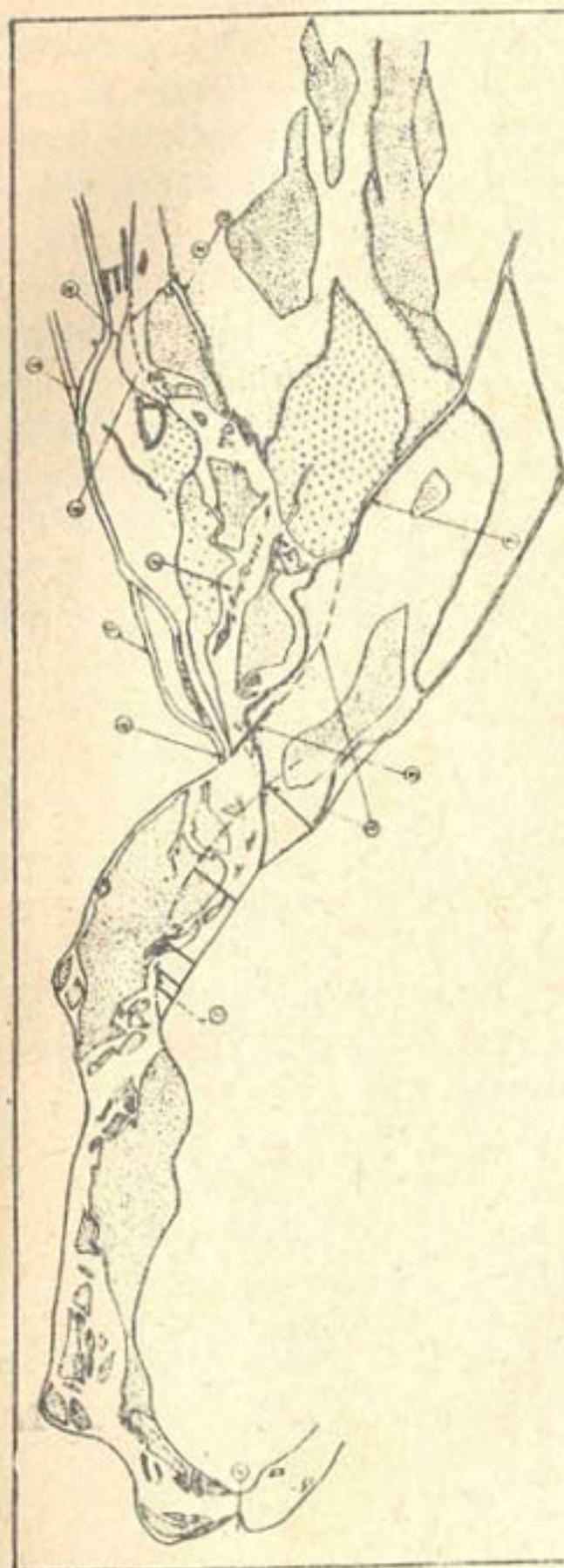
Рис. 4. План участка р. Амударья в районе Ташсака по материалам аэрофотоъемки 17-18 декабря 1961 г. при Q = 660 \text{ м}^3/\text{сек}
