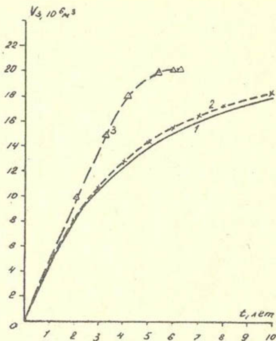
Рис.2 Объемы отложений второй стадии заиления Султанбентского водохранилища: 1-расчет по уравнению (5); 2-расчет по методу В.С.Лапшенкова; 3-то же И.А. Шнеера.
