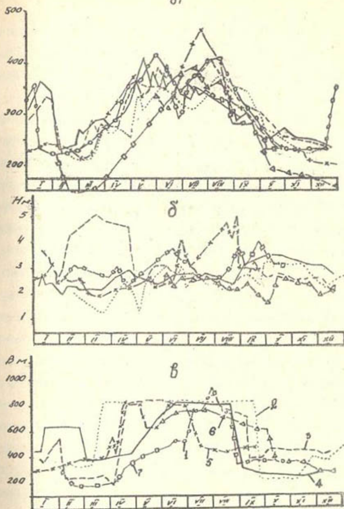
Рис.3. Графики изменения уровня воды (а), глубины потока (б) и ширины потока (в): 1-1938 г.; 2-1955; 3-1956; 4-1957; 5-1958; 6-1962; 7-1967 г.
