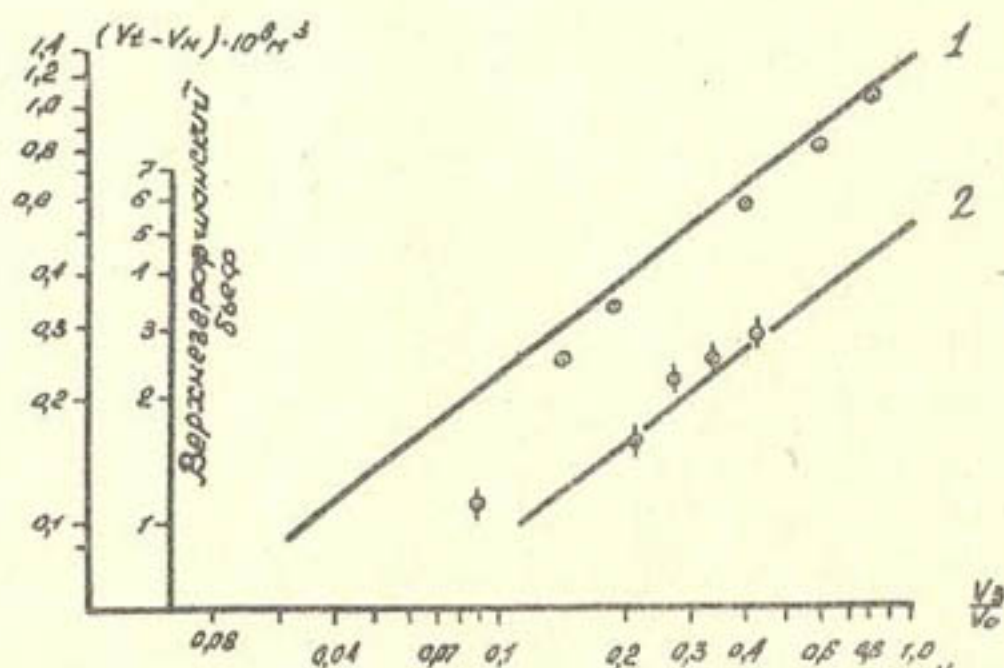
Рис. 4. График зависимости V_L - V_H = f\left(\frac{V_3}{V_0}\right) по натурным данным:
