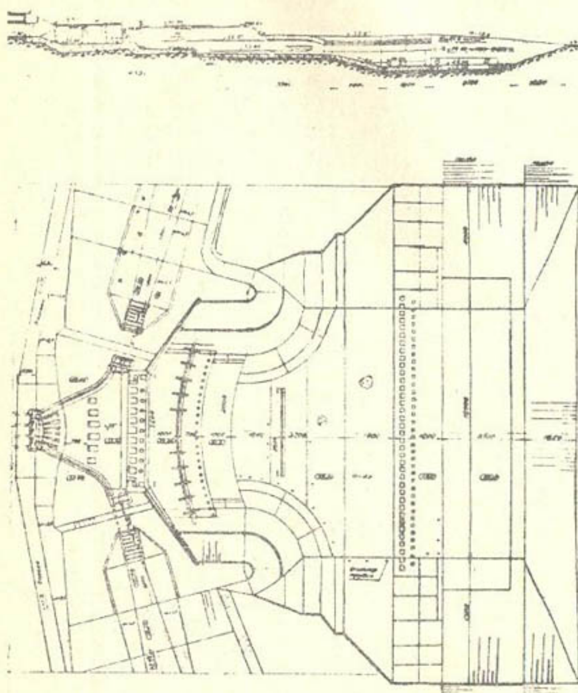
Рис. 5. План и продольный разрез реконструкции катастрофического сброса Чимкурганского водохранилища (после снижения русла НБ на расчетную величину - 2,5 м)
