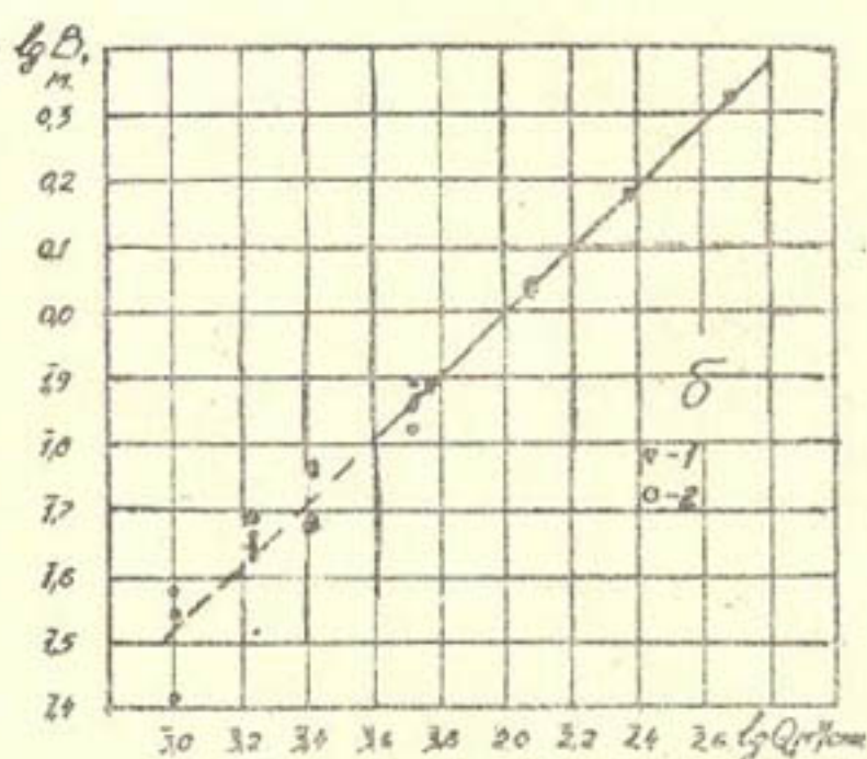
Рис. I Зависимость средней глубины (а) и ширины потока (б) от расходов воды: 1-опыты с сырдарьинским песком; 2-опыты с песком из жженого кирпича.
