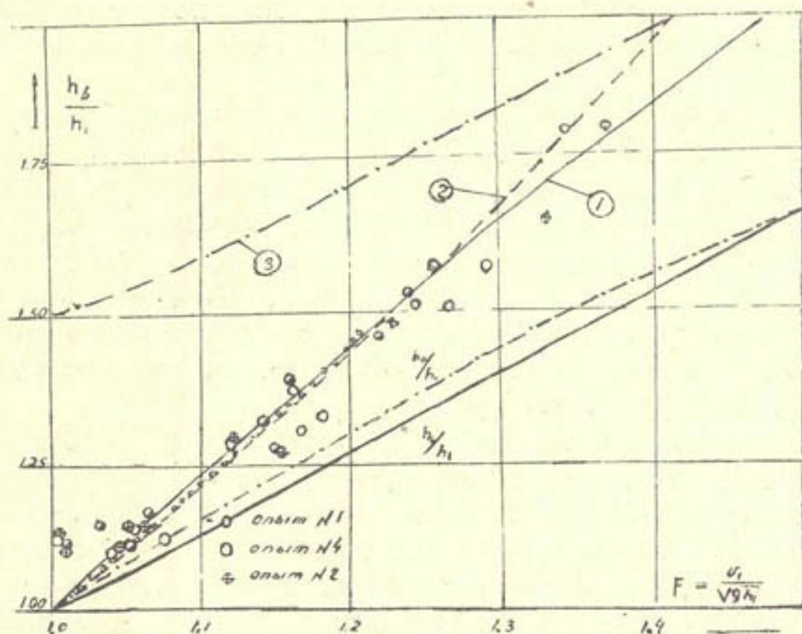
Рис. 7. Сравнение предлагаемых формул для h_\delta с опытными данными К.Тиррио и С.Беднарчика. Расчетные точки Р.Лемузна; 1- по предлагаемой формуле (19); 2- по формуле (2); 3- величина удельной энергии \mathcal{E}_1(h) .
