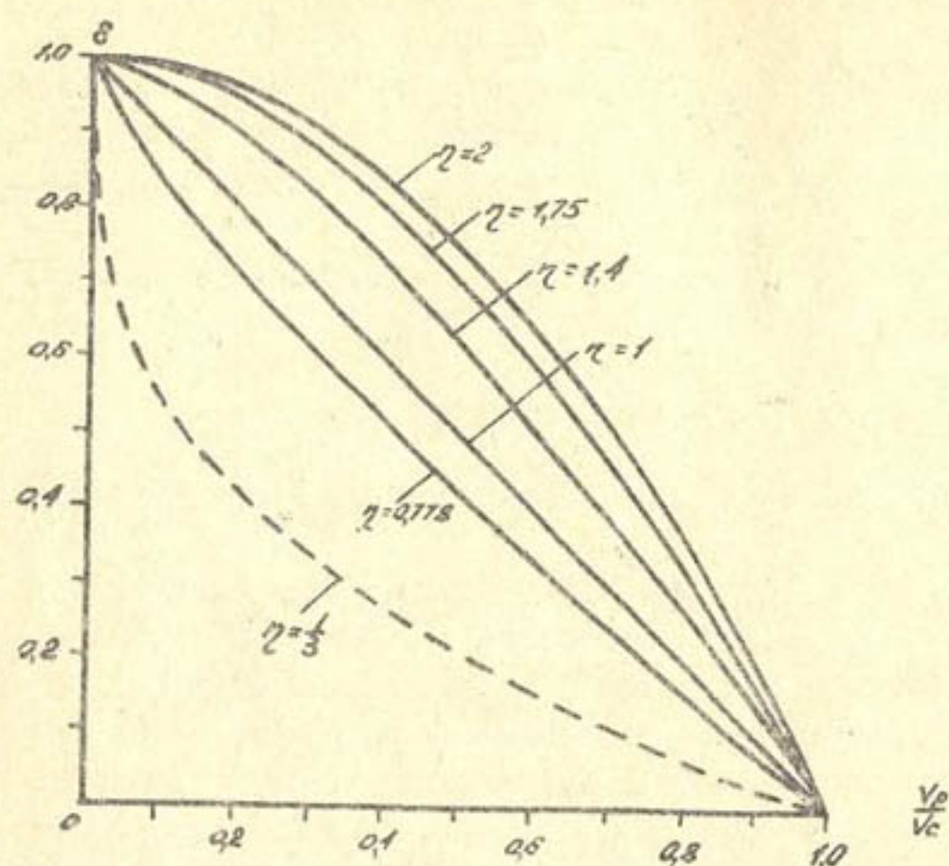
Рис. I. Расчетный график [по ур-нию (9)] изменения степени освещения \varepsilon верхних бьефов низконапорных гидроузлов от отношения \frac{v_p}{v_c} .
