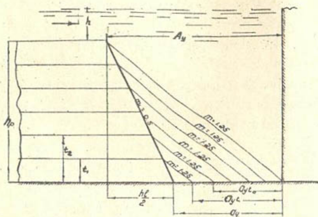
Рис. 4. Схема для расчета параметров безнаносной зоны при различной толщине слоя донных отложений
