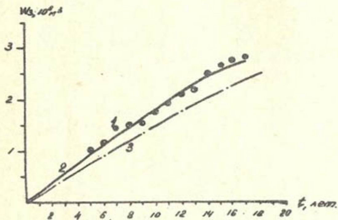
Рис. 4 Объемы заиления водохранилища Заалах (Бавария): 1—натурные данные; 2—расчет по предлагаемому методу; 3—то же по методу И.А. Шнедера.
