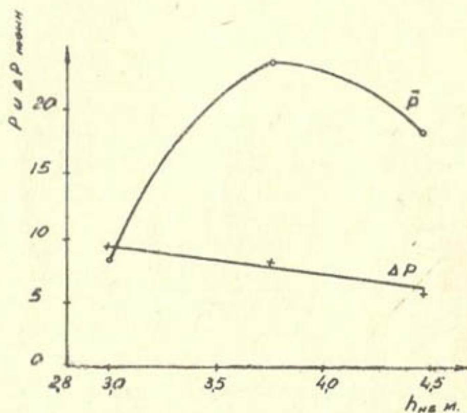
Рис.2 График зависимости осредненной \bar{P} и пульсационной \bar{P} составляющих гидродинамической нагрузки потока на плиту уральского пола от глубины нижнего бьефа
