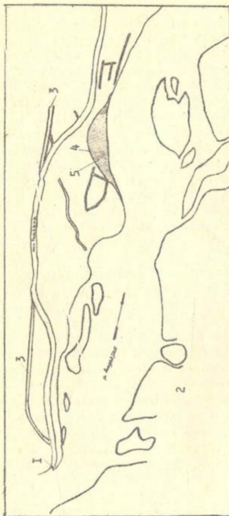
Рис. 3 План р. Амударьи ниже головного сооружения к Ташсака по аэрофотосъемке 1961г.:
