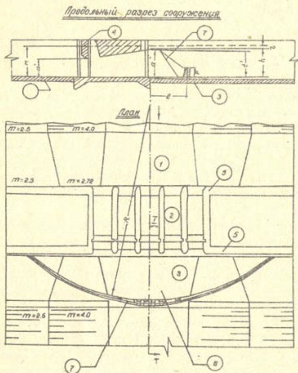
Рис. I. Подпорное сооружение с растекателем-криволинейной стенкой: 1-понур; 2-щитовая часть; 3-слив; 4-диафрагма; 5-обратные стенки; 6-донная плита слива; 7-криволинейная стенка-растекатель
