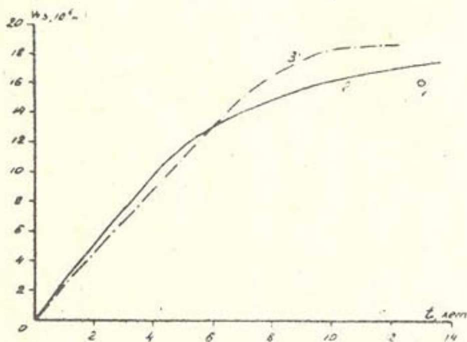
Рис.5 Объемы заиления водохранилища Байсен (С Ш А): 1-натурные данные; 2-расчет по предлагаемому методу; 3-то же по методу И.А.Шнеера .
