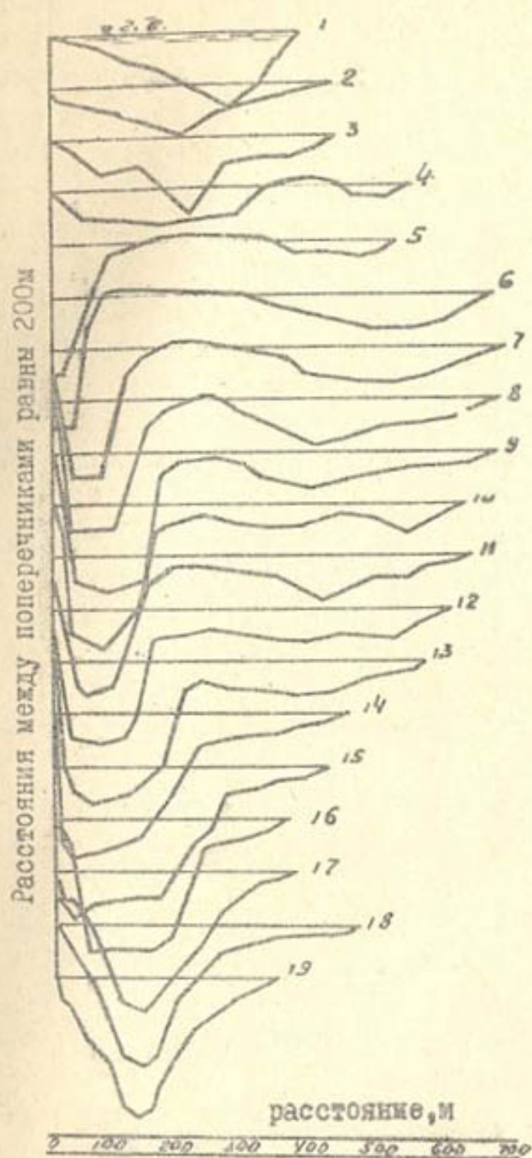
Рис. 7 Поперечные профили русла реки Амударьи на участке дейгиша в р-не к-ла Ташсака на 10 октября 1961г. (сверху вниз по течению).
