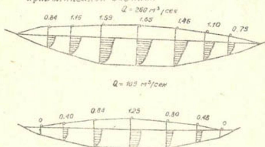
Рис. 3. Эпюры распределения скоростей (створ № 3).
