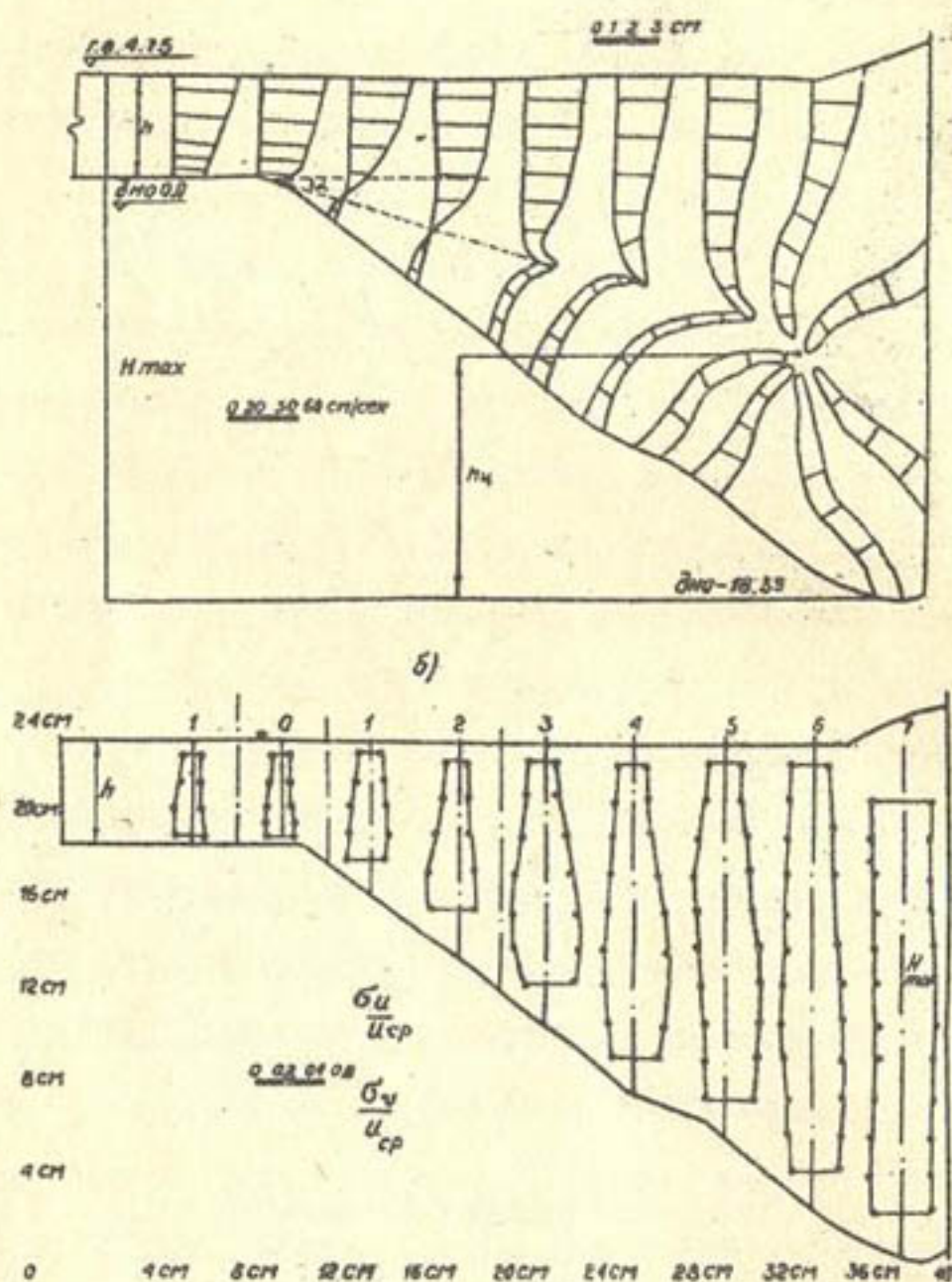
Рис. I. Распределение осредненных (а) и пульсационных (б) скоростей в под-ходном русле и воронке размыва при Fr = 0,38
