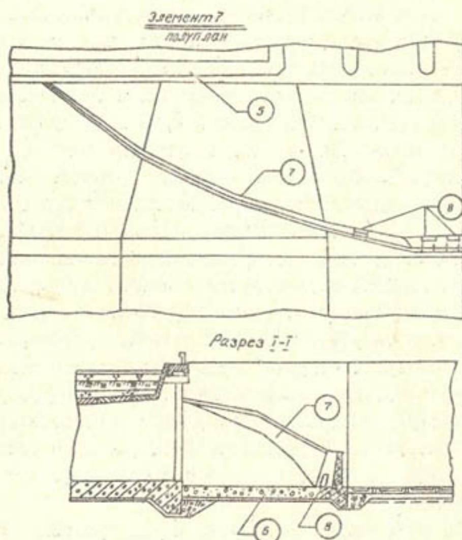
Рис.2. Растекатель в плане и в разрезе: 5-обратные стенки; 6-донная плита слива; 7-криволинейная стенка-рас- текатель; 8-донные отверстия.
