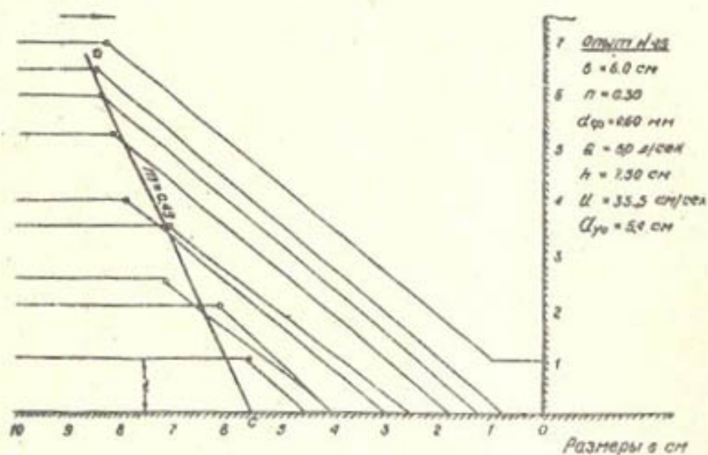
Рис.3. Картина донных отложений перед бычком
