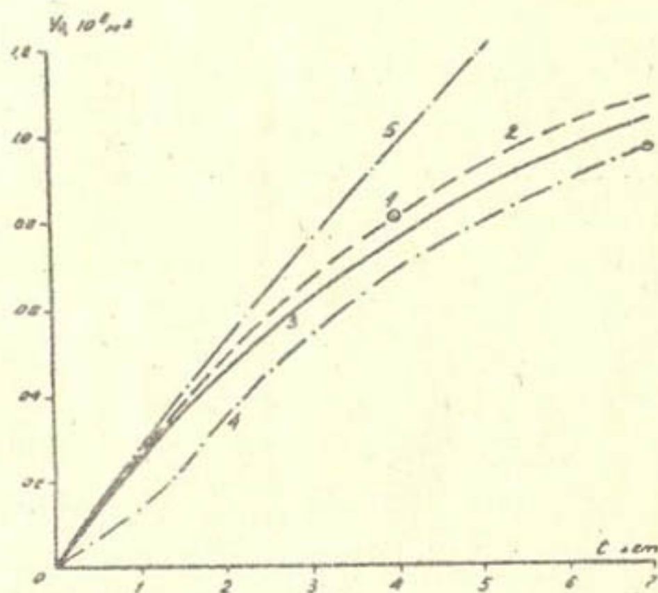
Рис.6 Объемы заплнения Бозсуйского бьефа: 1—натурные данные; 2—расчет по методу В.С.Лашенкова; 3—то же по уравнению (5); 4—по вычислениям И.А.Шнеера (при W_p = 0,549 \cdot 10^6 \text{ м}^3 ); 5—по уравнению (2) при W_p = 0,2 \cdot 10^6 \text{ м}^3 .
