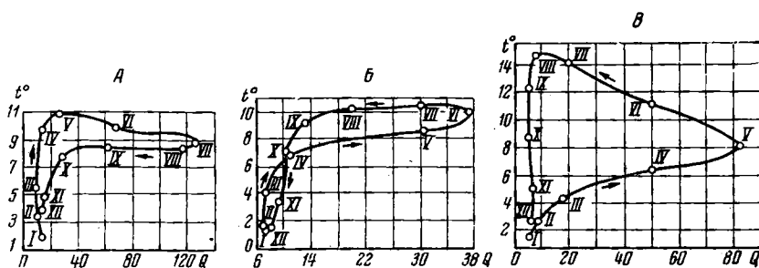
Рис. 49. Зависимость средних месячных температур воды от их расхода
