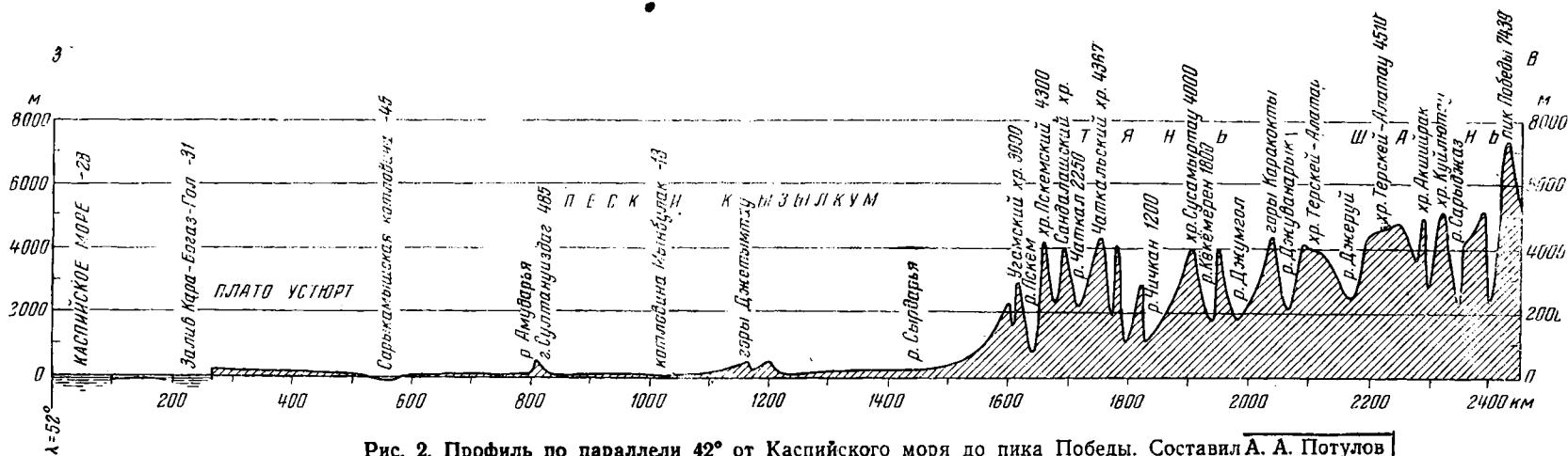
Рис. 2. Профиль по параллели 42^\circ от Каспийского моря до пика Победы. Составил А. А. Потулов
