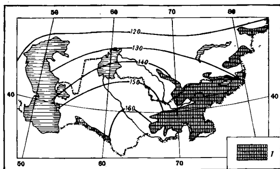
Рис. 17. Суммарная солнечная радиация за год, \text{ккал/см}^2\text{год}
