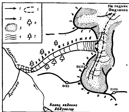
Рис. 37. План ледника Медвежьего
