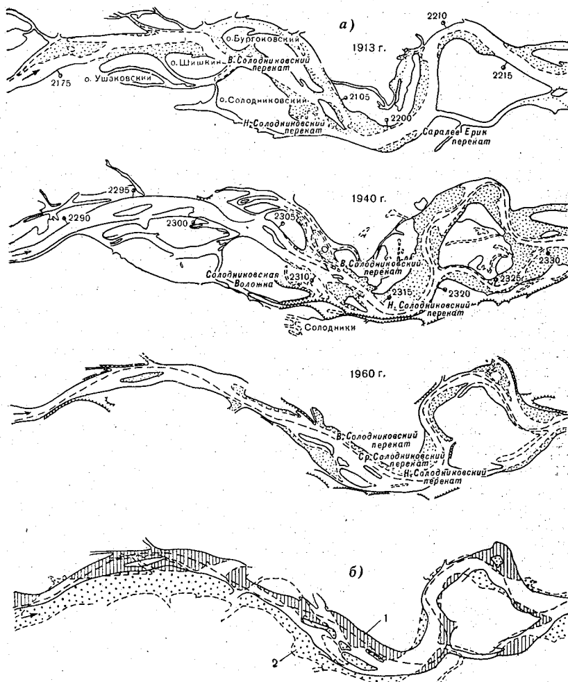
Рис. 73. Сопоставленные планы (а) и схема общих плановых деформаций берегов русла (б) на участке Солонниковских перекатов за период 1913—1940 гг.
