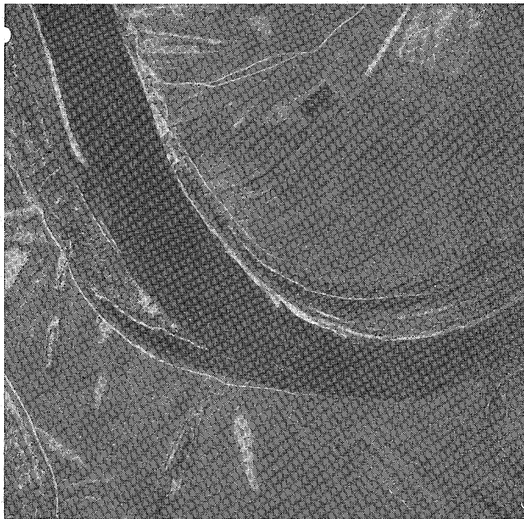
Рис. 23. Затоны, образовавшиеся в ходе свободного меандрирования.
