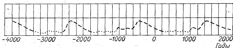
Рис. 1. Приближенные многовековые циклы колебаний увлажненности Евразии и Северной Америки (по А. В. Шнитникову).
