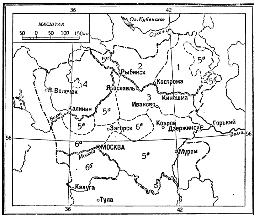
2. Схема расположения почвенных районов.
