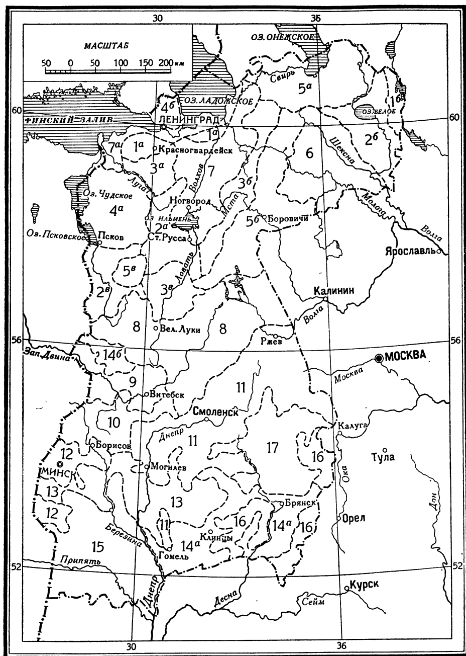
Схема расположения почвенных районов.
