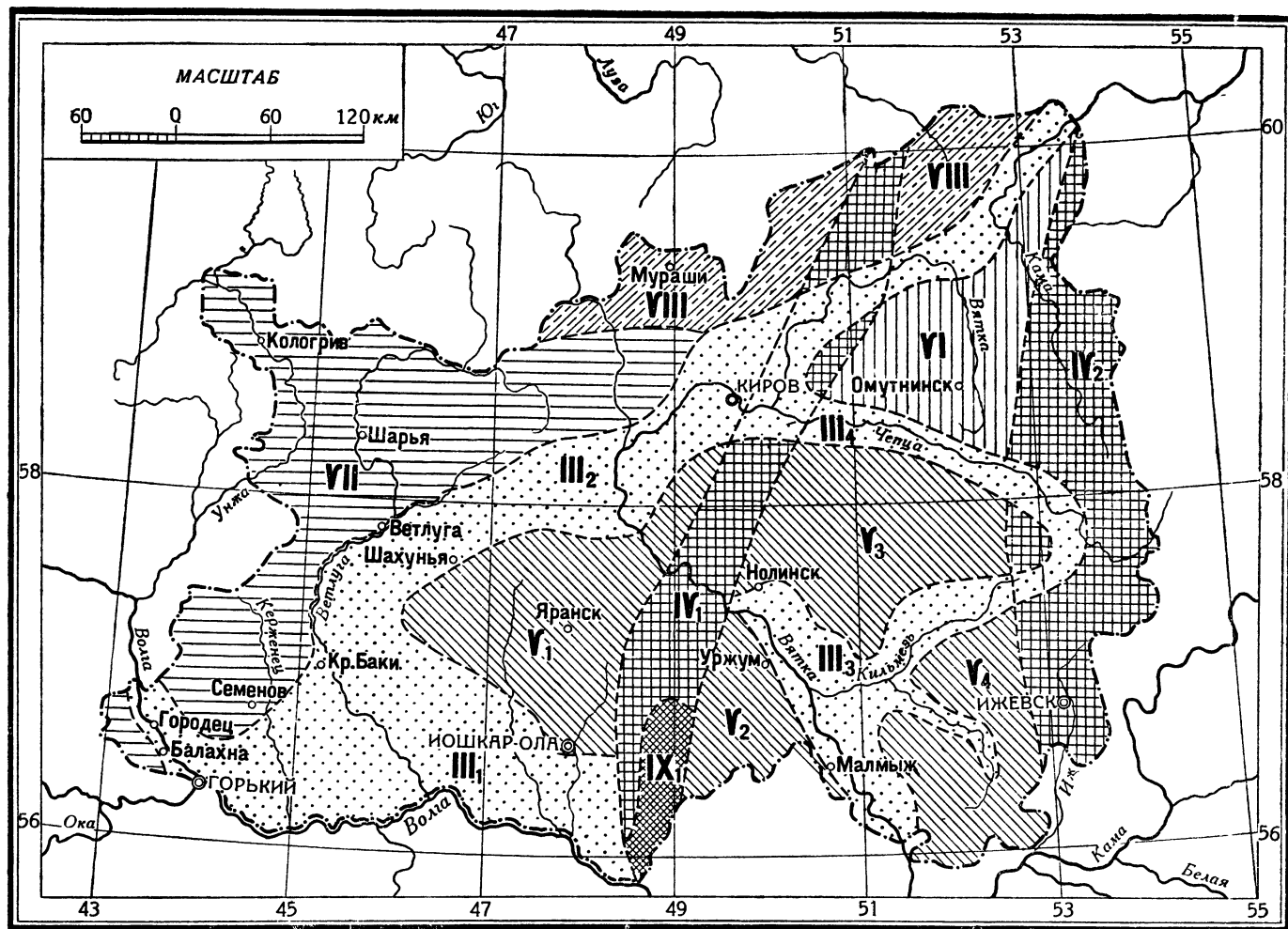
Геоморфологическая карта Кировской и Горьковской областей (по Добрынину).
