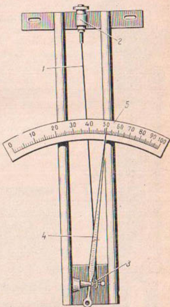
Рис. 6. Волосной гигрометр.
