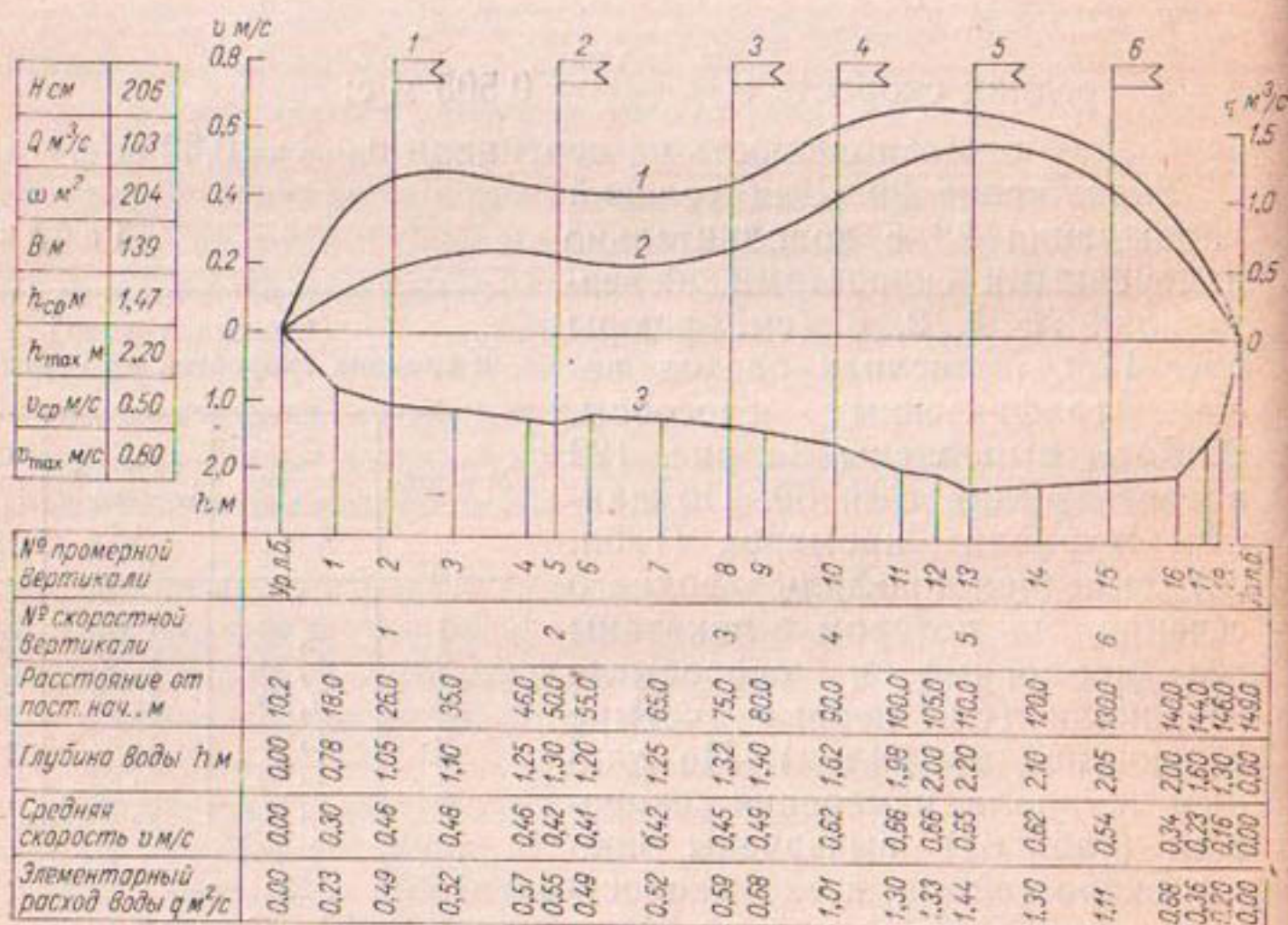
Рис. 122. Вычисление расхода
