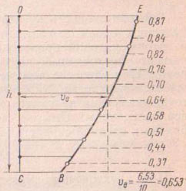
Рис. 112. Эпюра скоростей на вертикали.
