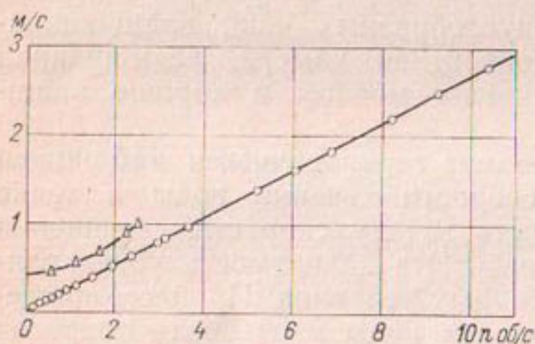
Рис. 120. Тарифовочные кривые.
