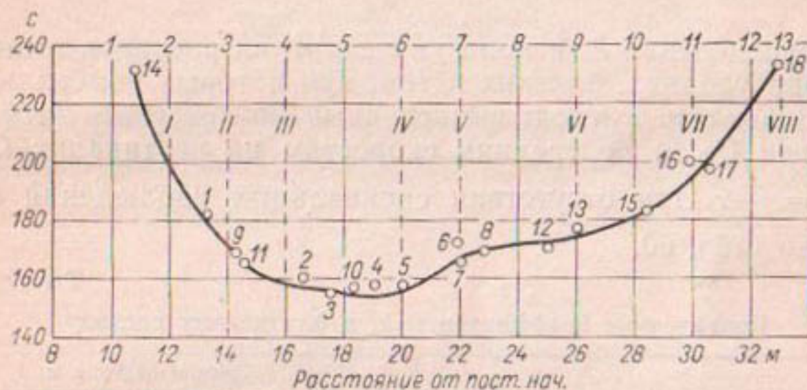
Рис. 116. Эпюра распределения продолжительности хода поплавков по ширине русла.
