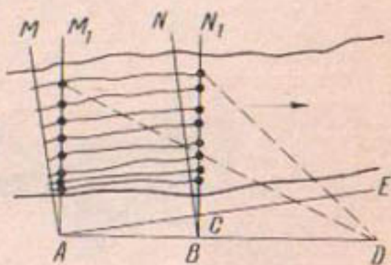
Рис. 89. Определение направления гидрометрического створа.
