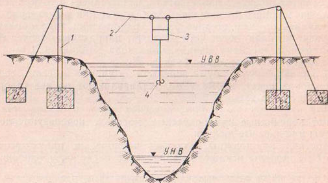
Рис. 92. Подвесная люлька. 1 — стойка; 2 — перекидной трос; 3 — люлька; 4 — вертушка.
