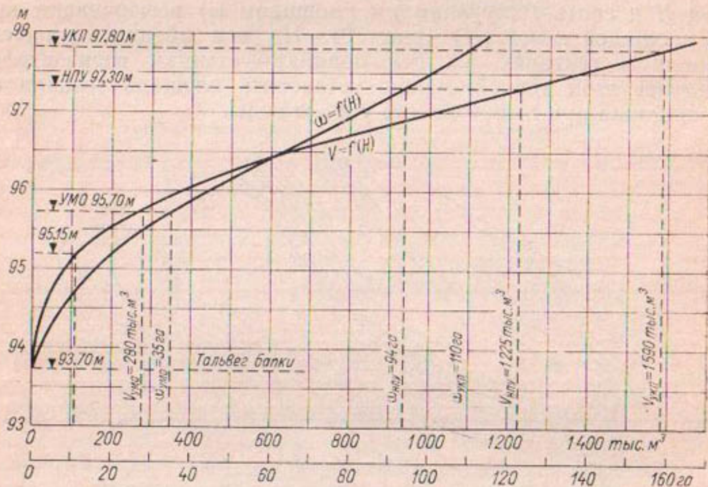
Рис. 79. Кривые площадей и объемов водохранилища на р. Сухая Маячка.
