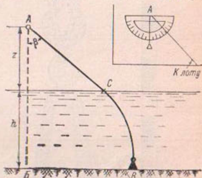
Рис. 104. Относ лота.
