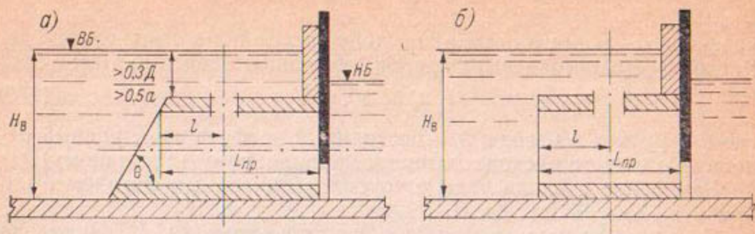
Рис. 147. Водомерная приставка. а — наклонный вход в приставку, б — прямой вход.
