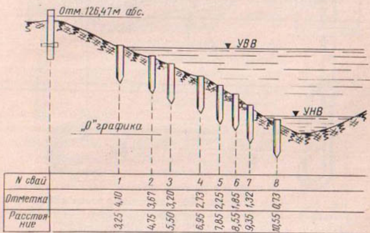
Рис. 83. Свайный водомерный пост (расстояния даны от репера водомерного поста). Отметки — над нулем графика.
