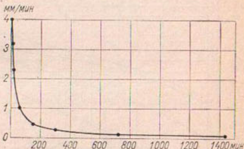
Рис. 17. Кривая зависимости средней интенсивности дождя (повторяемостью 1 раз в 100 лет) от его продолжительности для района г. Свердловска.
