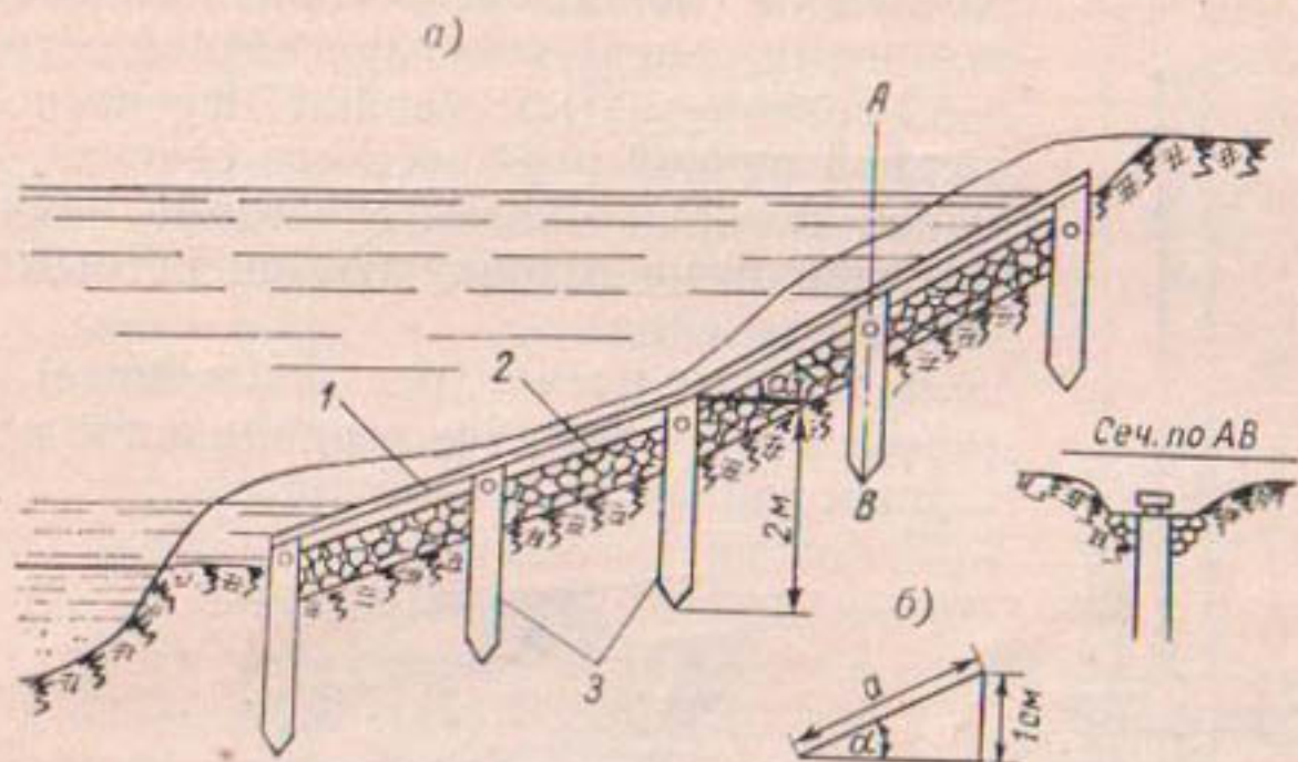
Рис. 82. а — схема установки наклонной рейки. 1 — наклонная рейка, 2 — щебенчатая подготовка, 3 — сваи. б — расчет делений наклонной рейки.
