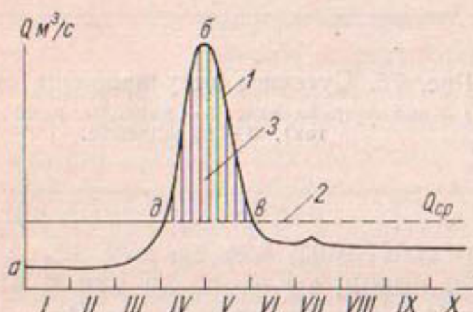
Рис. 77. Сезонно-годовое регулирование стока.
