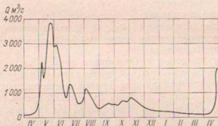
Рис. 44. График колебания расходов воды (гидрограф) р. Вычегды у г. Сыктывкара.
