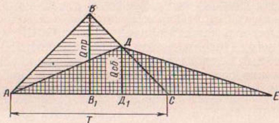
Рис. 65. Схема трансформации паводка при треугольной форме гидрографа.
