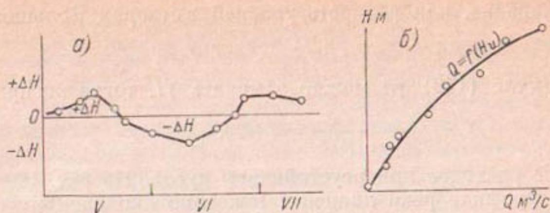
Рис. 130. Внесение поправок к уровням воды в случае неустойчивого русла. а — хронологический график поправок; б — кривая расходов.
