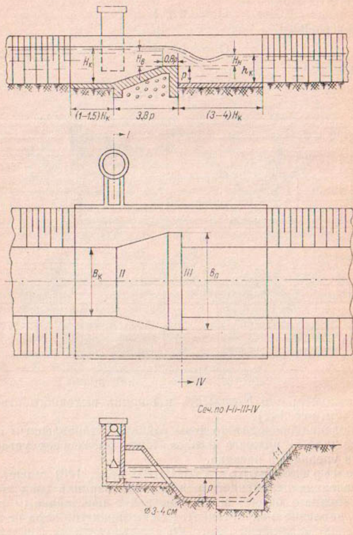
Рис. 143. Водомерный порог САНИИРИ.
