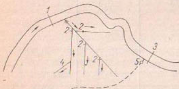
Рис. 139. Гидрометрические посты на оросительных системах.
