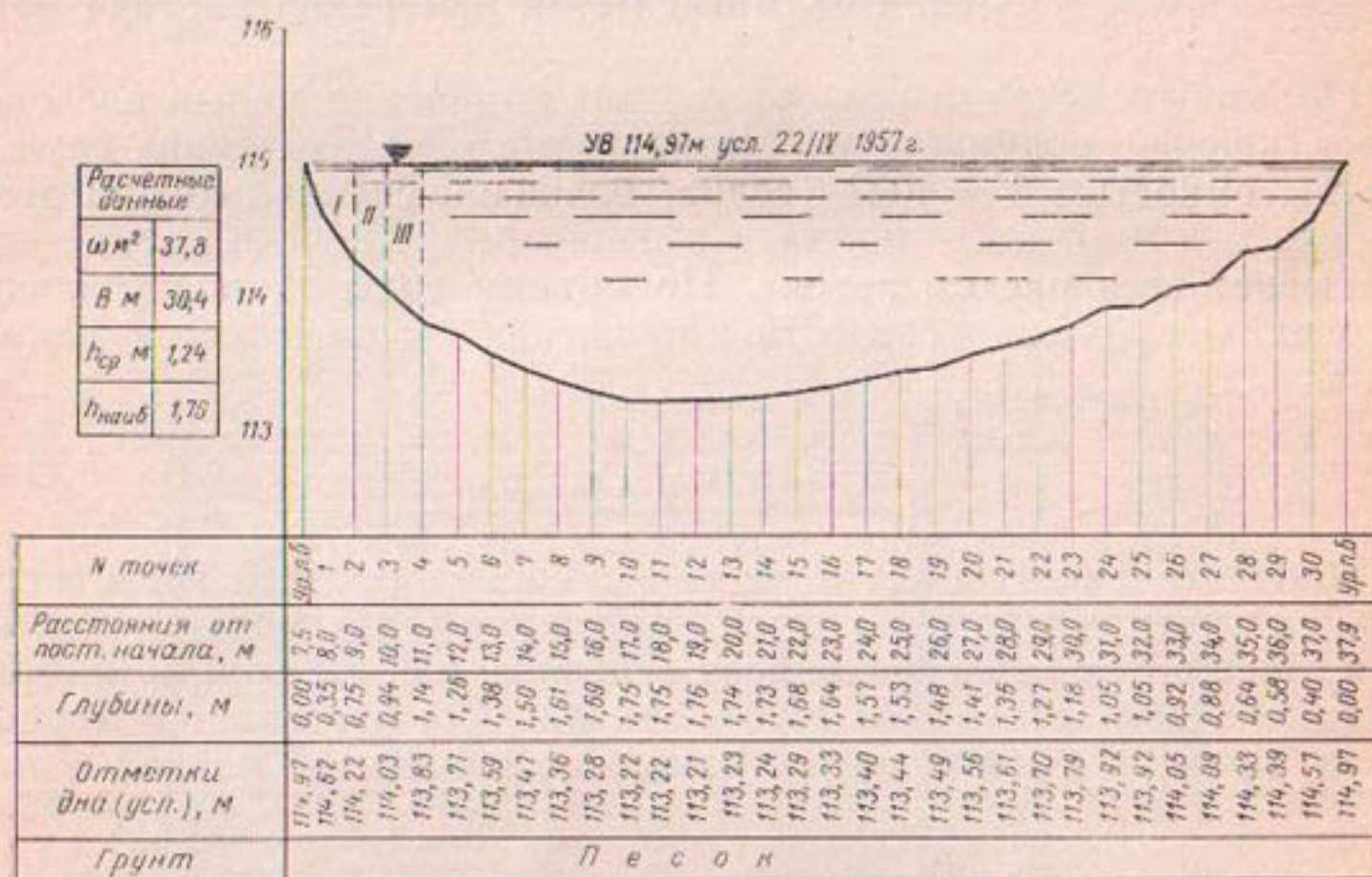
Рис. 125. Поперечный профиль оврага.
