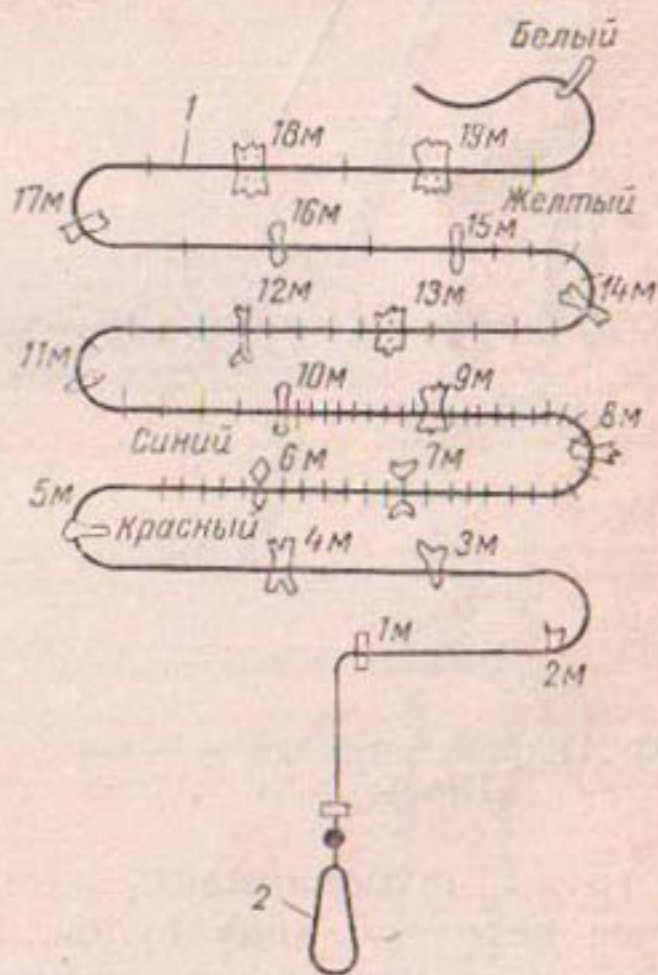
Рис. 102. Размеченный лотлинь. 1 — лотлинь; 2 — лот.
