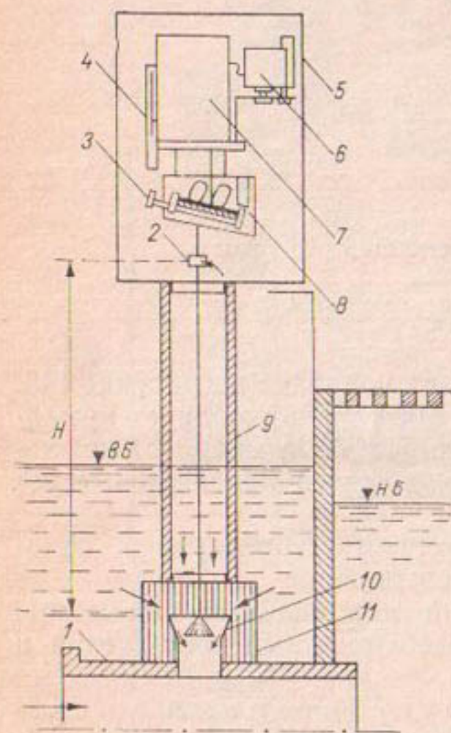
Рис. 148. Многопредельный расходоуказатель ДРС-66.
