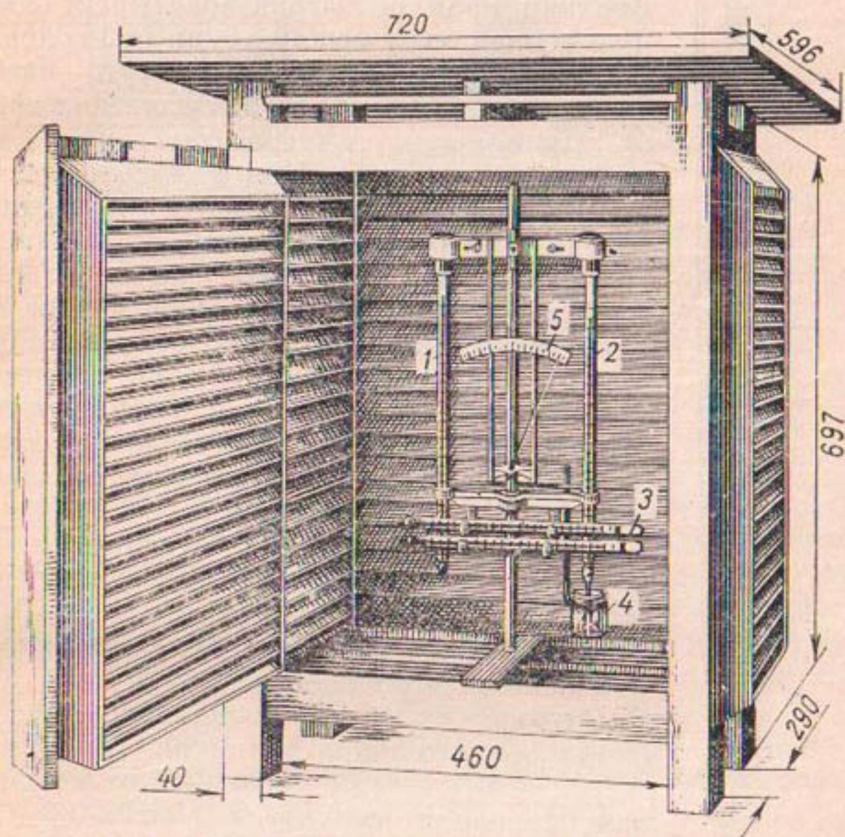
Рис. 3. Психрометрическая будка с установленными в ней приборами.
