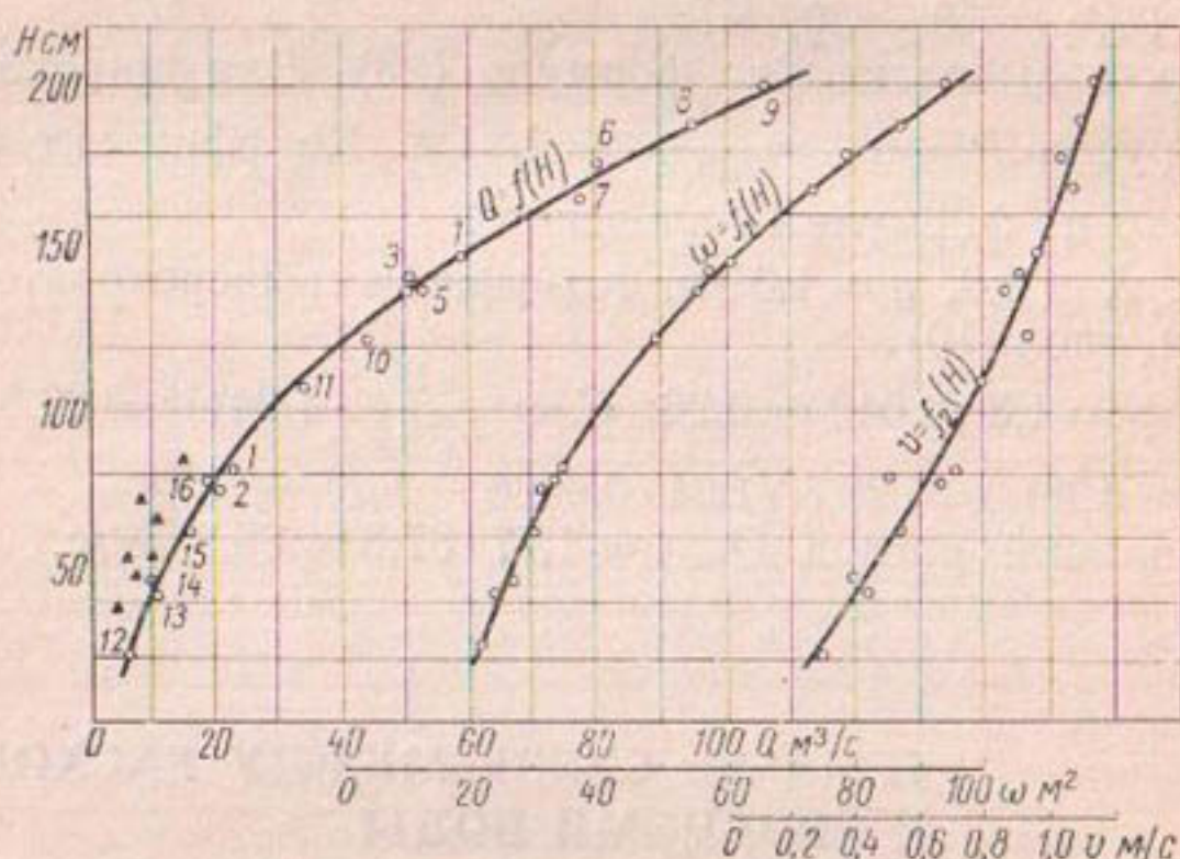
Рис. 126. Кривые расходов, площадей живого сечения и скоростей в зависимости от уровней.
