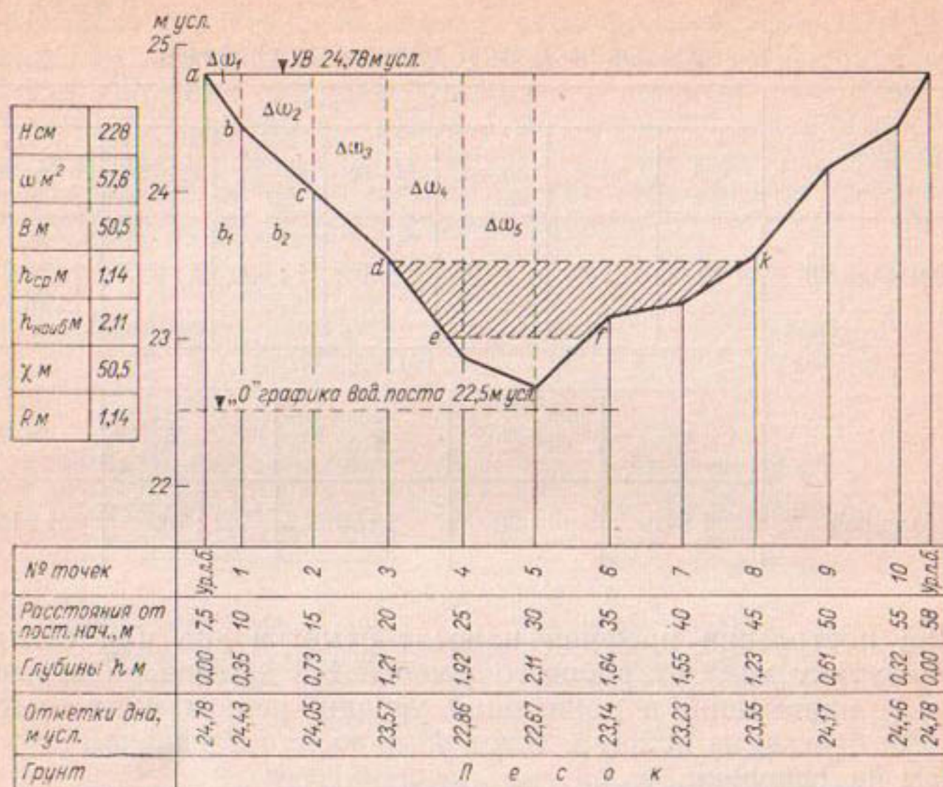
Рис. 110. Профиль водного сечения р. Супой у с. Песчаного.
