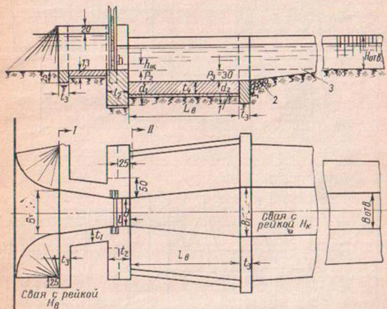
Рис. 144. Водовыпуск СБ-47. B = 1,70 b ; B_1 = 2 b .
