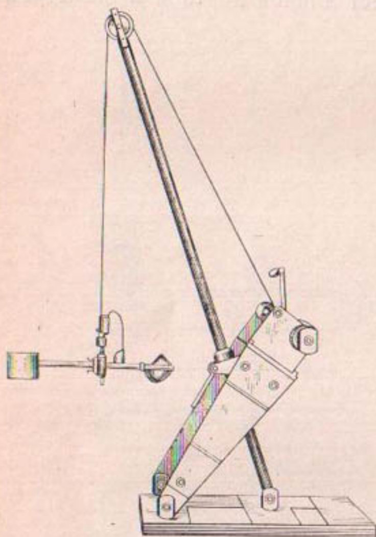
Рис. 103. Гидрометрическая лебедка «Нева».
