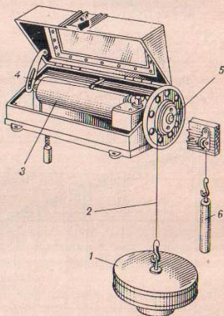
Рис. 85. Самописец уровня «Валдай». 1 — пустотелый поплавок; 2 — провод; 3 — барабан; 4 — каретка с пером; 5 — ко- лесо; 6 — противовес.
