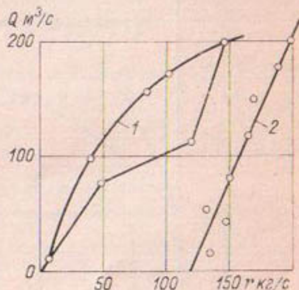
Рис. 136. Кривые зависимости расходов наносов от расходов воды.
