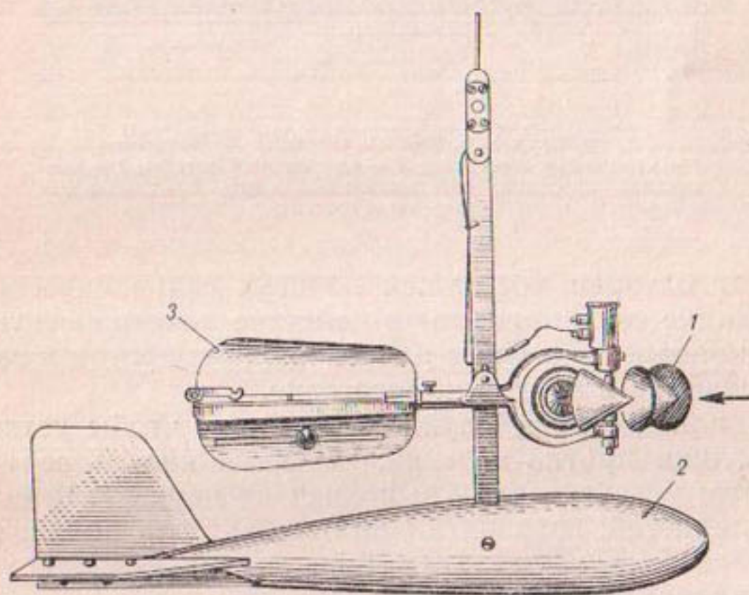
Рис. 118. Вертушка ИВХ.
