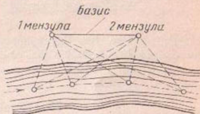
Рис. 107. Схема промеров по продольникам.
