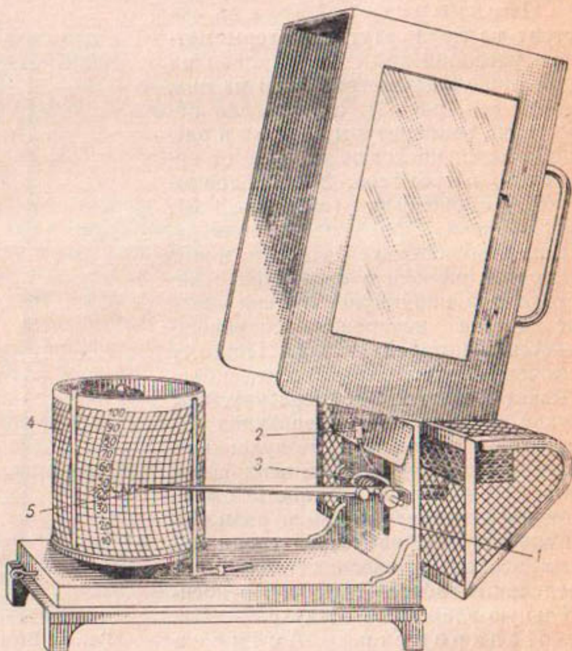
Рис. 8. Гигрограф.
