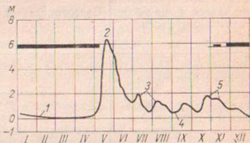
Рис. 42. График колебания уровней р. Днестра у г. Тирасполя.
