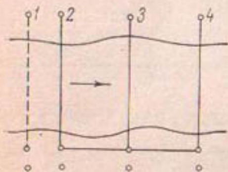
Рис. 115. Расположение створов для измерения скоростей поплавками.
