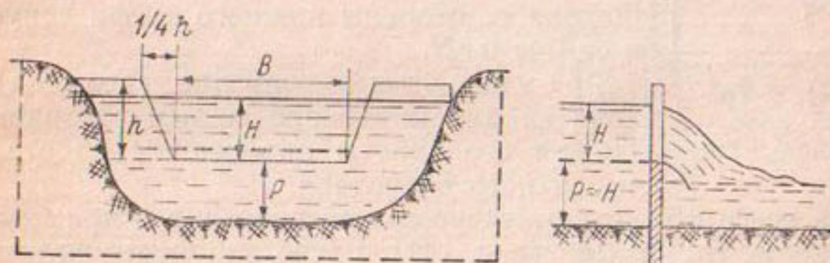
Рис. 140. Трапецеидальный водослив.
