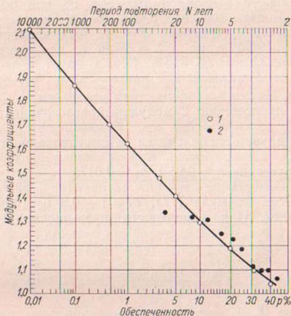
Рис. 66. Кривая обеспеченности модульных коэффициентов максимальных расходов р. Вятки у г. Кирова.
