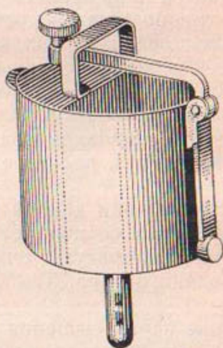
Рис. 10. Бюретка ГГИ.
