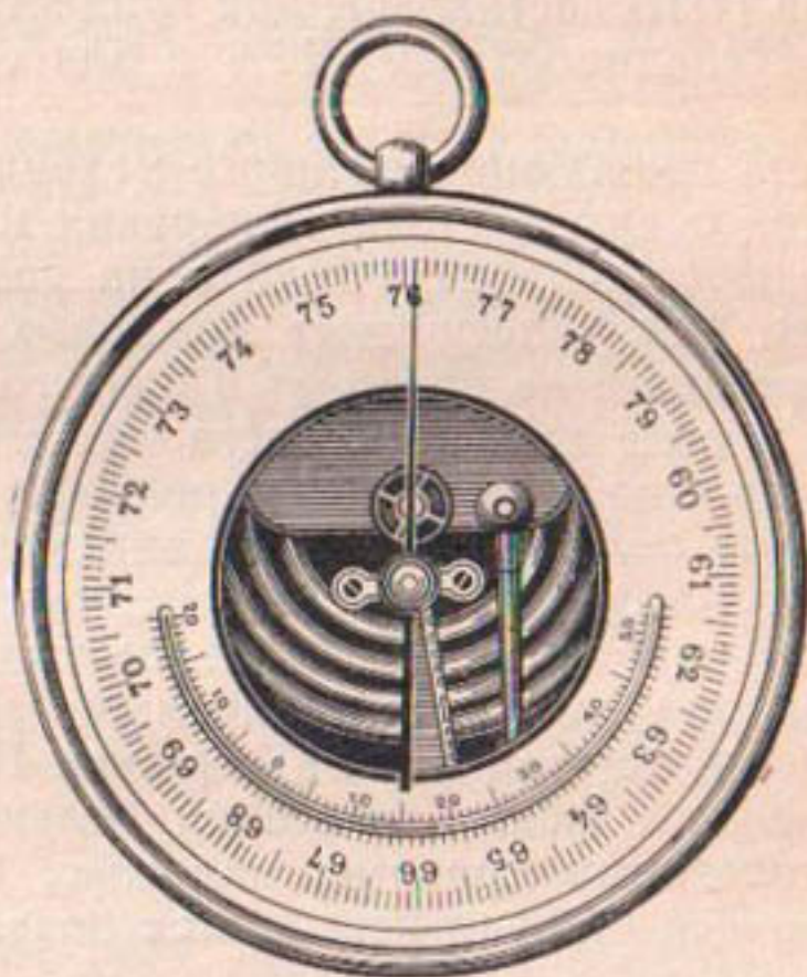
Рис. 27. Барометр aneroid.
