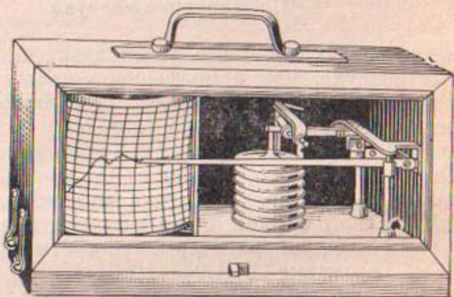
Рис. 28. Барограф.
