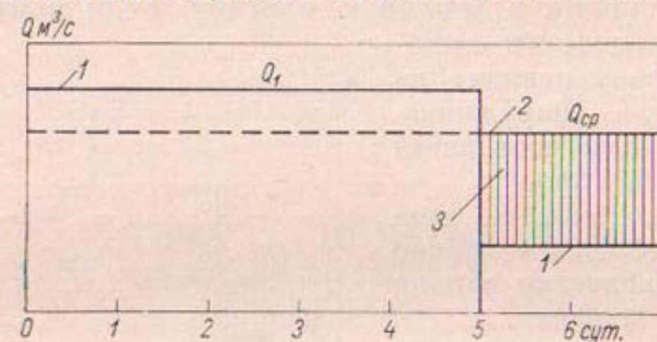
Рис. 76. Недельное регулирование.
