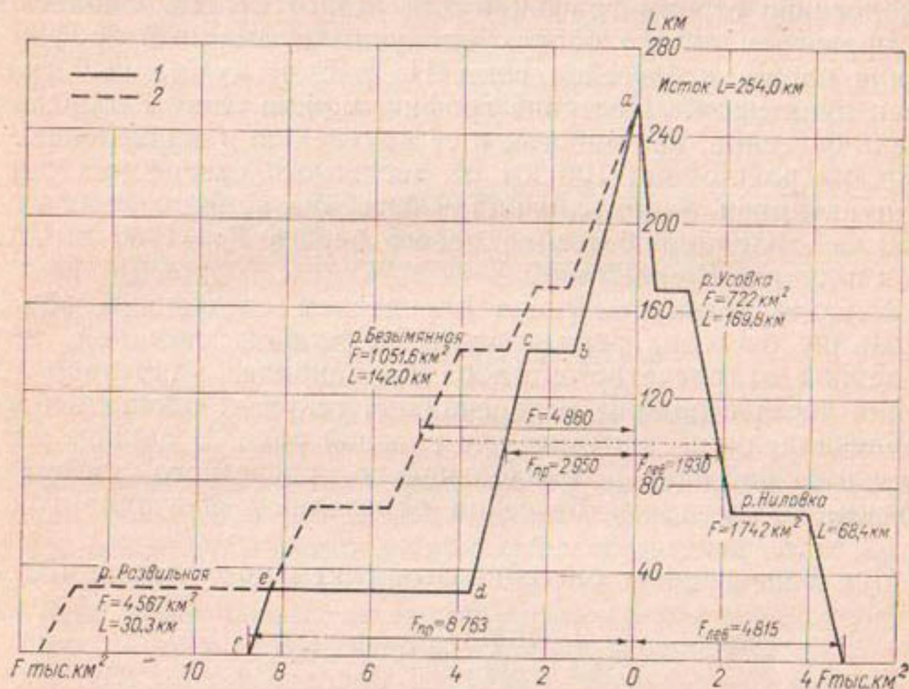
Рис. 47. График нарастания площади бассейна р. Раздольной. 1 — частная площадь бассейна по правому или левому берегу; 2 — суммарная площадь бассейна.
