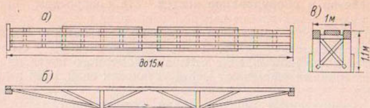
Рис. 90. Перекидной мостик. а — план; б — фасад; в — поперечный разрез.
