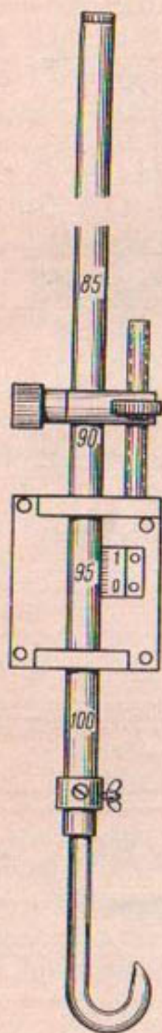
Рис. 84. Крючковая рейка.
