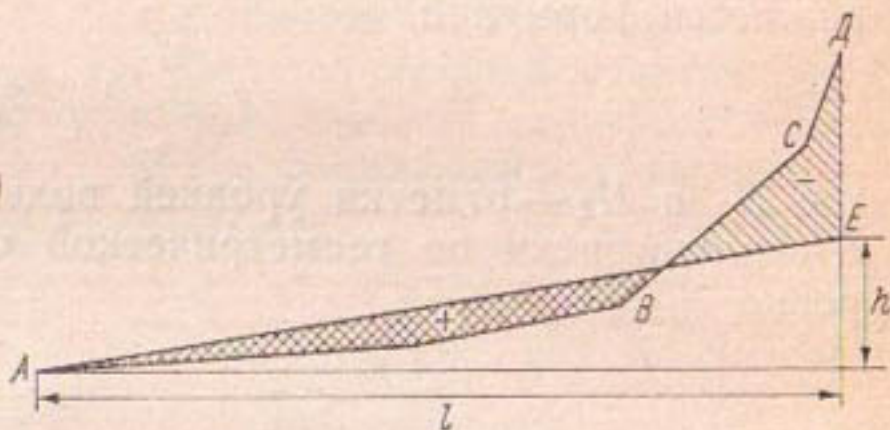
Рис. 39. Определение уклона выравненного продольного профиля реки.
