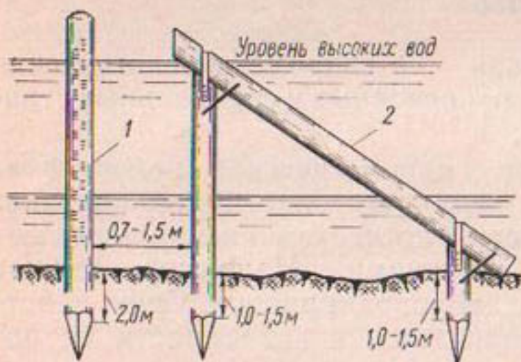
Рис. 80. Речной водомерный пост.
