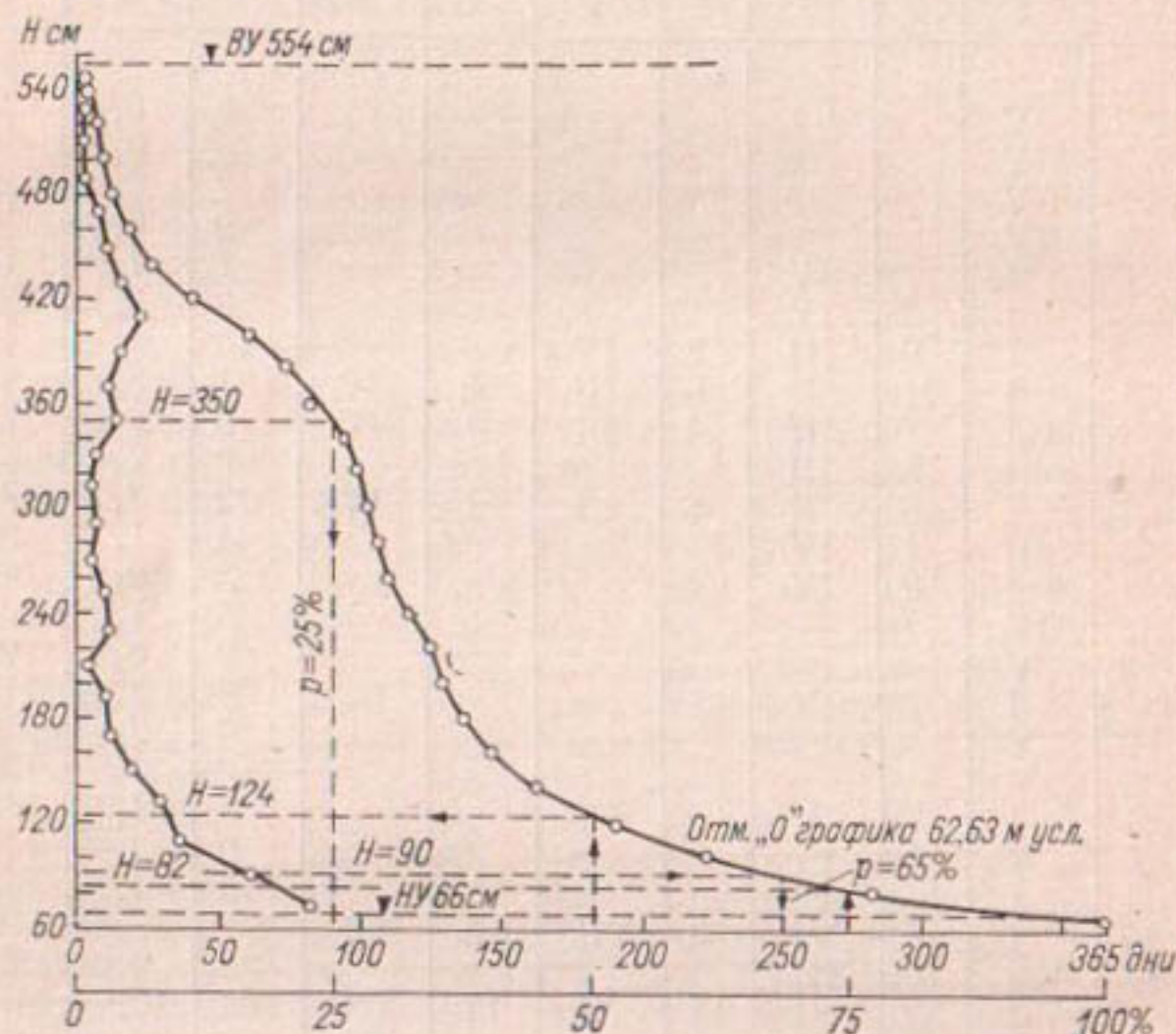
Рис. 99. Графики повторяемости (слева) и продолжительности стояния (справа) уровней воды р. Псел у с. Запселья за 1955 г.
