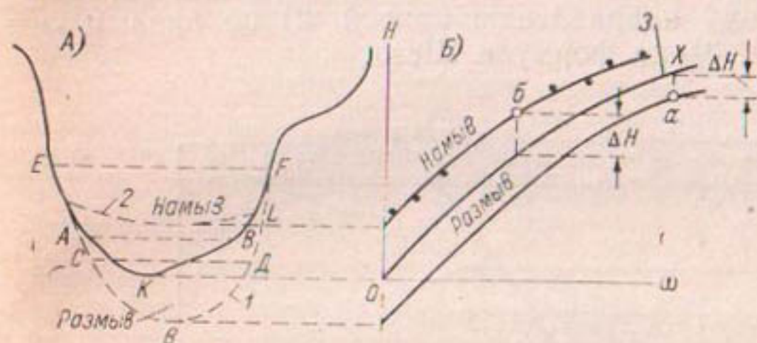
Рис. 129. Приведение промеров к основному сечению.
