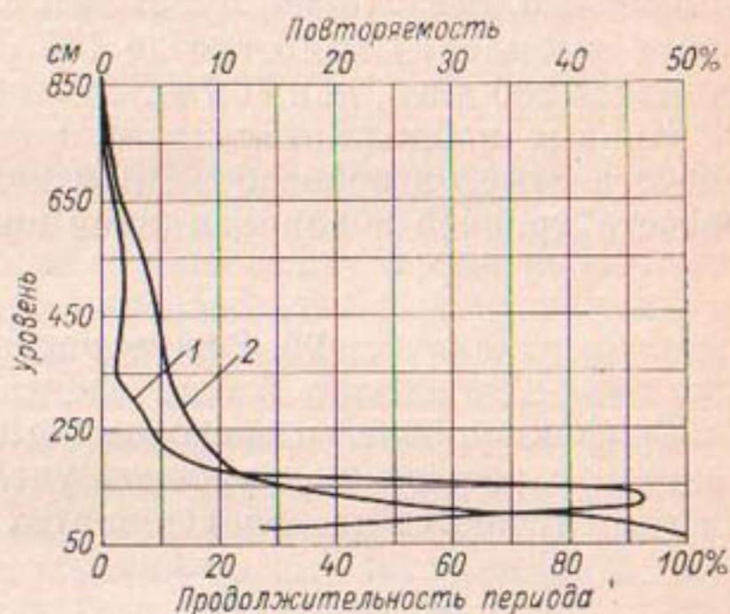
Рис. 43. Кривые повторяемости (1) и продолжительности (2) стояния уровней воды.
