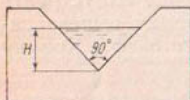
Рис. 141. Треугольный водослив.
