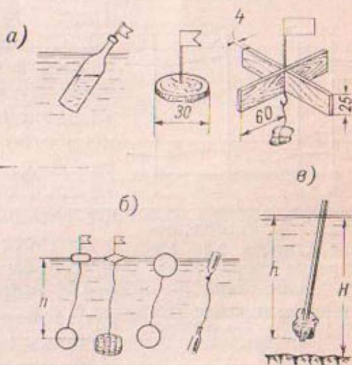
Рис. 114. Поплавки.
