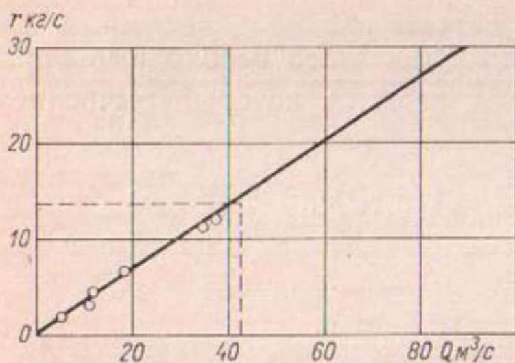
Рис. 72. Зависимость средних годовых расходов наносов от среднегодового расхода воды р. Синюхи у с. Синюхина Брода.
