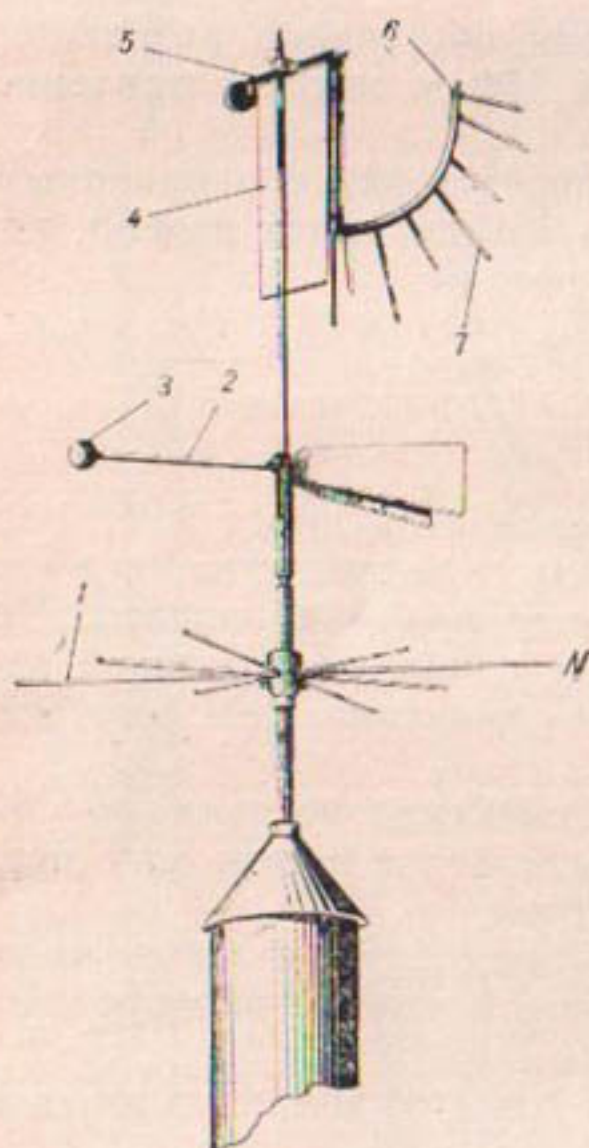
Рис. 29. Флюгер Вильда.
