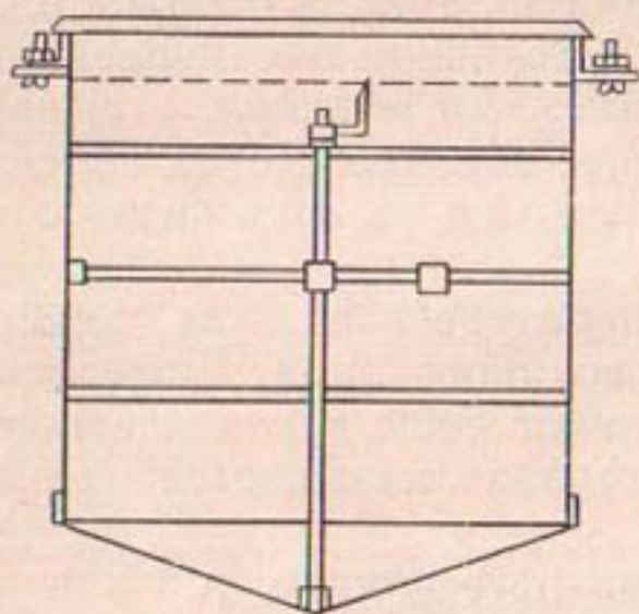
Рис. 9. Испаритель ГГИ-3000.
