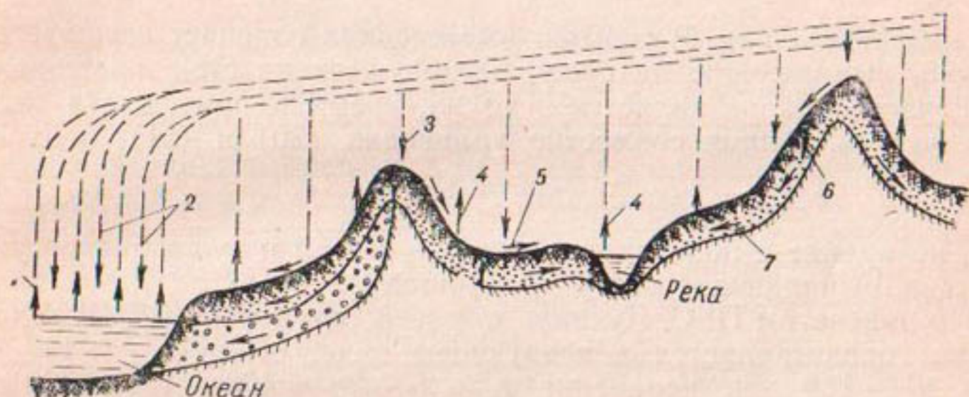
Рис. 34. Схема круговорота воды в природе.
