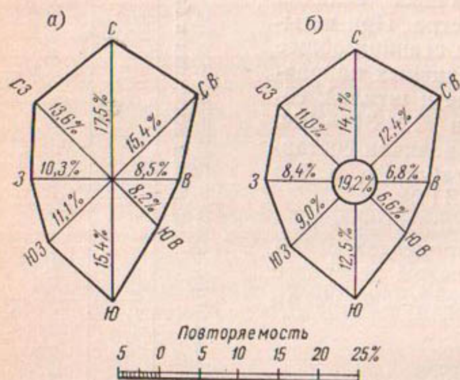
Рис. 33. Розы ветров для метеорологической станции Озерная.
