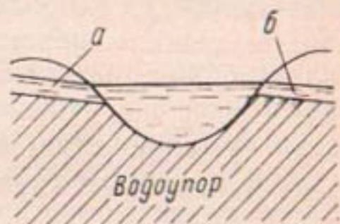
Рис. 48. Направление движения грунтовых вод в водоносном горизонте, прорезанном руслом реки.
