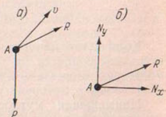
Рис. 70. Схема действия сил на взвешенную в воде частичку грунта.
