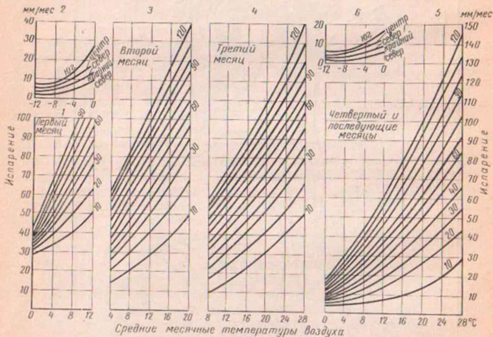
Рис. 15. Зависимость испарения с поверхностных речных бассейнов от температуры воздуха и суммы осадков (по Б. В. Полякову).
