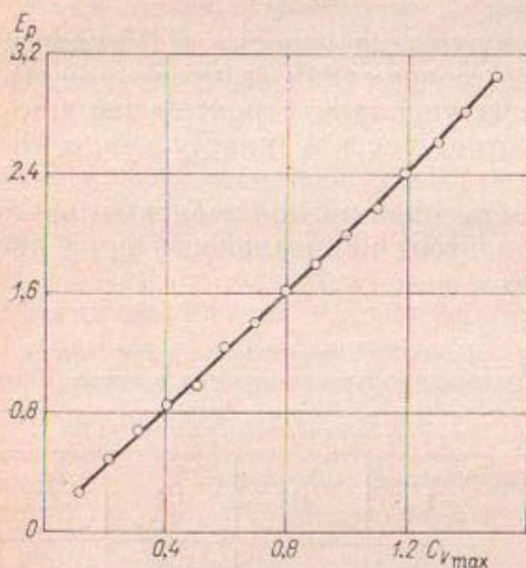
Рис. 59. Ошибка E_p максимального расчетного расхода обеспеченностью 0,01% при разных значениях коэффициента вариации C_{v\max} .
