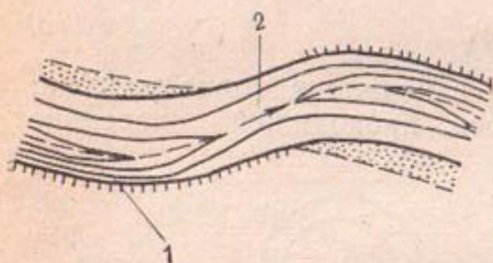
Рис. 38. Чередуемость плесов и перекатов в плане. 1 — плес; 2 — перекат.
