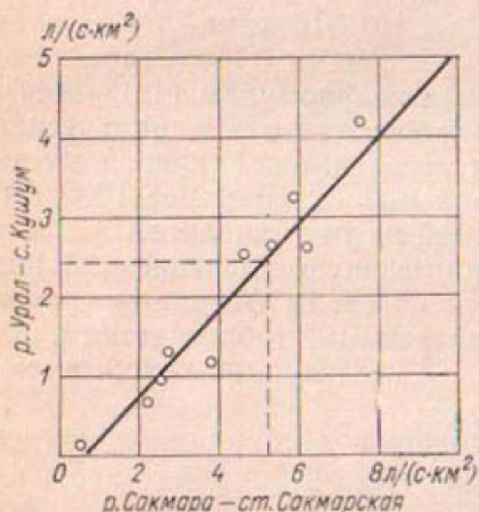
Рис. 54. Связь между годовыми величинами стока р. Урала у с. Кушум и р. Сакмары у ст. Сакмарской.
