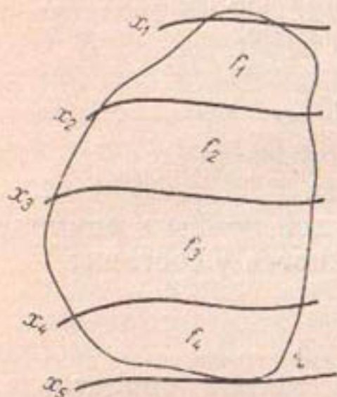
Рис. 24. Вычисление средней суммы осадков методом изогнет.
