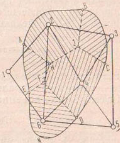
Рис. 25. Вычисление среднего количества осадков для территории методом взвешивания.
