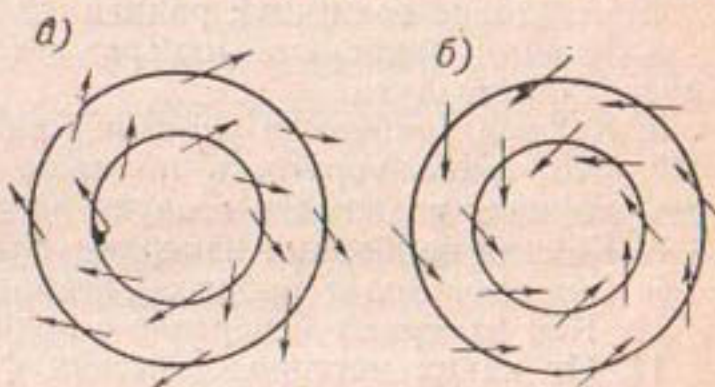
Рис. 31. Схема движения воздушных масс.
