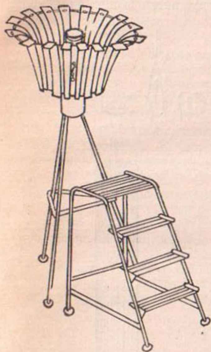
Рис. 20. Осадкомер Третьякова.
