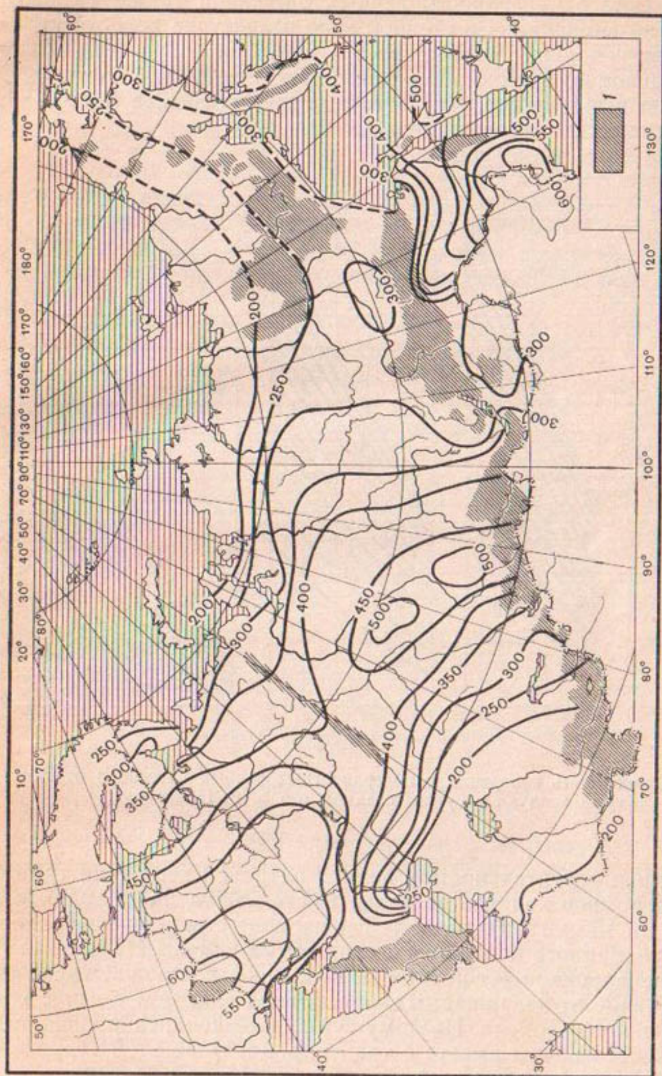
Рис. 14. Среднее многолетнее испарение с речных бассейнов (мм). 1 — горные районы.
