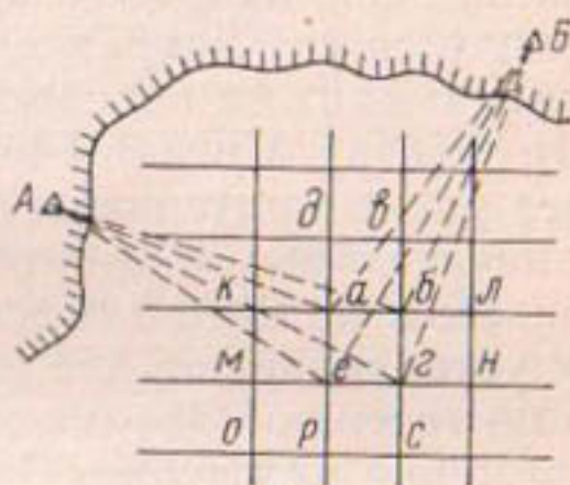
Рис. 109. Промеры по квадратам.
