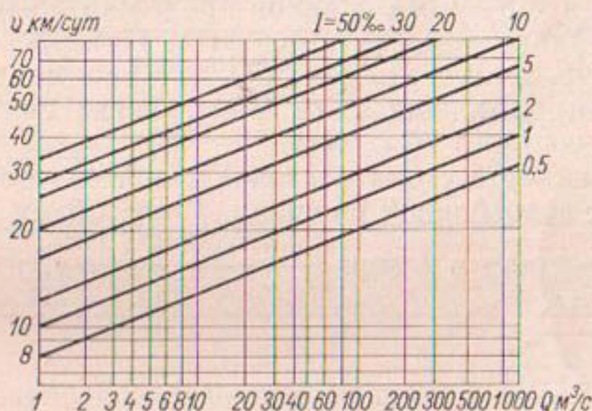
Рис. 62. Скорость добега в зависимости от максимального расхода при разных уклонах.
