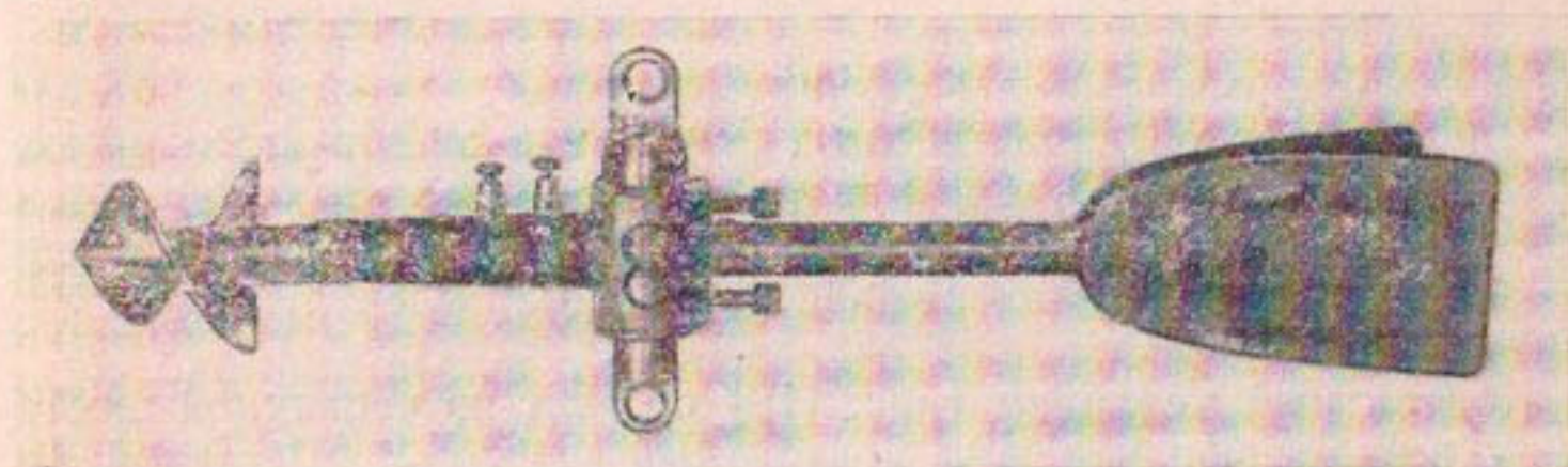
Рис. 117. Вертушка ВБ-61.
