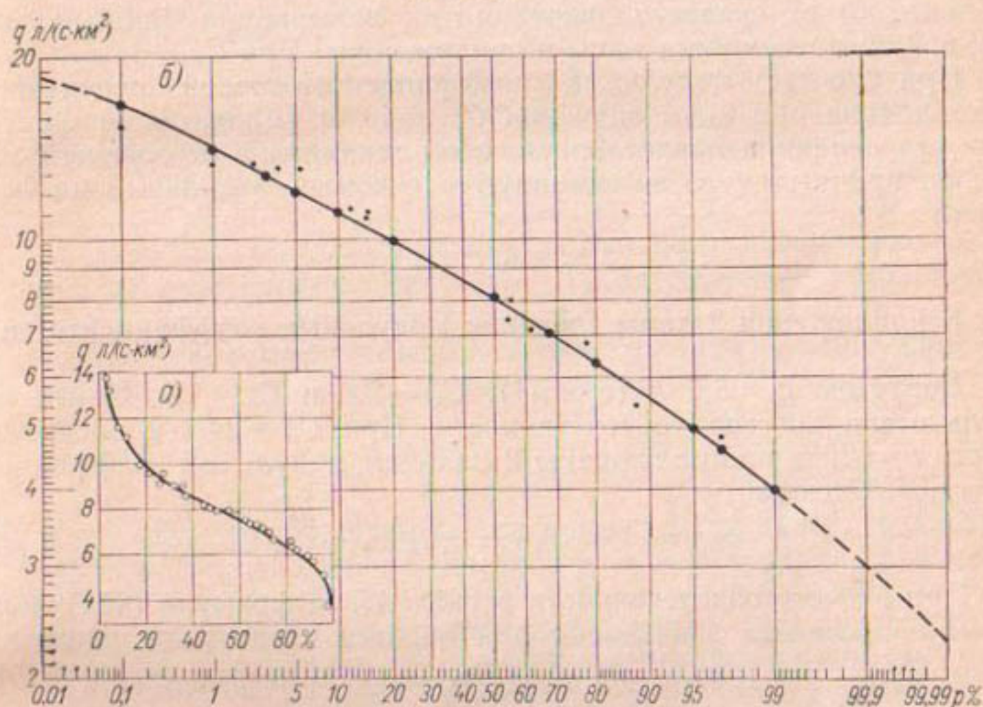
Рис. 53. Кривая обеспеченности модулей годового стока p . Западной Двины у г. Витебска.
