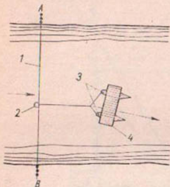
Рис. 94. Паром-самолет.
