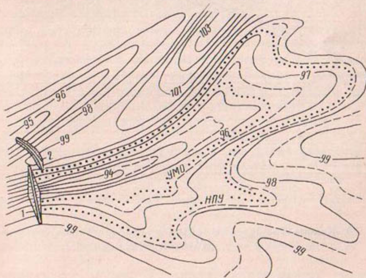
Рис. 78. План водохранилища в горизонталях.
