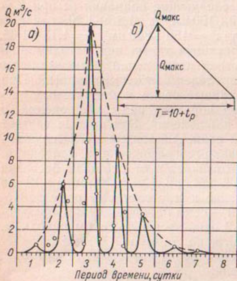
Рис. 61. К расчету максимальных расходов с малых водосборов.
