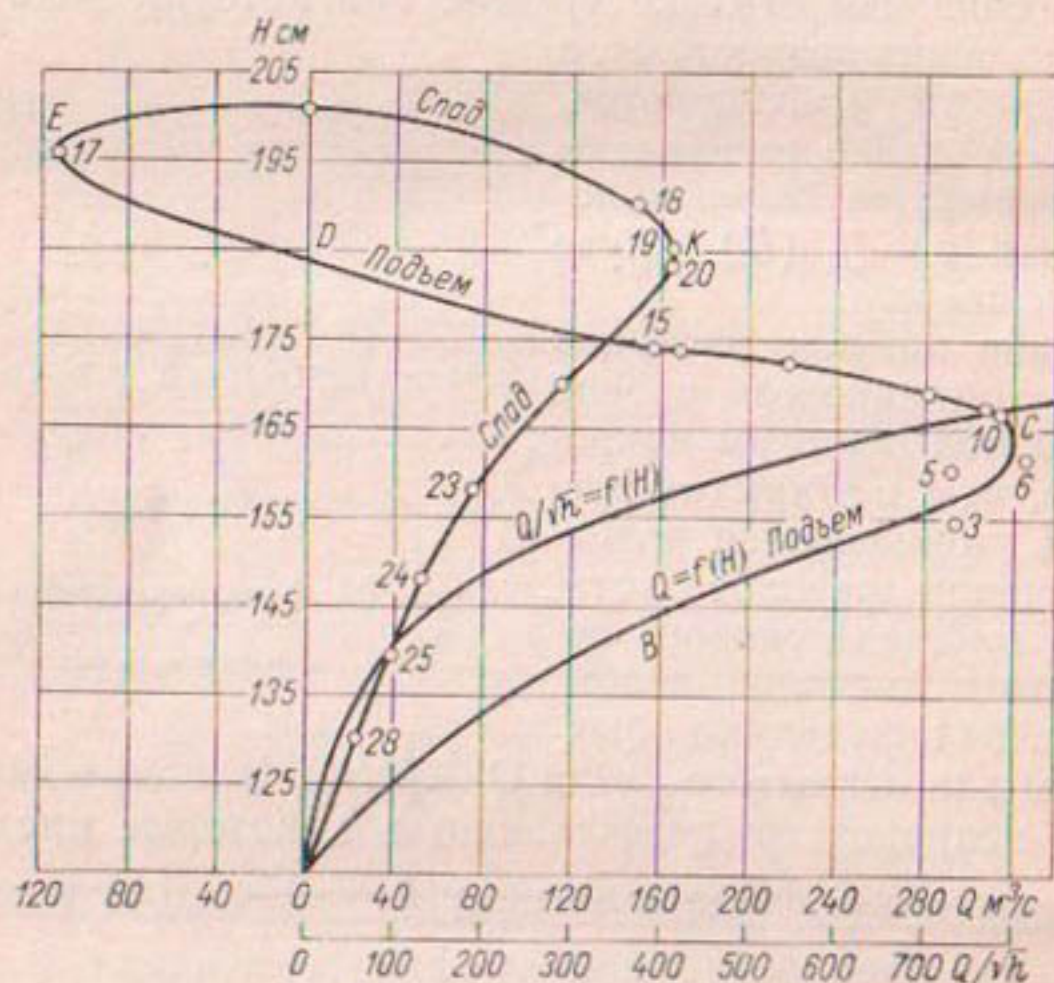
Рис. 128. Кривая расходов в условиях переменного подпора на р. Большой Иргиз у с. Малая Быковка.
