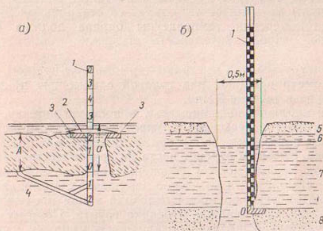
Рис. 95. Ледомерные рейки.
