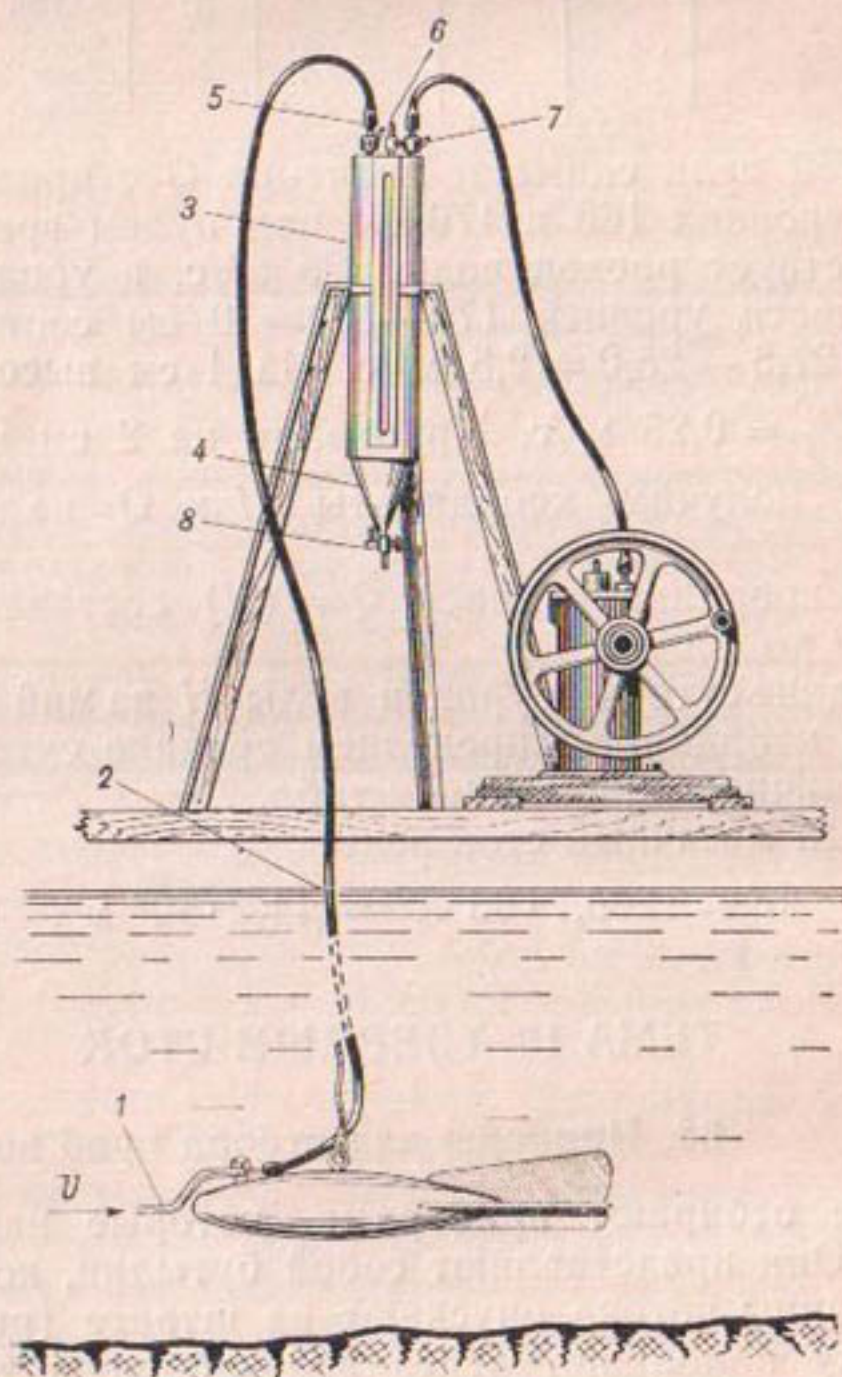
Рис. 134. Вакуумный батометр.
