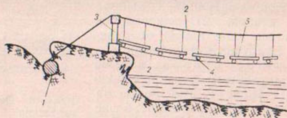
Рис. 91. Подвесной мостик. 1 — мертвый якорь; 2 — тросы; 3 — подпорная рама; 4 — бруски; 5 — настил.
