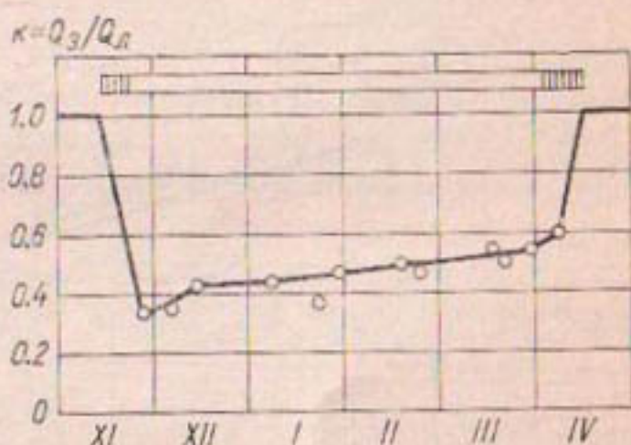
Рис. 127. График колебания коэффициента k = \frac{Q_z}{Q_{\text{л}}} .
