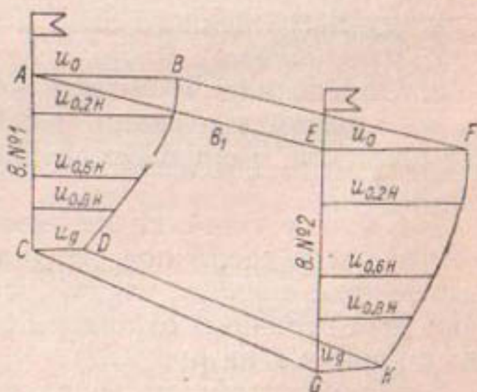
Рис. 121. Модель частичного расхода воды.
