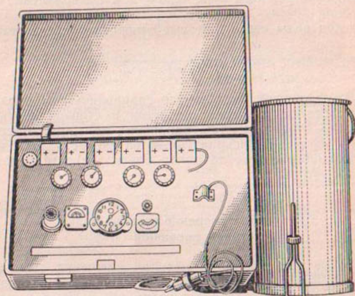
Рис. 124. Измеритель расхода воды ИРВ-52.
