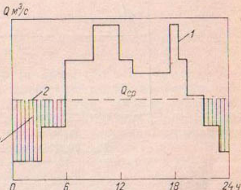
Рис. 75. Суточное регулирование стока. 1 — водопотребление; 2 — расходы реки (приток), 3 — накопление.
