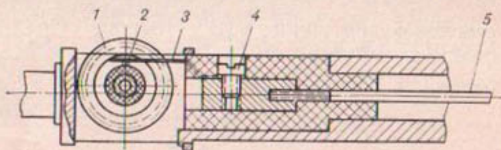
Рис. 119. Счетно-контактный механизм.
