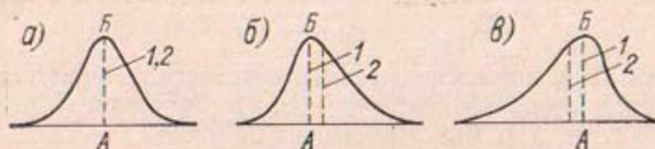
Рис. 52. Основные типы кривых распределения. а — симметричная кривая; б и в — асимметричные кривые; 1 — мода, 2 — средняя арифметическая.
