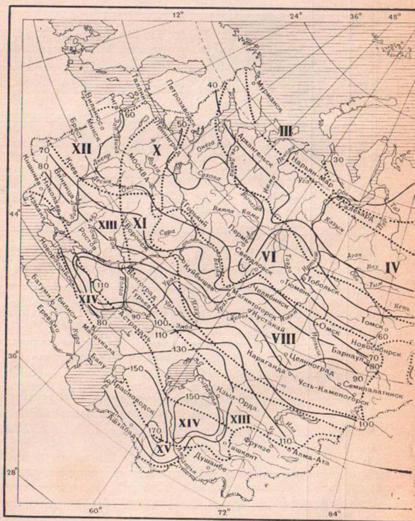
Рис. 11. Испарение с водной поверхности малых водоемов I — изолинии испарения в сантиметрах;
