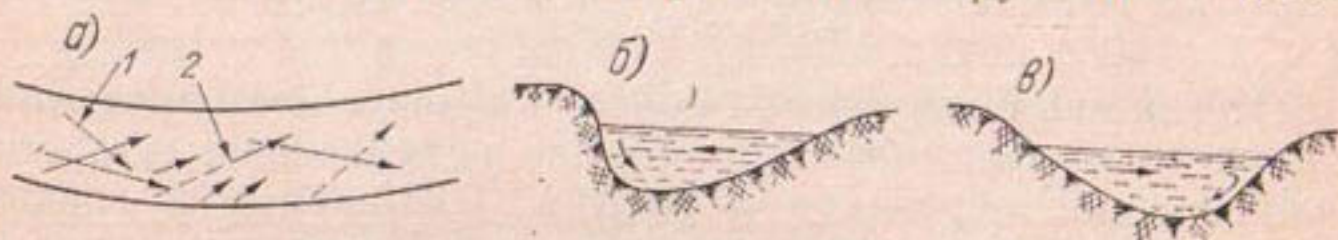
Рис. 69. Образование поперечной циркуляции.
