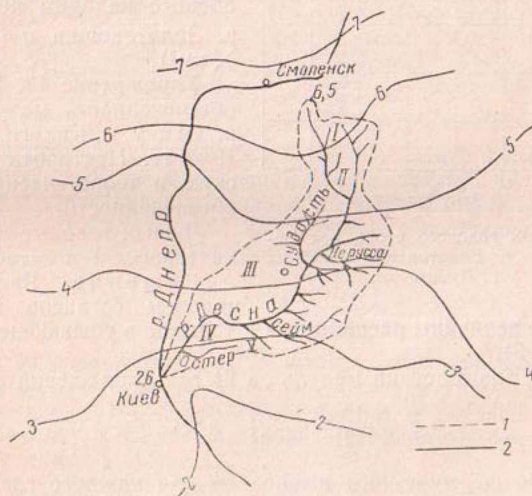
Рис. 56. Годовой сток в бассейне р. Десны. 1 — водораздел, 2 — изолинии модуля стока в л/(с · км 2 ).
