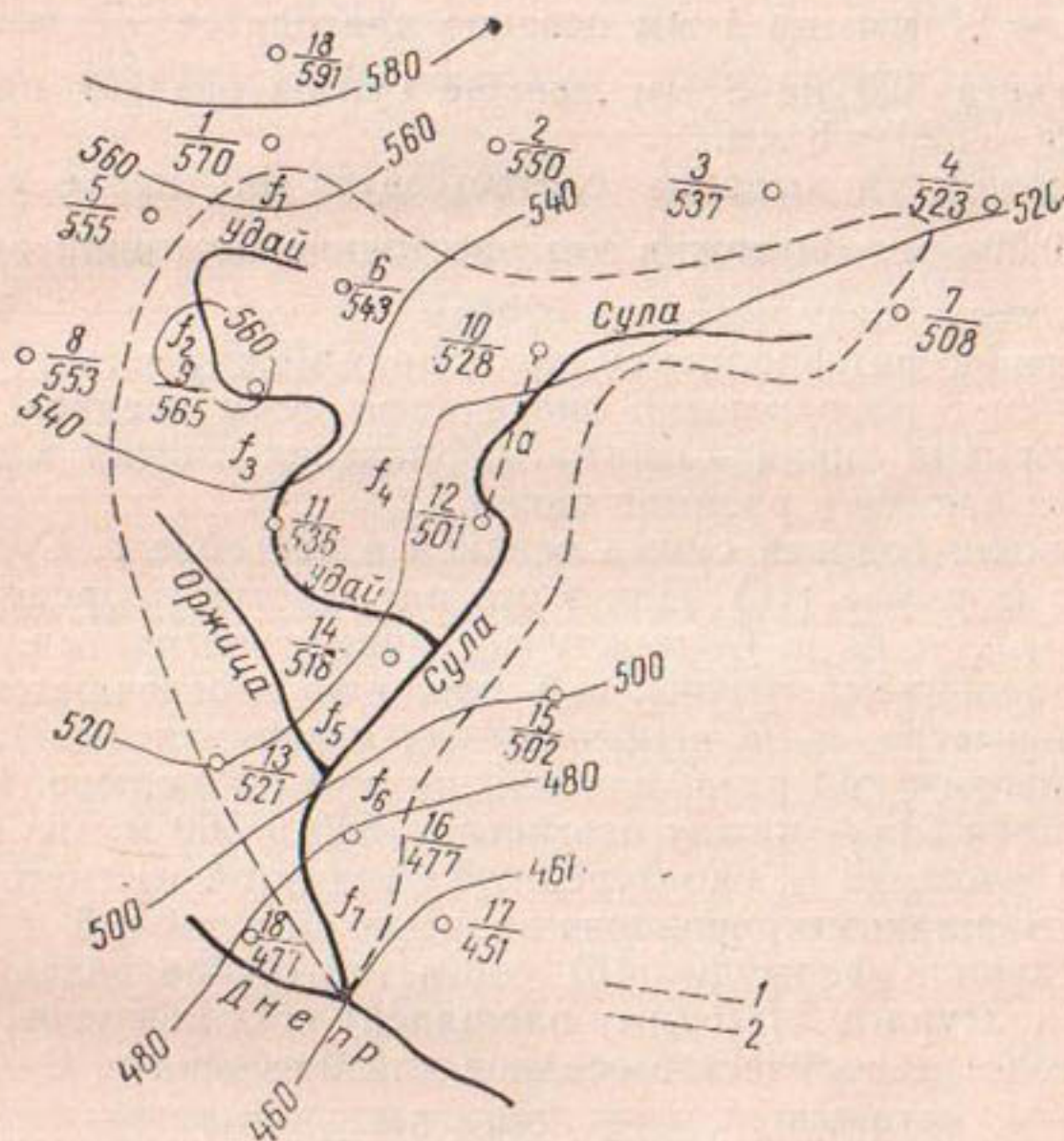
Рис. 32. Определение среднего количества осадков для бассейна р. Сулы методом изогнет:
