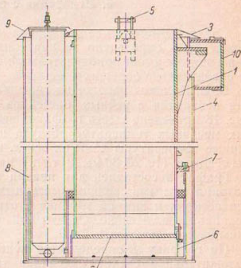
Рис. 13. Лизиметр ГР-80.
