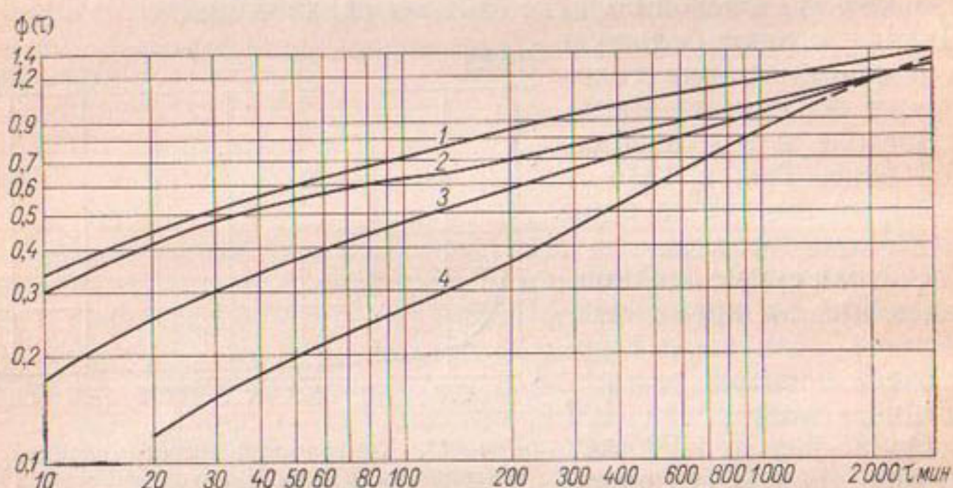
Рис. 18. Типовые кривые редукции слоя осадков в зависимости от интервала времени.
