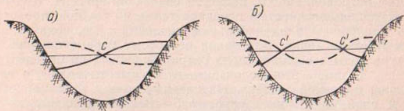
Рис. 74. Сейши.
