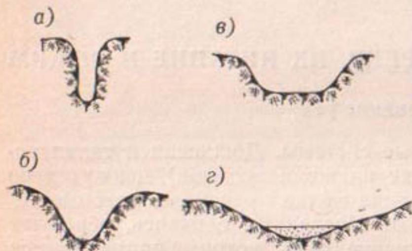
Рис. 35. Форма долин.
