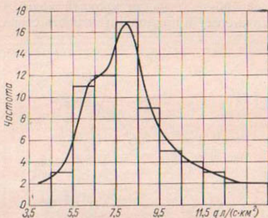
Рис. 51. Кривая распределения частот модулей стока р. Западной Двины у г. Витебска.
