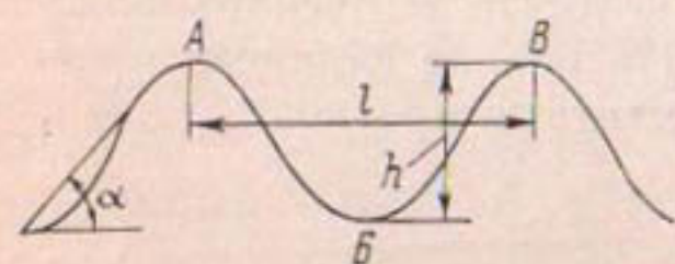
Рис. 73. Элементы волны.
