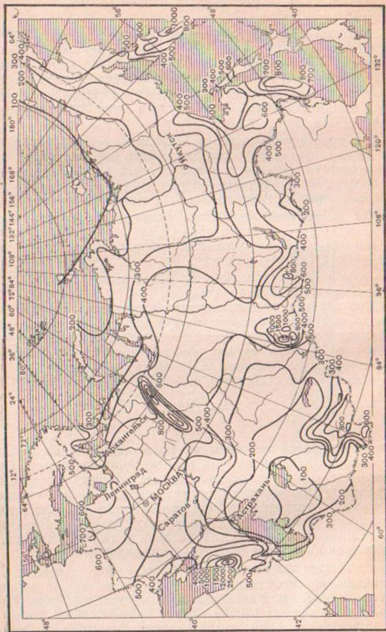
Рис. 23. Средние многолетние годовые суммы осадков на территории СССР.
