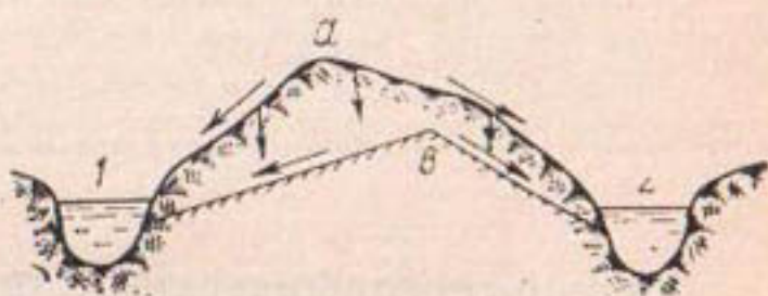
Рис. 41. Несовпадение вершин поверхностного (а) и подземного (б) водоразделов.
