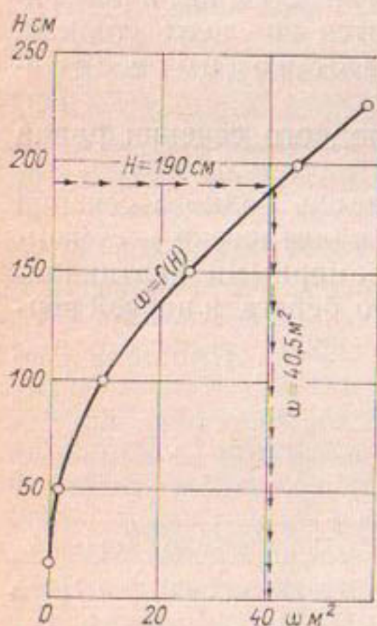
Рис. 111. Кривая зависимости площадей водного сечения от уровней воды р. Супой у с. Песчаного.
