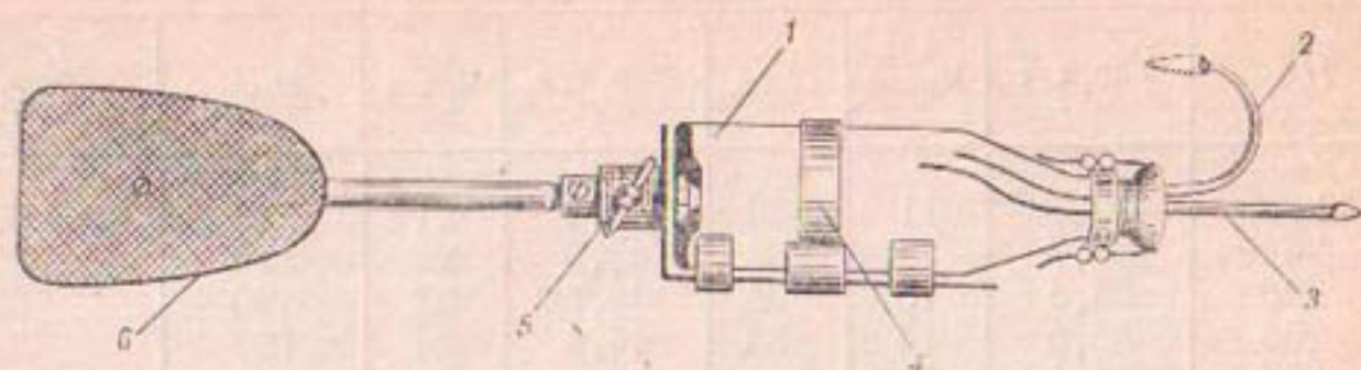
Рис. 133. Батометр-бутылка на штанге.
