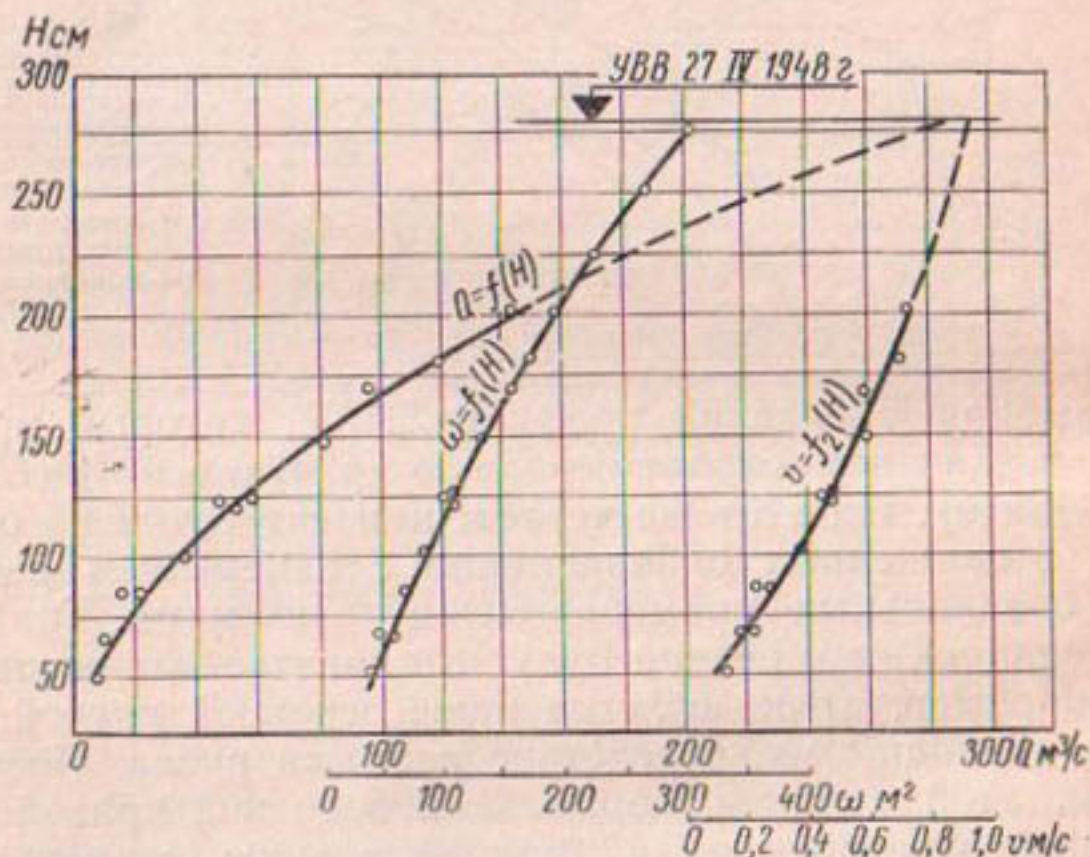
Рис. 131. Экстраполяция кривой Q = f(H) .
