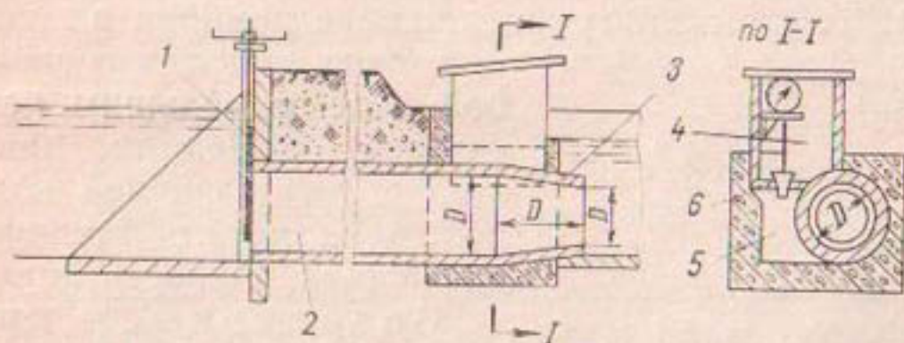
Рис. 146. Трубчатый водомер-регулятор со сходящимся насадком.
