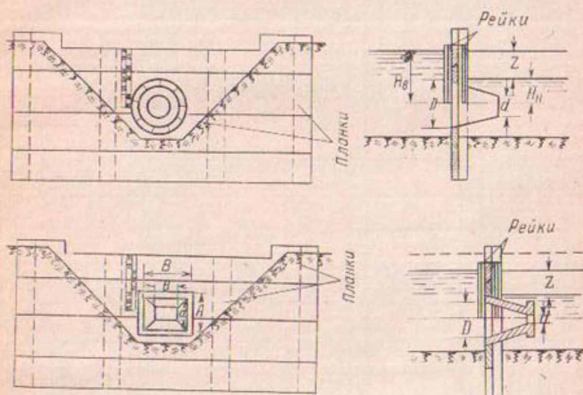
Рис. 142. Насадки-водомеры
