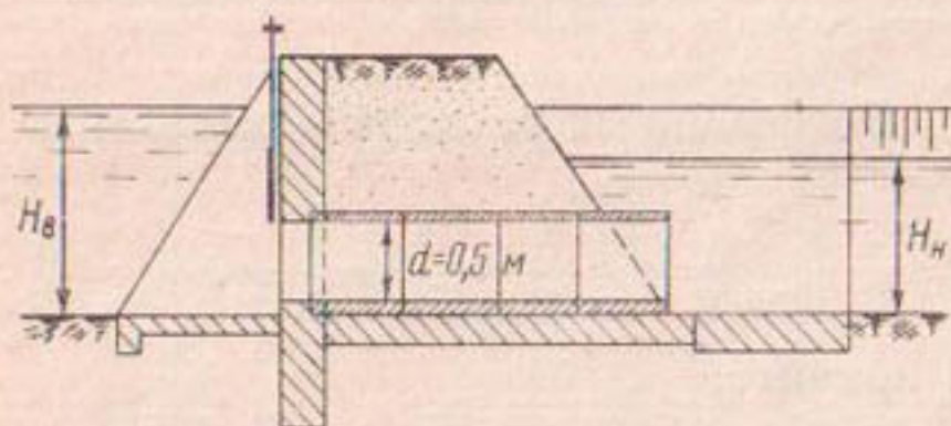
Рис. 149. Трубчатый водовыпуск.
