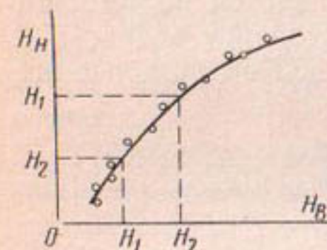
Рис. 97. График связи соответственных уровней.
