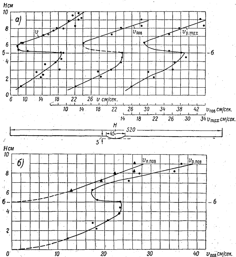
Рис. 10-6. Зависимость средней скорости всего потока v , средней поверхностной скорости всего потока v_{п.пов} , максимальной скорости v_{р.мах} (на оси русла) (а), средней поверхностной скорости в основном русле v_{р.пов} и средней поверхностной скорости в пойме v_{п.пов} (б) от уровня воды по опытам 1947 г.
