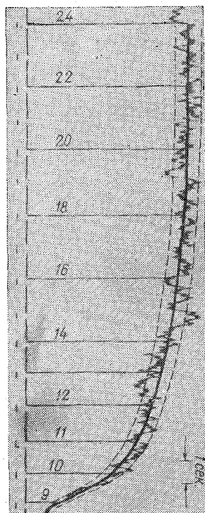
Рис. 6-9. Осциллограмма записи выходного сигнала при интеграционном способе измерения скоростей с помощью круглой металлической пластинки с собственной частотой 80 гц при скорости ее подъема w = 0,76 см/сек.
