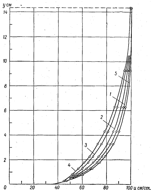
Рис. 6-5. Эпюры скоростей, измеренные интеграционным (1, 2, 3, 4) и точечным (5) способами с помощью гидрометрической трубки с динамическим отверстием d = 0,85 мм.
