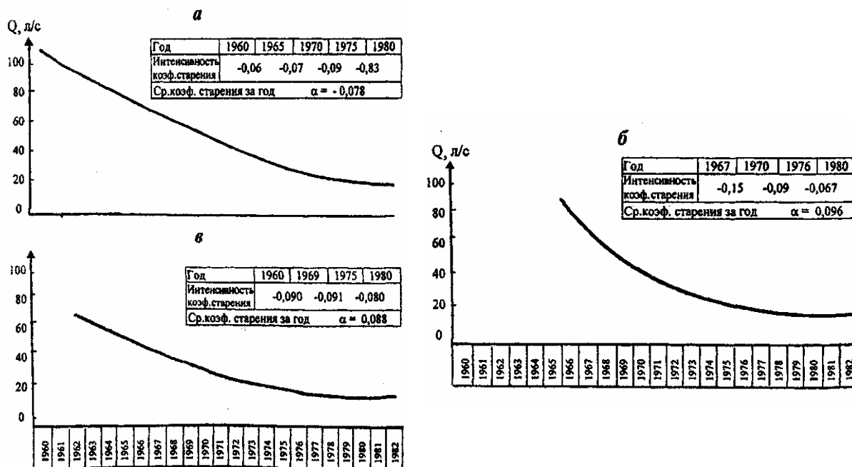
Рис.5.5. Изменение дебита скважин в процессе физико-химического коьматажа в зависимости от продолжительности их работы при: а – карбонатизации; б – коррозионных явлениях; в – смешанных процессах
