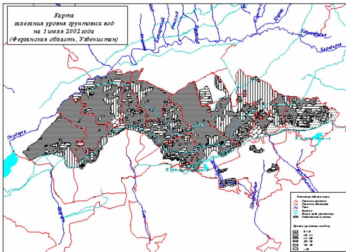
Рис. 6.3.1.9 Карта УГВ на июль 2002 г.
