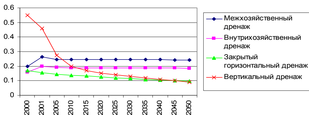
Доля дренажной сети требующей, полной реконструкции. Сценарий 2.
