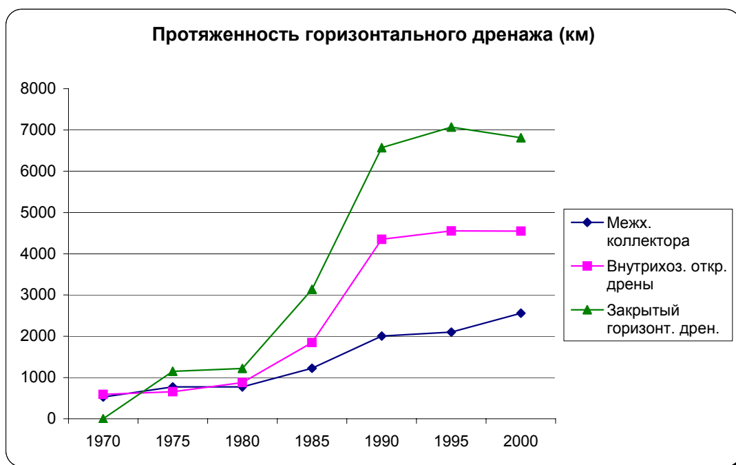
Рис 6.6.1.4.1 Горизонтальный дренаж Кашкадарьинской области
