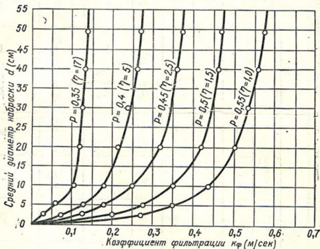
Р и с. 29. График зависимости коэффициента фильтрации от грансостава каменной наброски.
