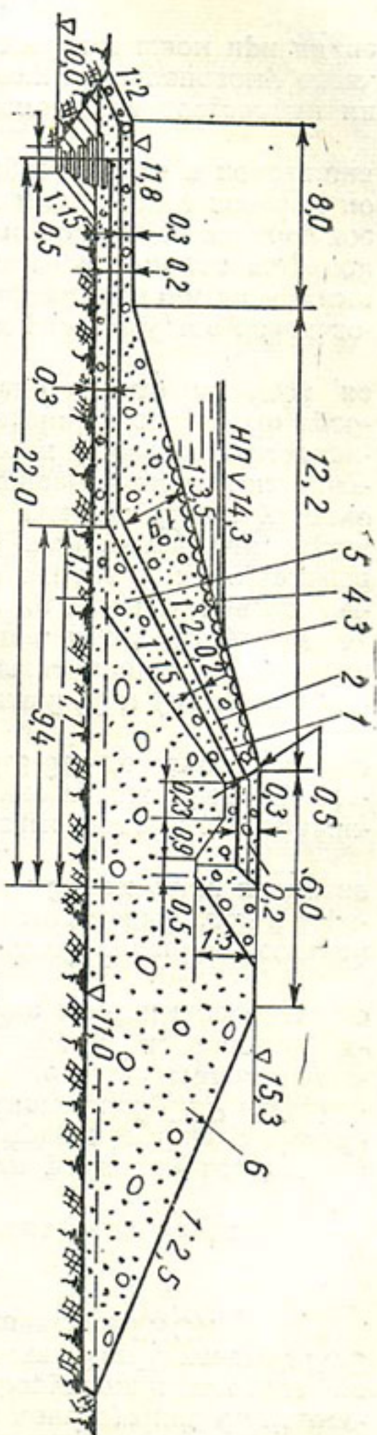
Рис. 19. Поперечный разрез по плотине на р. Карасу.
