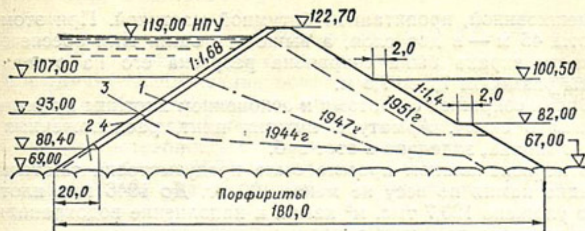
Р и с. 11. Поперечный профиль по Кассансайской плотине.
