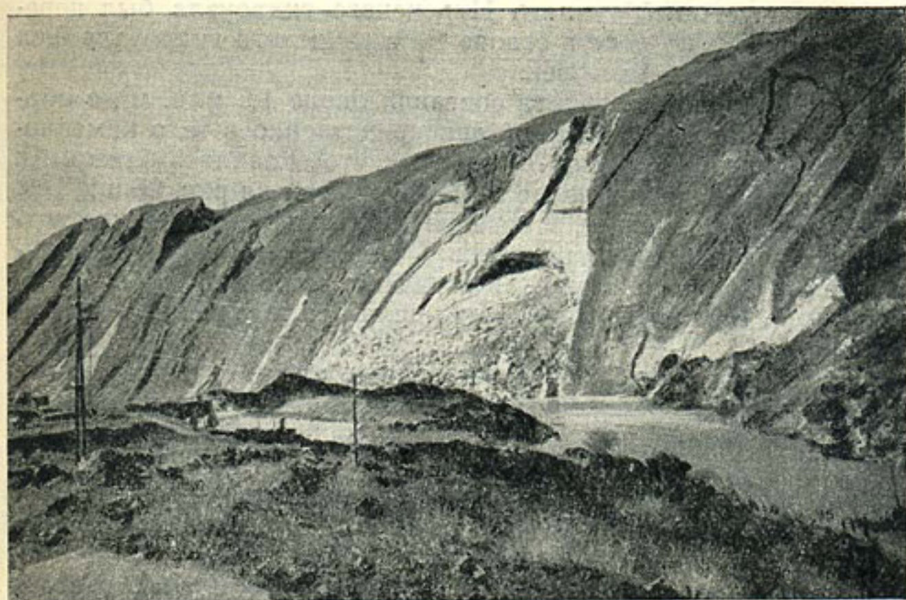
Р и с. 26. Панорама Байпазинского гидроузла со стороны верхнего бьефа после взрыва.
