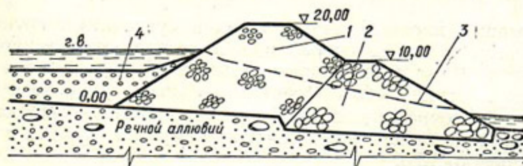
Рис. 30. Фильтрующая плотина на р. Басмандысай.
