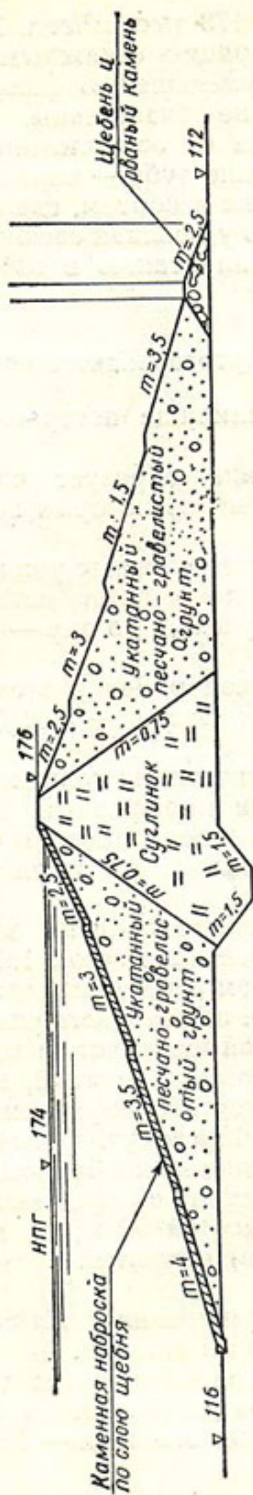
Рис. 12. Поперечный разрез насыпной плотины Каттасайского водохранилища.
