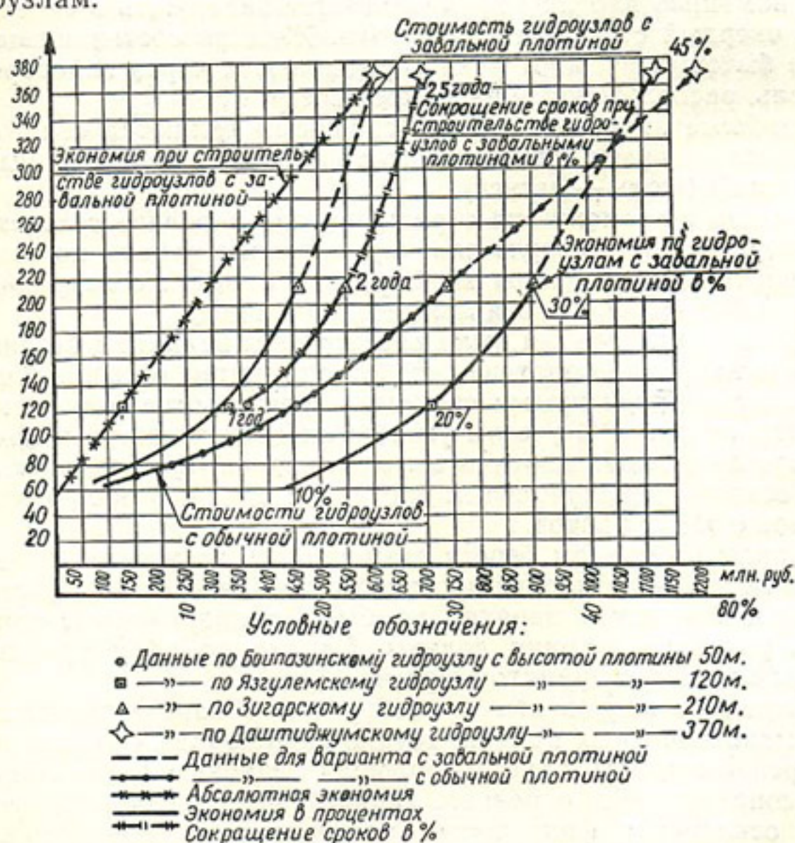
Рис. 23. График эффективности возведения гидроузлов с завальными плотинами.
