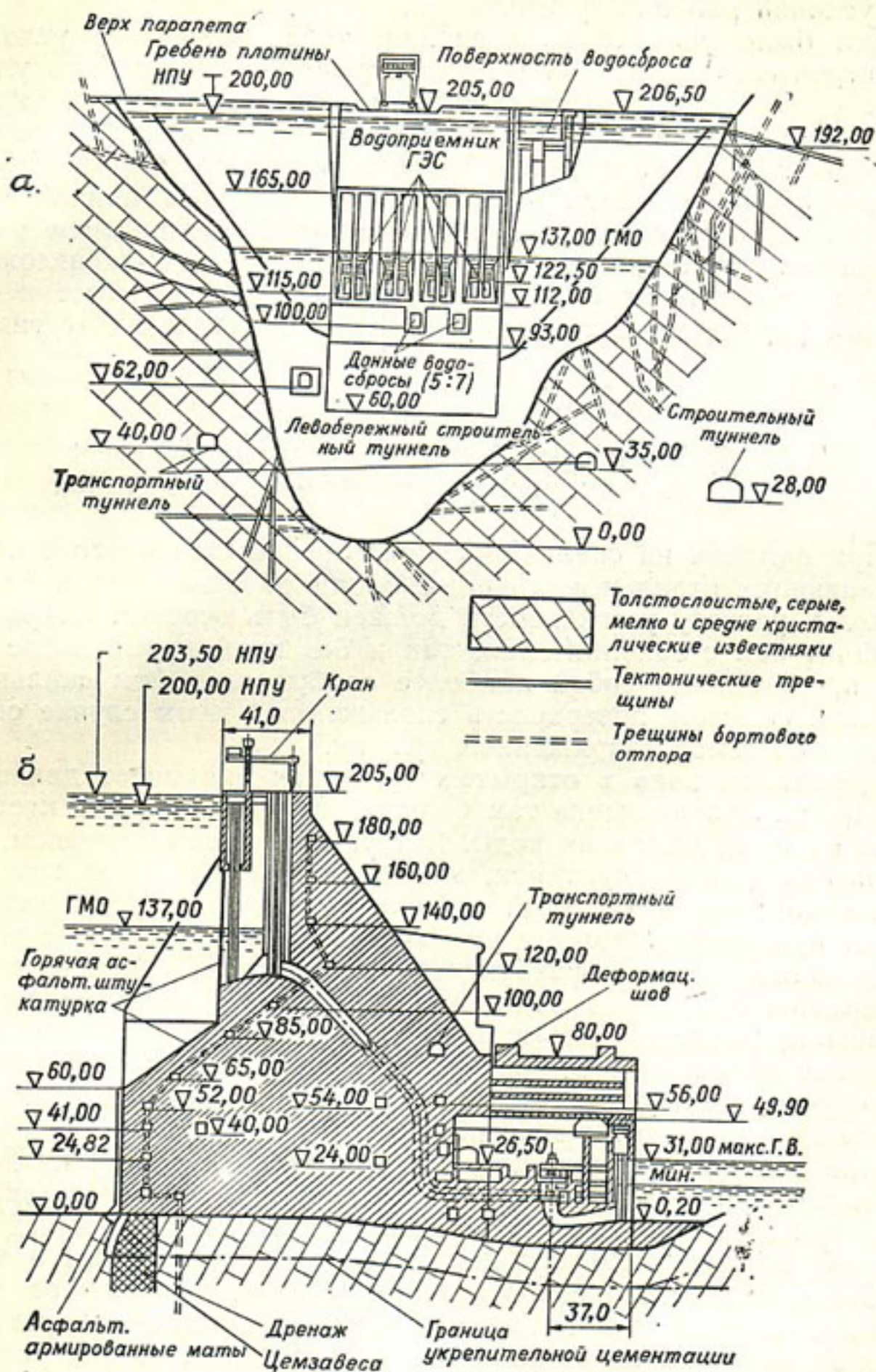
Р и с. 47. Разрезы по Токтогульской плотине.
