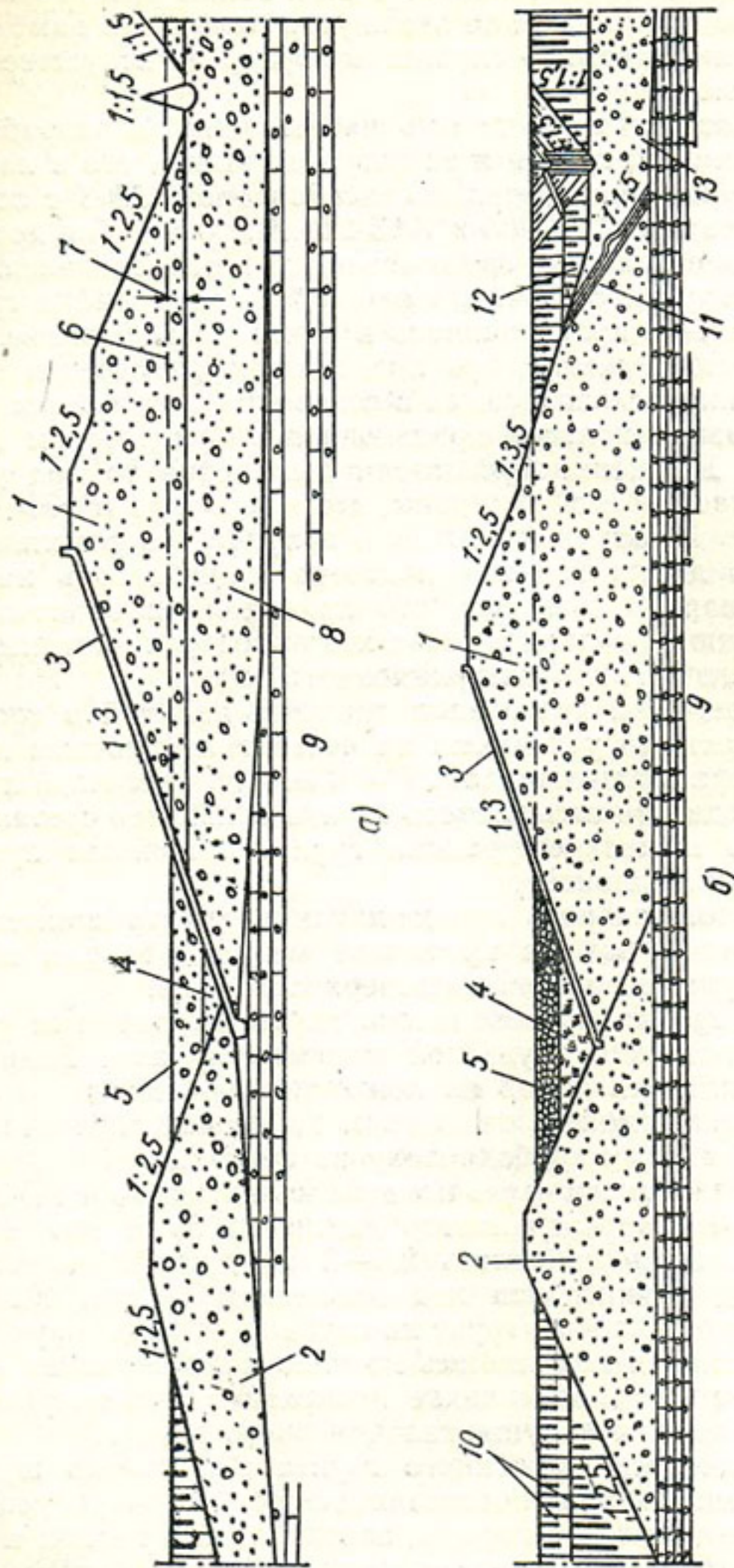
Р и с. 18. Поперечные профили плотины Учкурганской ГЭС.
