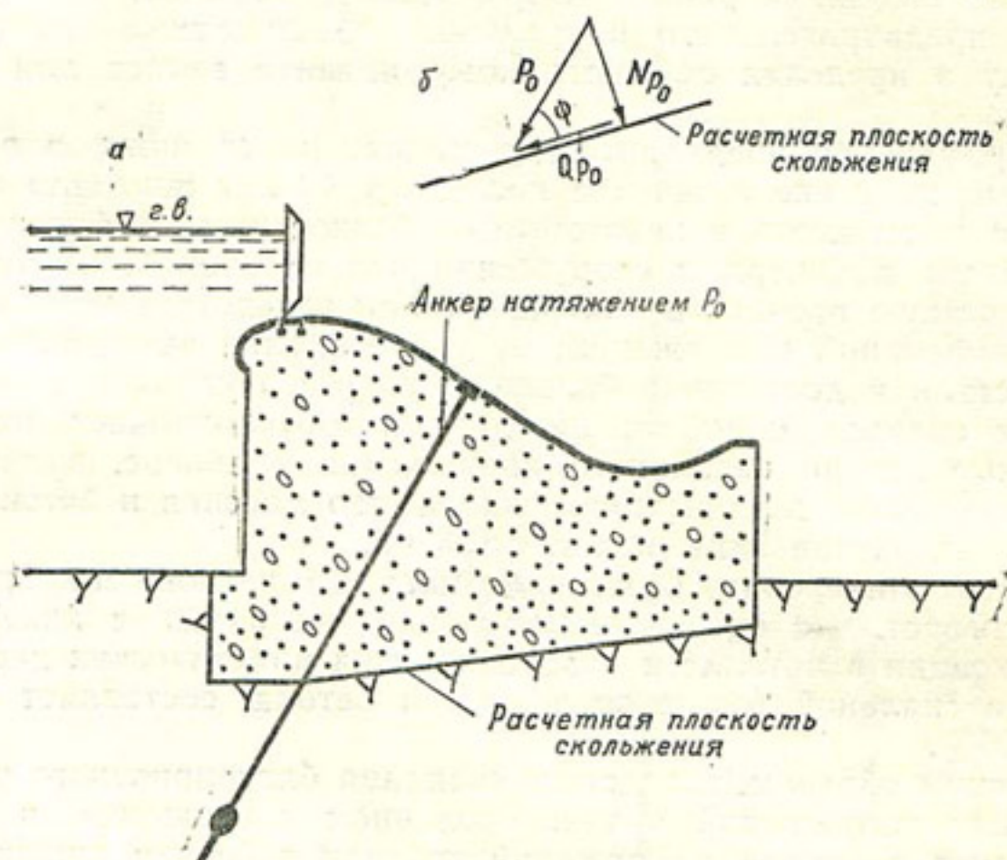
Р и с. 41. Расчет на скольжение заанкерного сооружения. а) Схема заанкереного сооружения, б) Разложение силы натяжения ( P_0 ) на составляющие.
