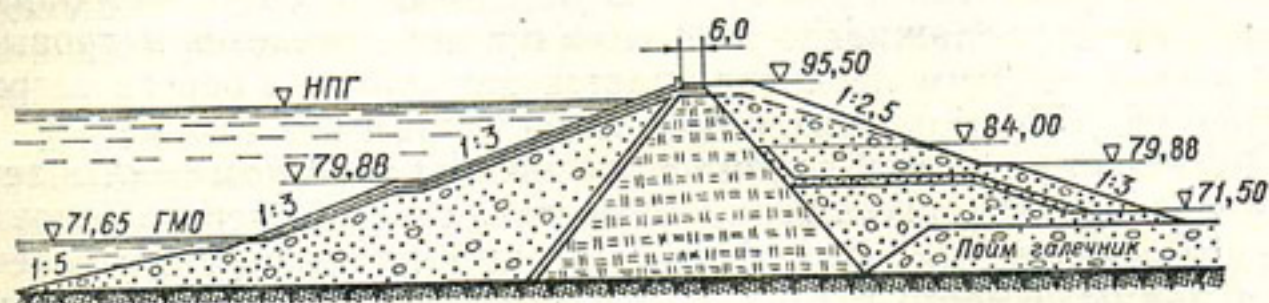
Рис. 15. Поперечный профиль плотины Тюябугузского водохранилища.
