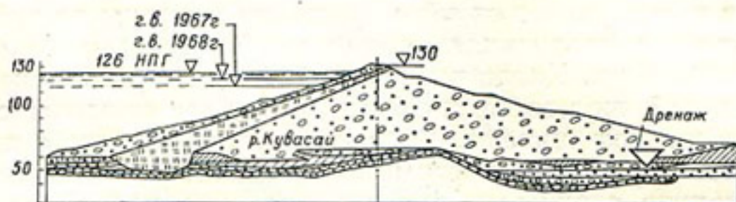
Р и с. 17. Поперечный разрез по плотине Каркиданского водохранилища.
