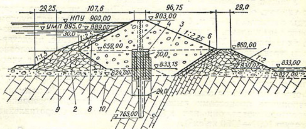
Рис. 22. Поперечный разрез по Атбашинской плотине.
