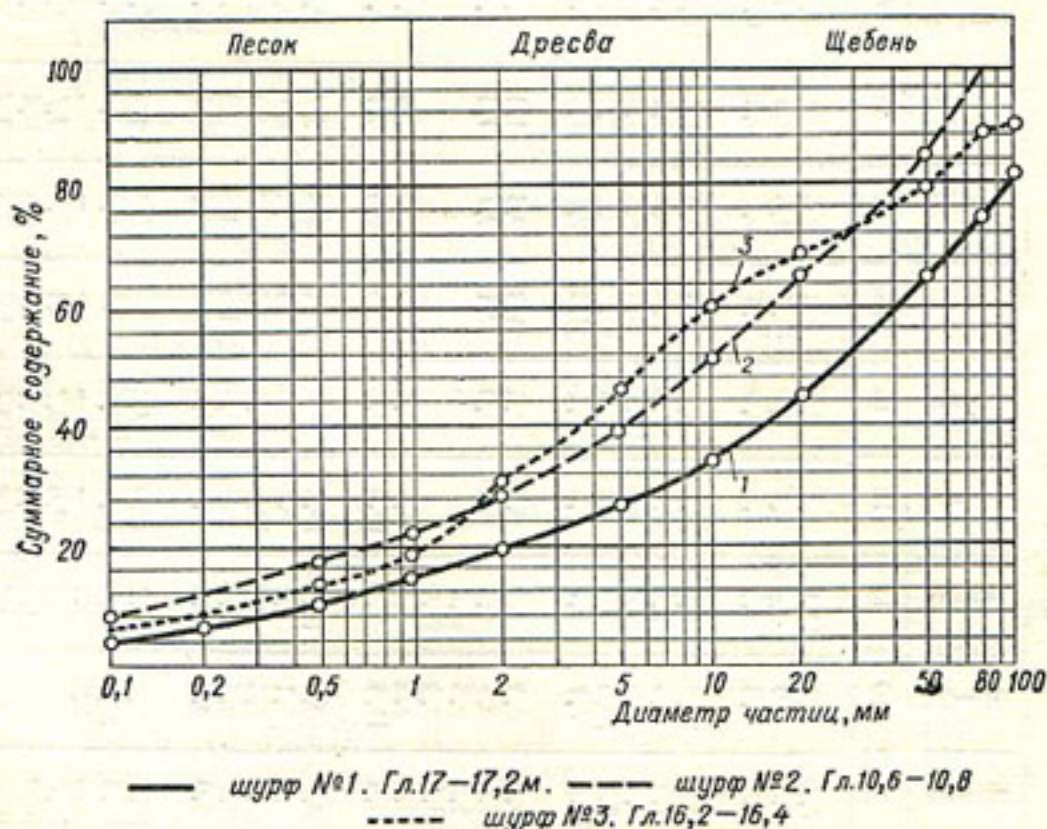
Р и с. 25. График грансостава материала тела плотины Медео.
