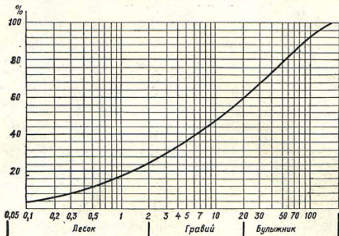
Р и с. 14. Предельная кривая грансостава грунта тела Орто-токойской плотины.
