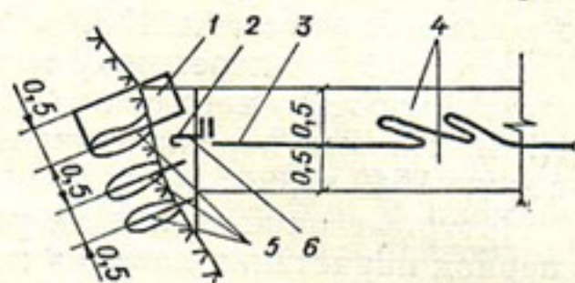
Рис. 21. Примыкание полиэтиленового экрана к скальному борту.
