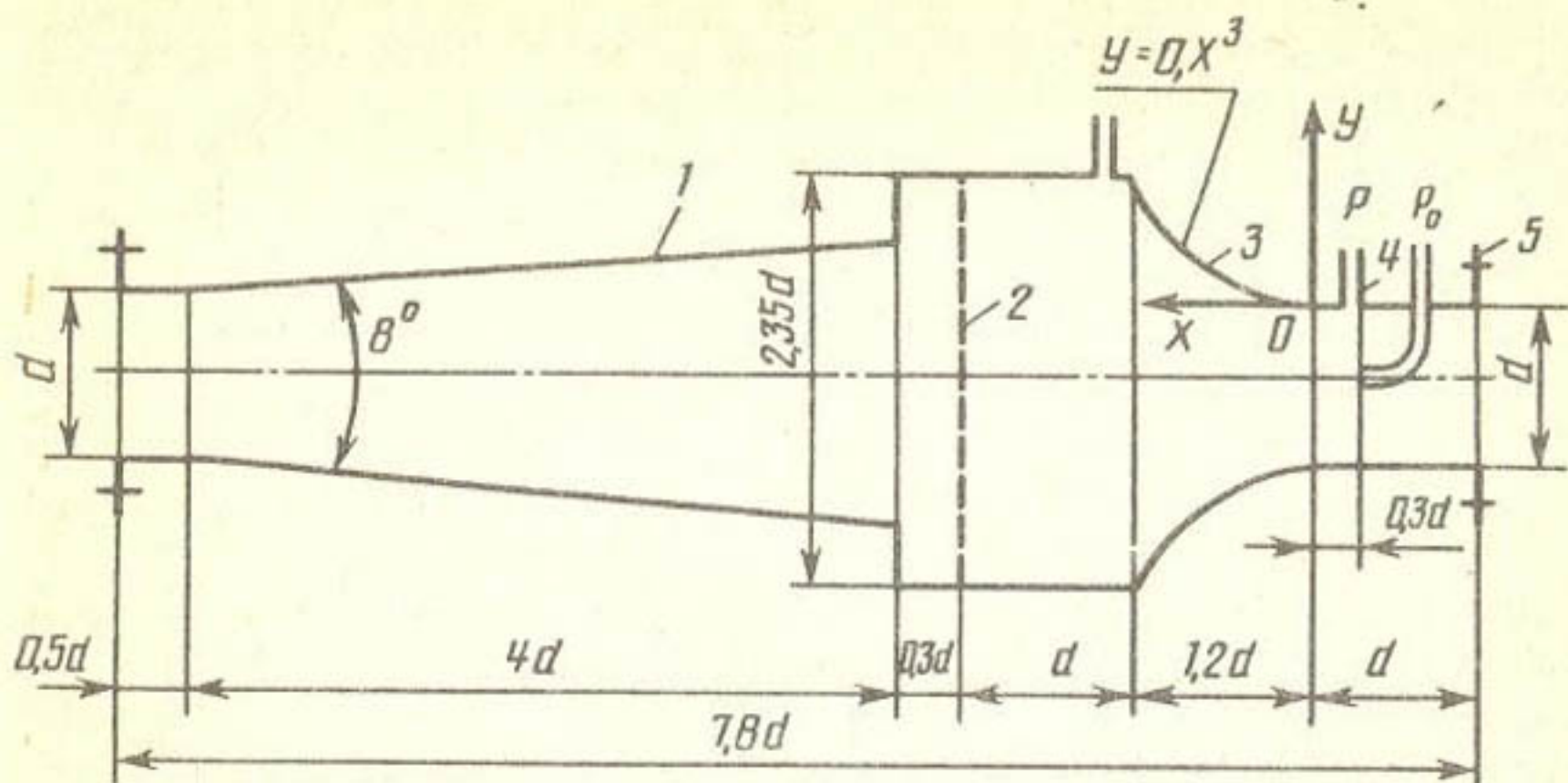
Рис. 3.10. Диффузорный расходомер:
