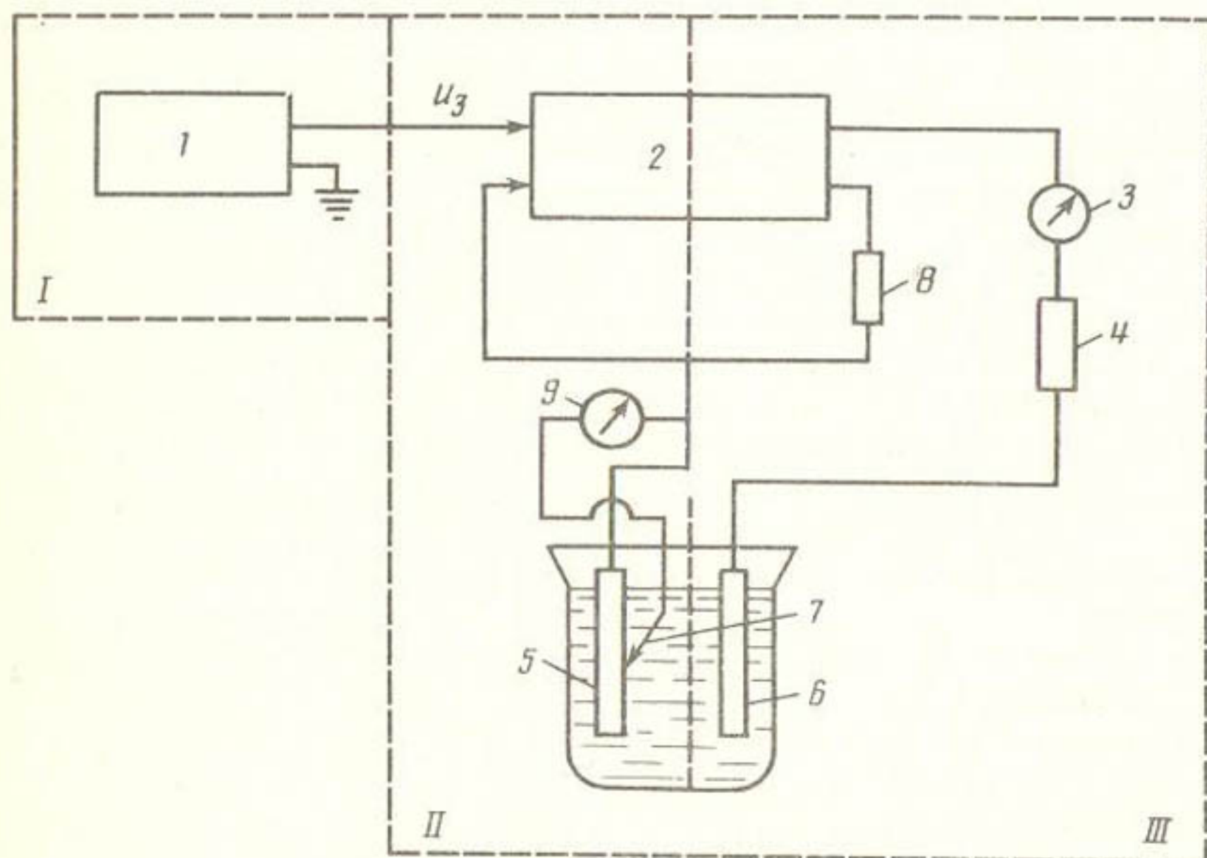
Рис. 2.22. Блок-схема установки для амперостатической кулонометрии:
