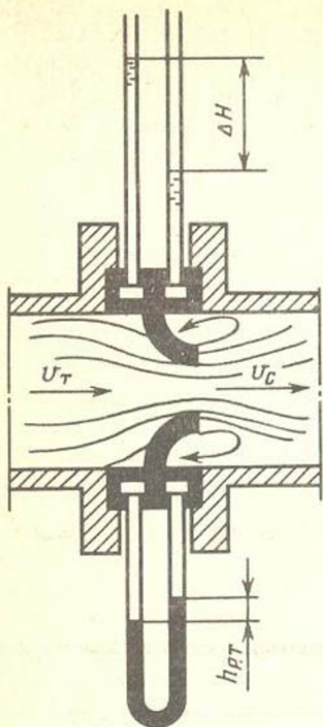
Рис. 3.7. Нормальное сопло
