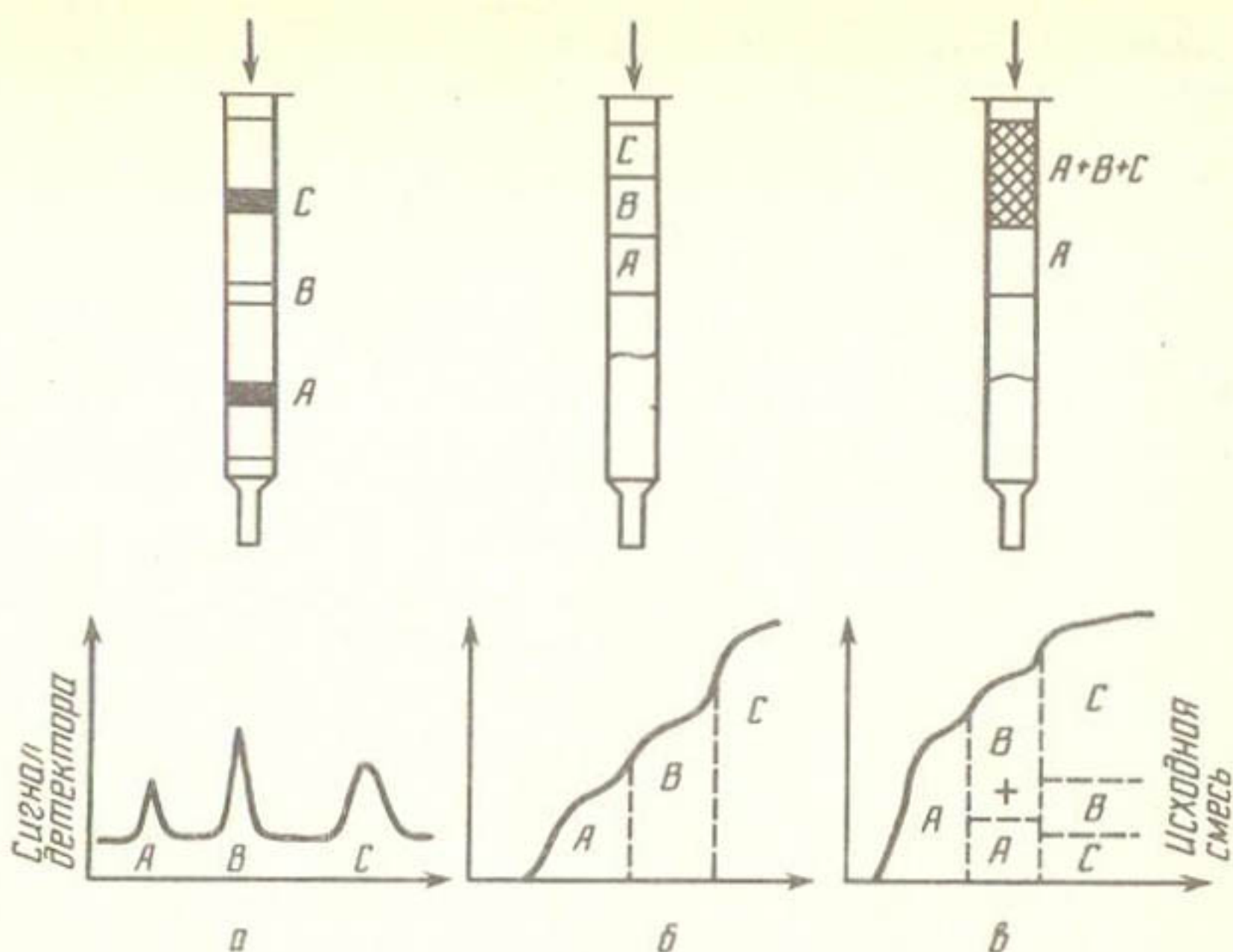
Рис. 2.15. Виды хроматографических методов:
