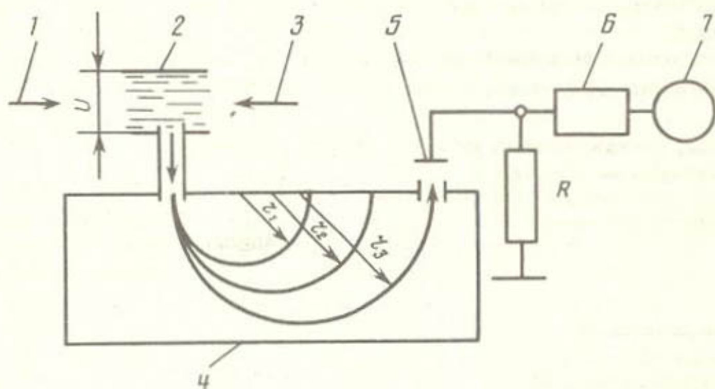
Рис. 2.14. Схема масс-спектрометра:
