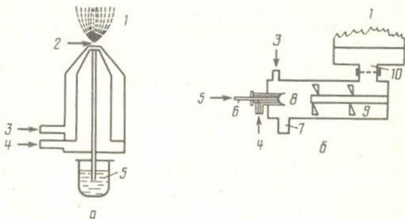
Рис. 2.12. Конструкция распылителей:
