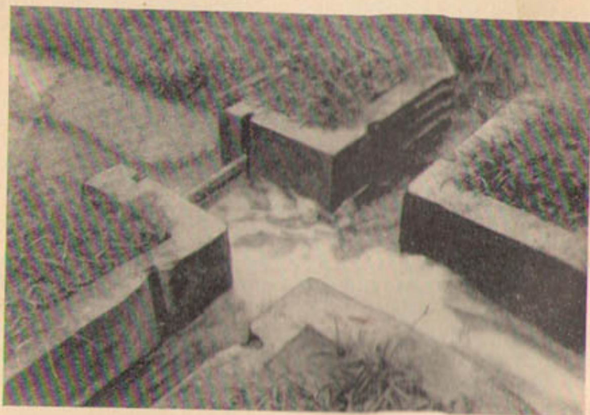
Рис. 95. Бетонный вододелитель с отводом воды в любом из трех направлений.
