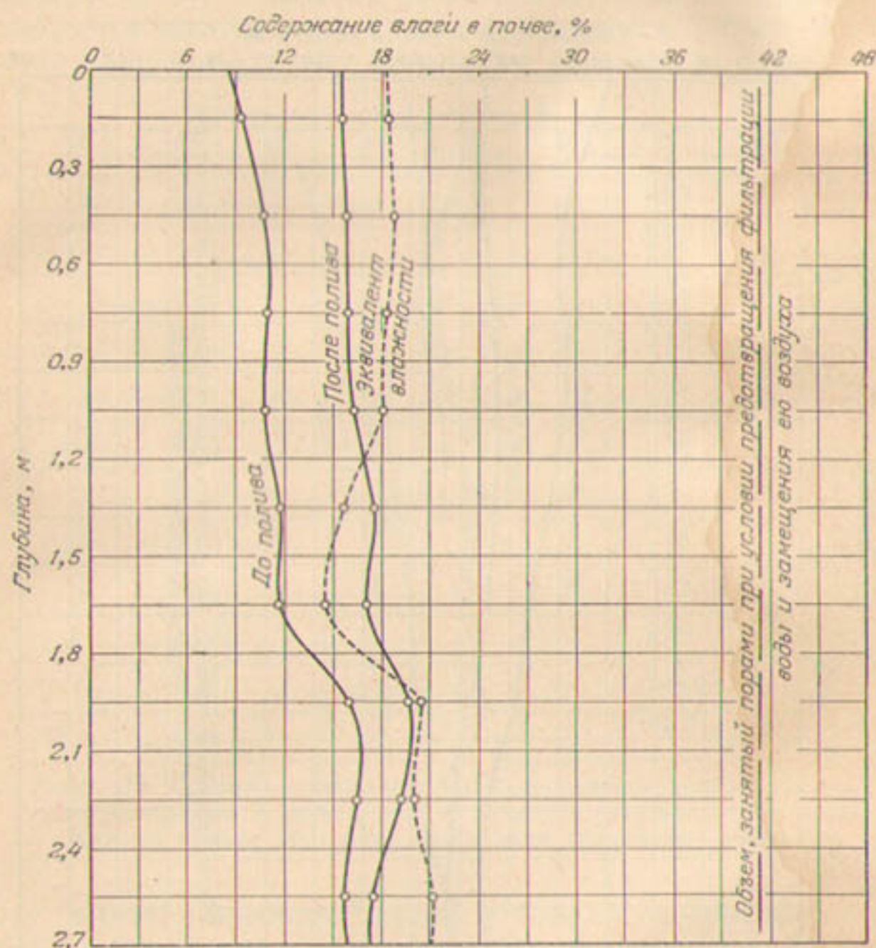
Рис. 113. Графики, показывающие содержание воды в почве до и после полива, эквивалент влажности и объем пор в илесто-суглинистых почвах, подстилаемых тонким песчанистым суглинком. Каждая кривая построена по средним значениям 68 проб.
