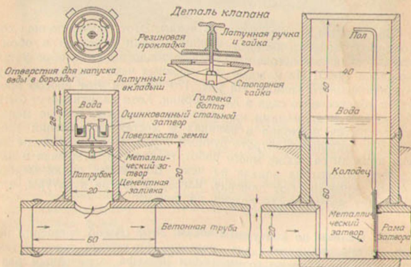
Р и с. 172. Конструкция бетонного трубопровода с вертикальными трубами для орошения фруктовых садов (размеры в см).
