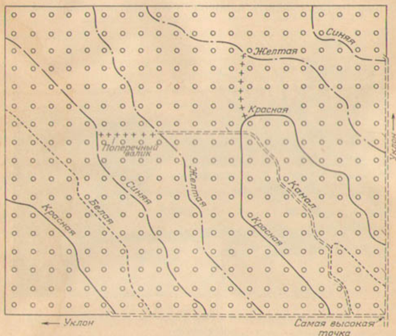
Рис. 174. План поливов фруктового сада затоплением чеканов, расположенных по горизонталям на суглинистой почве, с расходом воды 3,4 \text{ м}^3/\text{мин} . На одной площадке посажено не более 40 деревьев. Горизонтали рельефа отмечены на деревьях разным цветом — красным, белым, синим и желтым.
