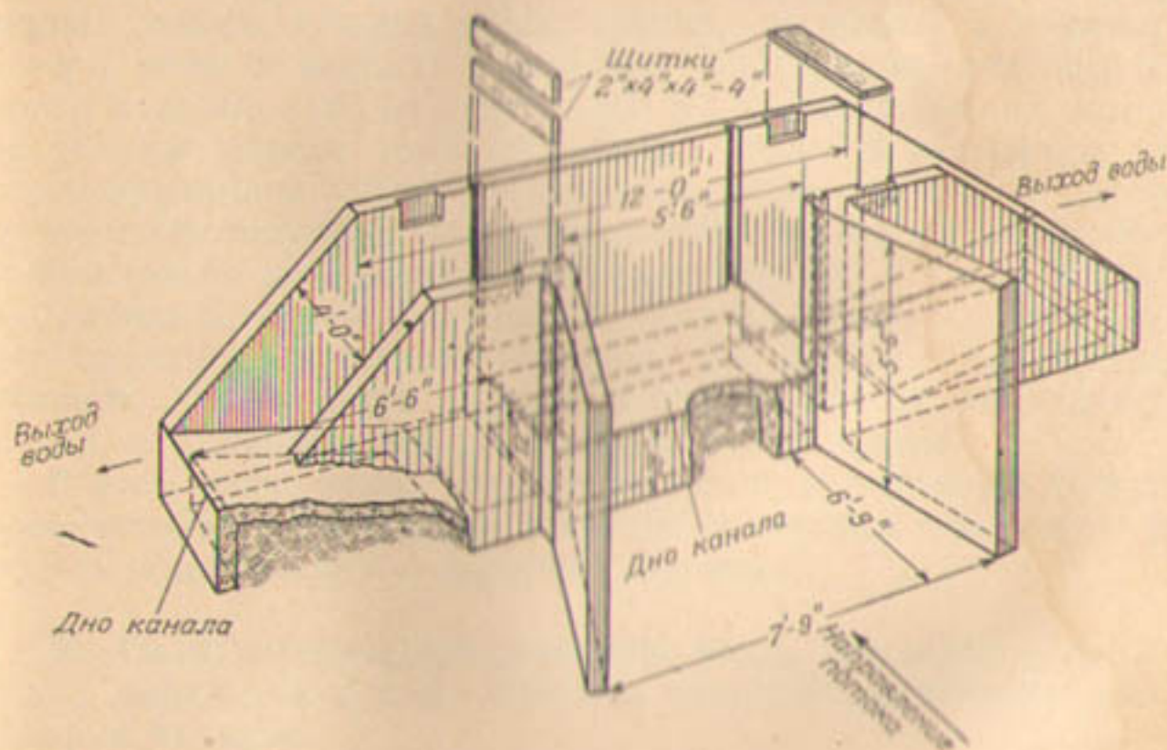
Рис. 28. Бетонный ящик-вододелитель.
