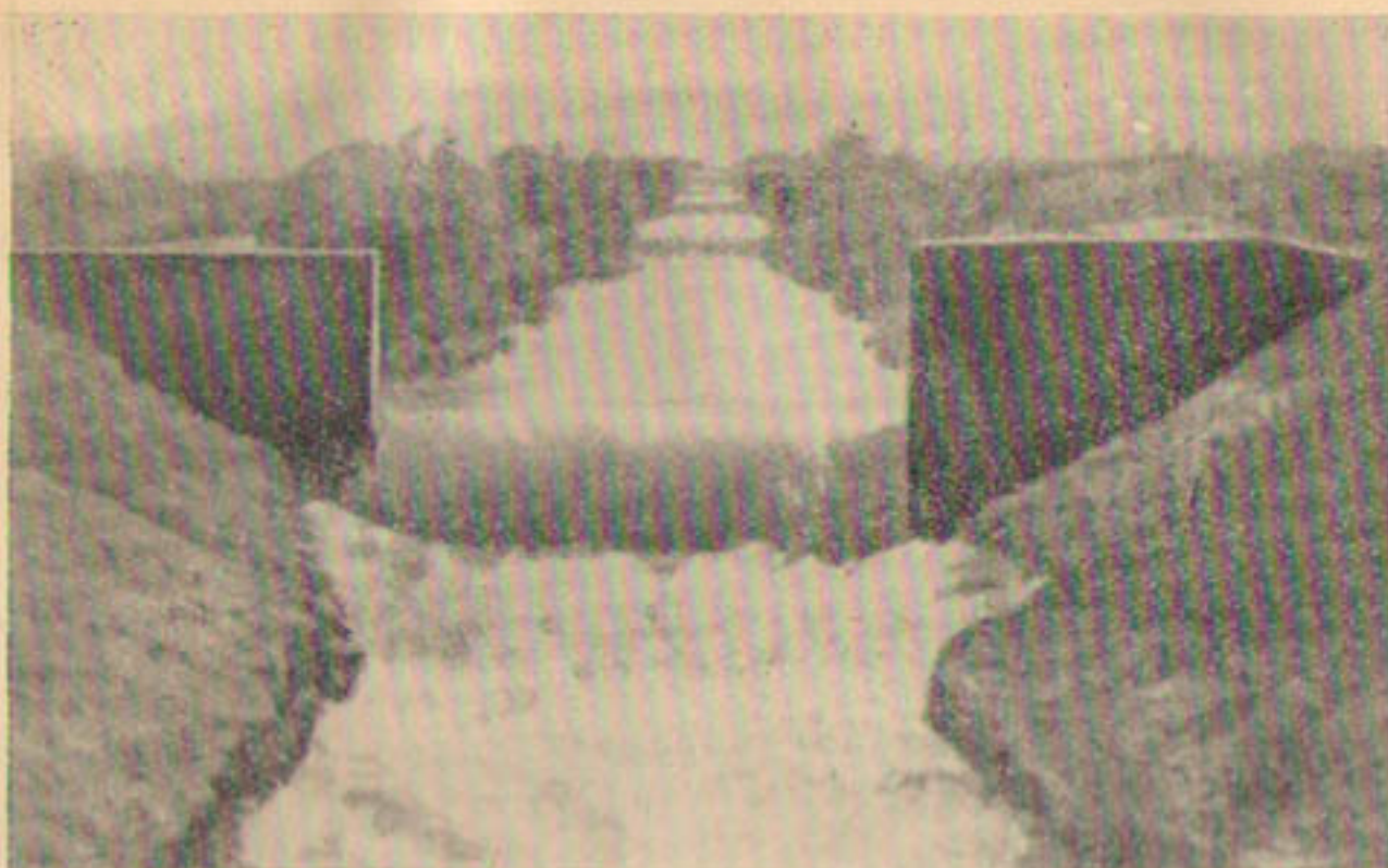
Р и с. 45. Ряд последовательно расположенных перепадов для уменьшения скорости течения и предупреждения размыва. Для поднятия уровня воды в канале могут быть установлены узкие щиты, скользящие в пазах. Благодаря этому можно производить полив полей по обеим сторонам канала.
