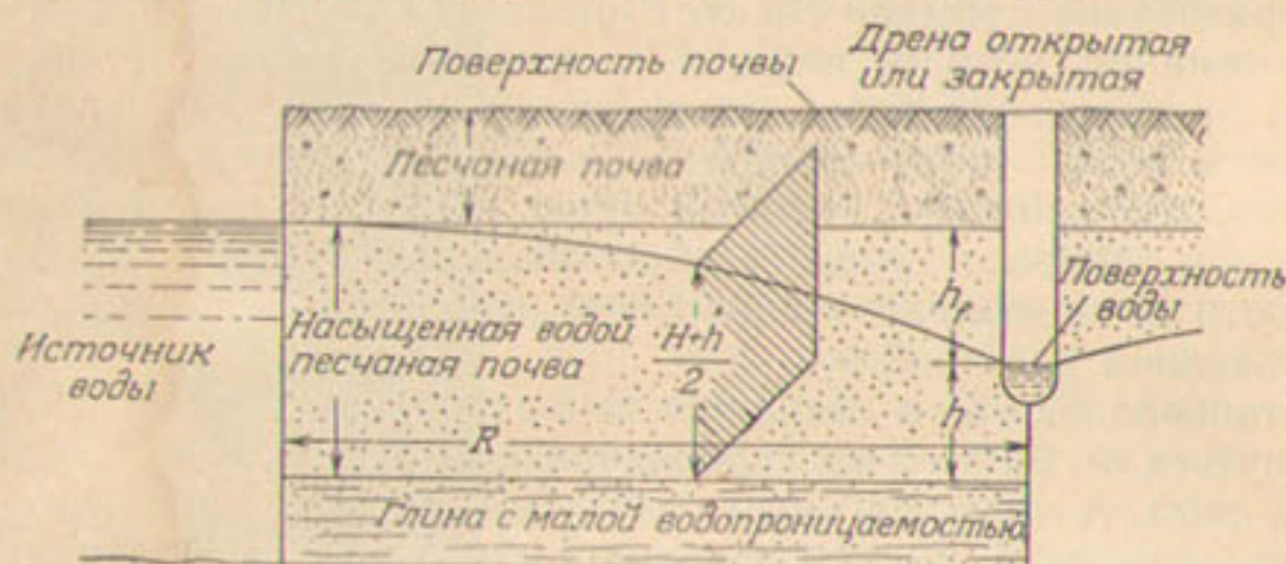
Рис. 150. Схема прямолинейных токов грунтовых вод в направлении к дренам с расстоянием между ними 2R . Уровень грунтовых вод находится на H-h выше горизонта воды в дренах, проложенных в песчаной почве, подстилаемой глиной.
