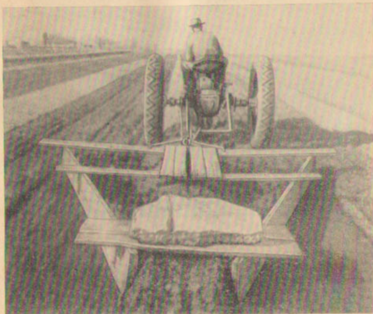
Р и с. 87. Устройство валиков, ограничивающих поливные полосы.
