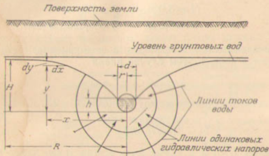
Рис. 151. Схема радиальных токов грунтовых вод в направлении к дренам, прорытым в однородной почве. Уровень грунтовых вод расположен на (H - h) м выше горизонта воды в дренах.
