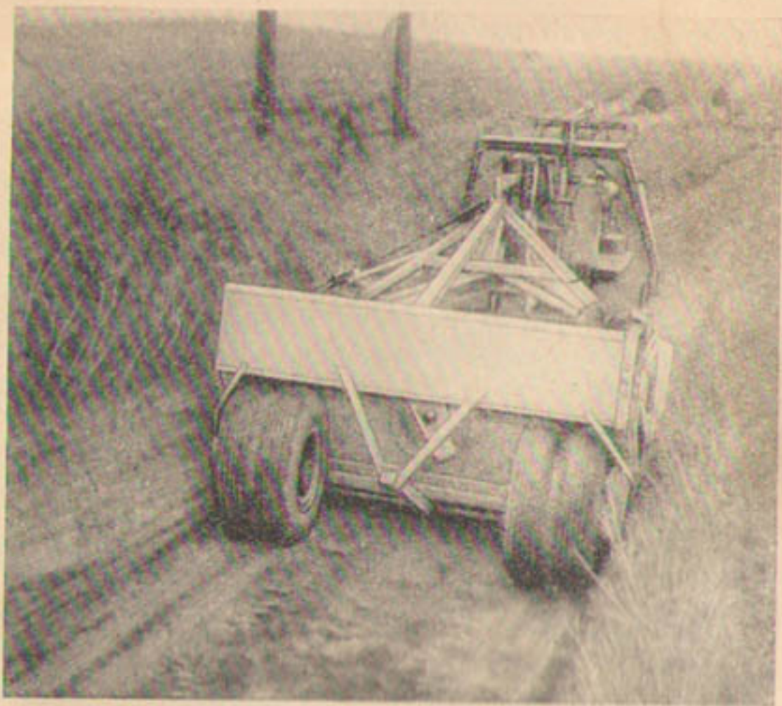
Р и с. 89. Скрепер на тяге гусеничного трактора. Применяется для рытья каналов с крутыми откосами с перемещением грунта на большие расстояния.
