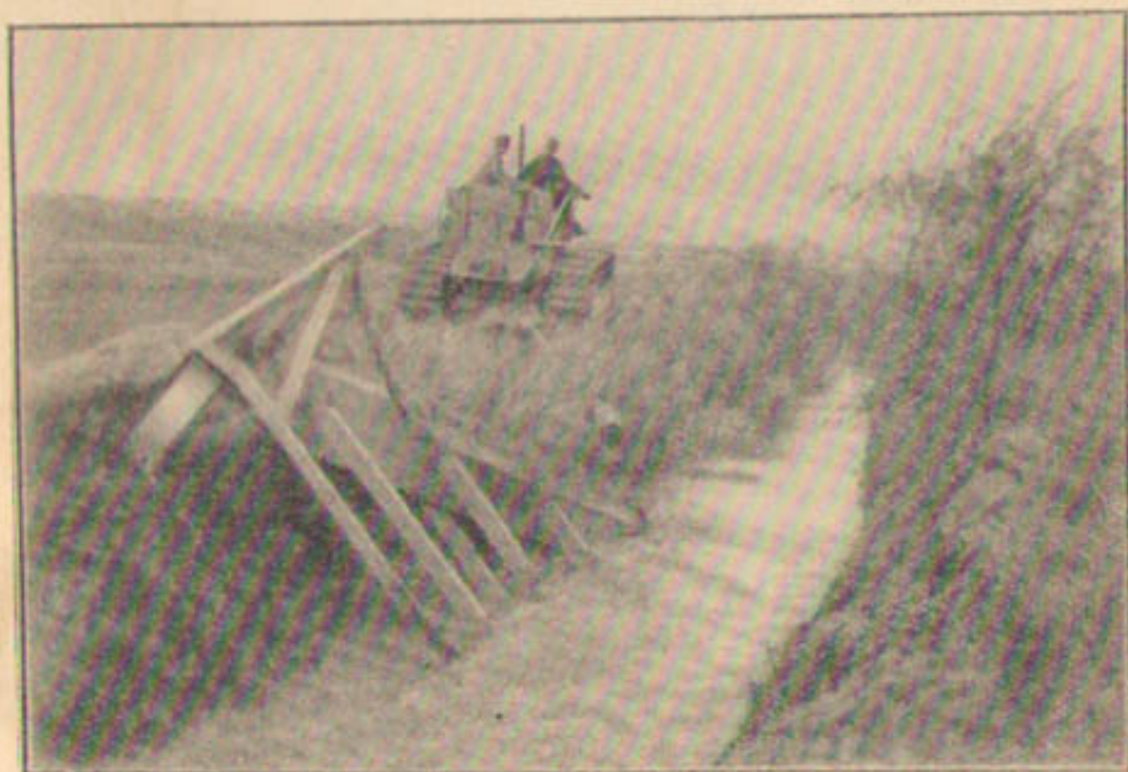
Р и с. 91. Механизм для очистки откосов каналов с длиной ножа 55 см, весом 3,2 т. Очищает канал глубиной 1,5 м с крутыми откосами.
