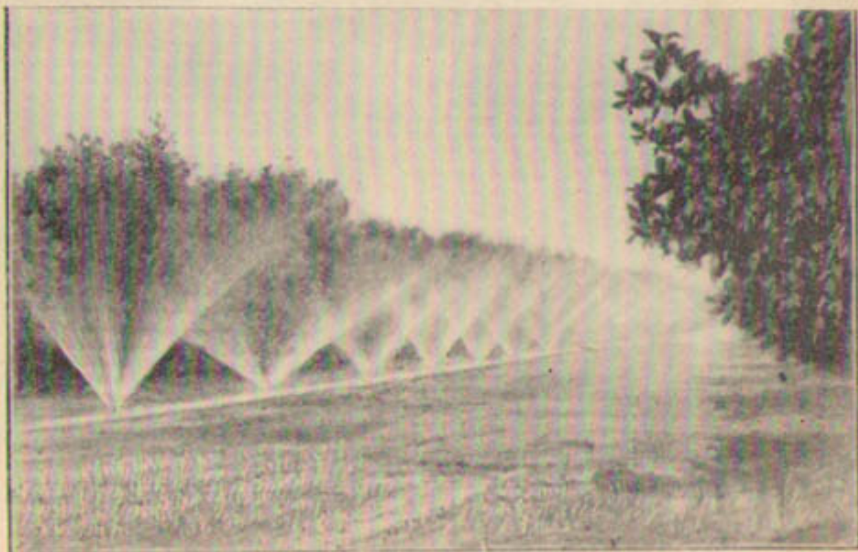
Рис. 169. Переносный трубопровод с неподвижными насадками с круговым разбрызгиванием для орошения citrusового сада.
