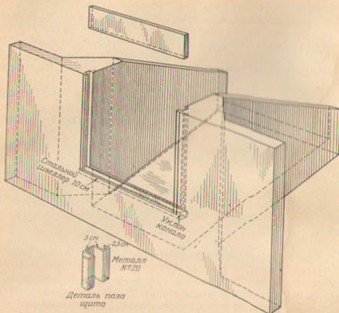
Рис. 94. Бетонный регулятор с деревянным узким щитом.
