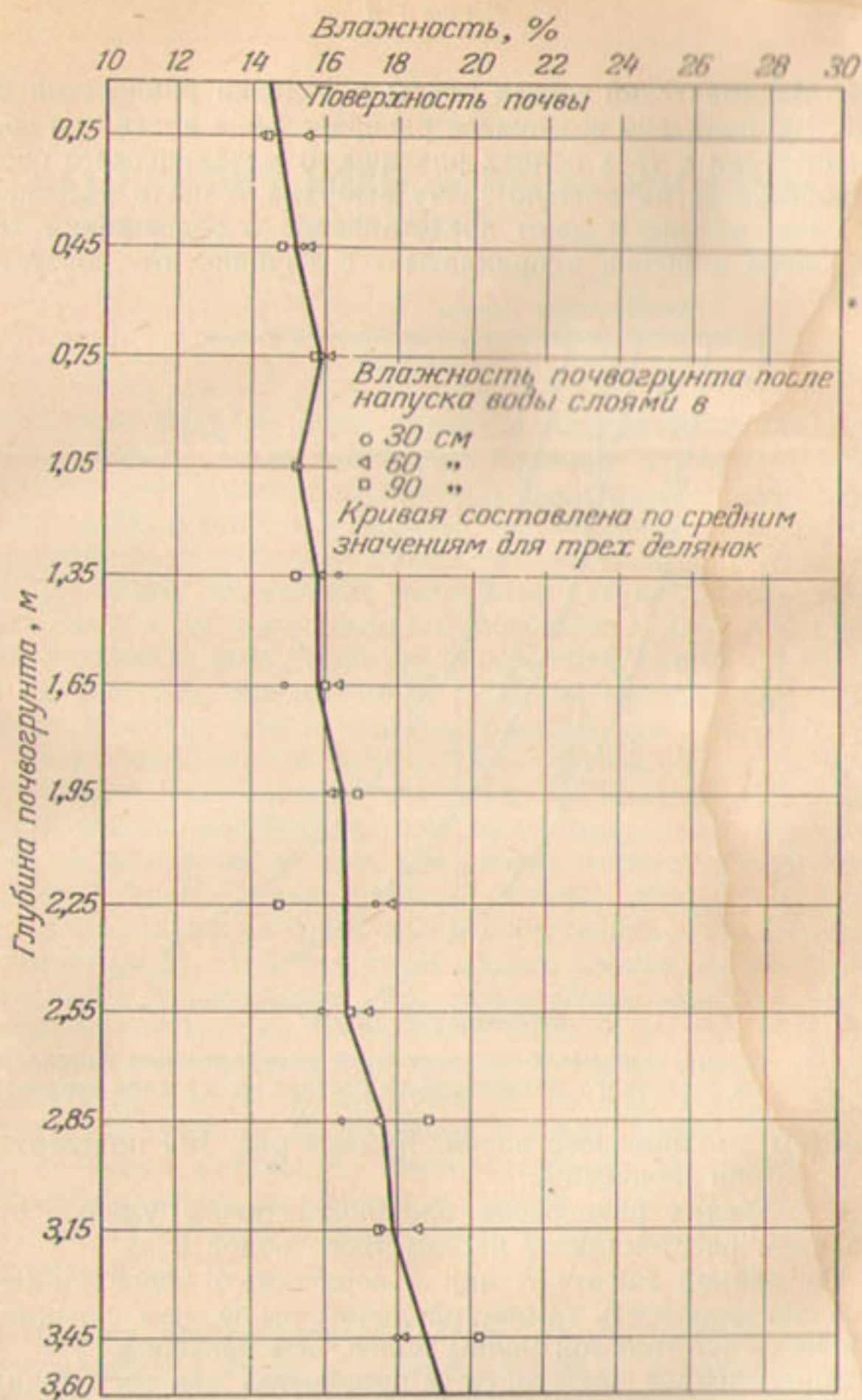
Рис. 108. График распределения влажности в почвогрунте через 68 дней после полива с поправками на разнообразие механического состава почвогрунта, что дает представление о распределении, которое могло бы быть в почве с однородным механическим составом.
