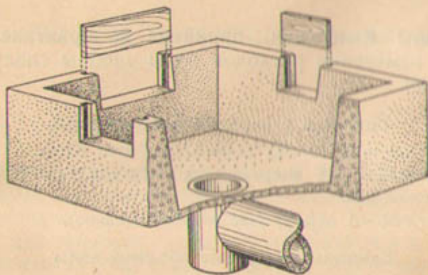
Рис. 27. Водосливной ящик для пропорционального деления воды.
