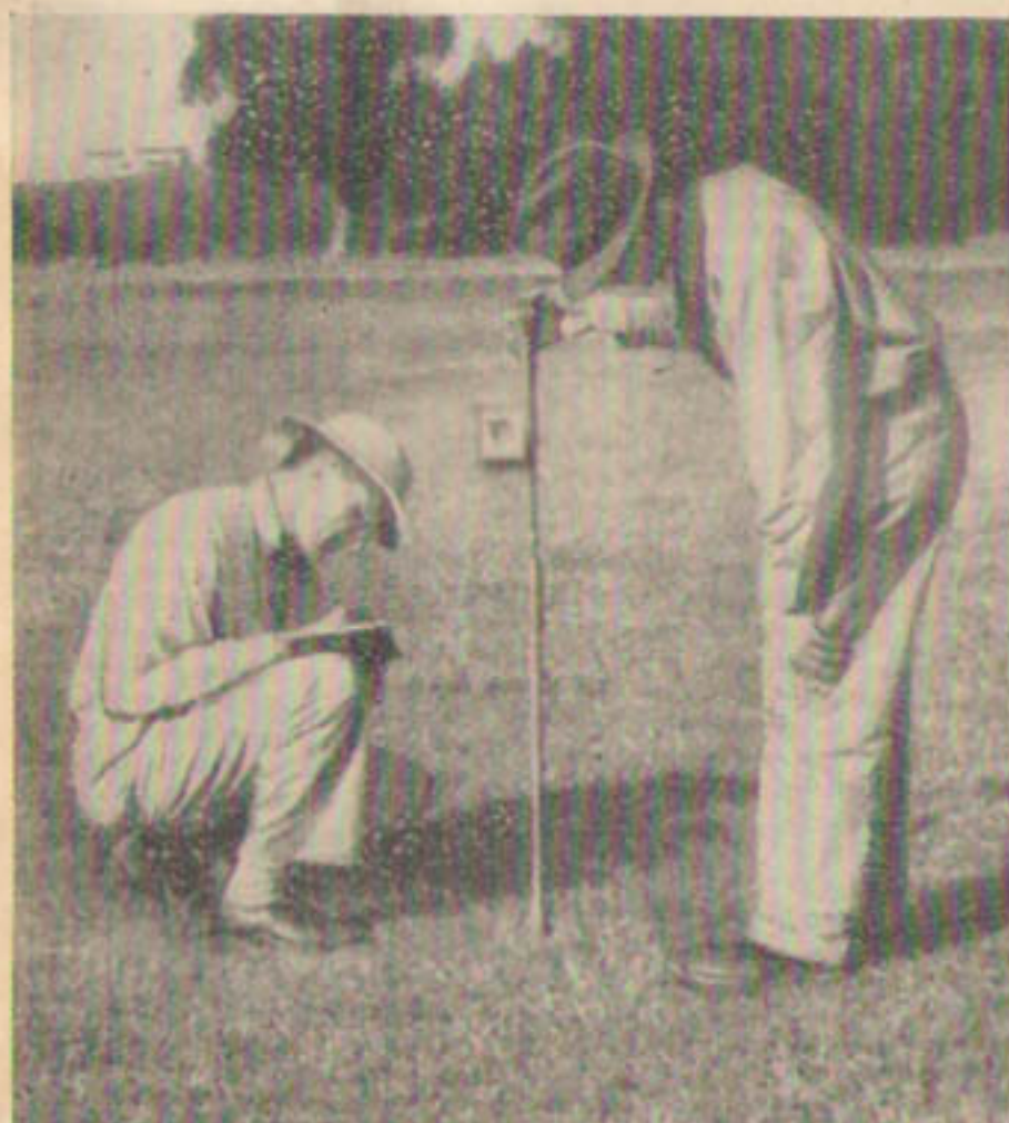
Р и с. 131. Измерение напора пьезометром при помощи электрического звукового аппарата.
