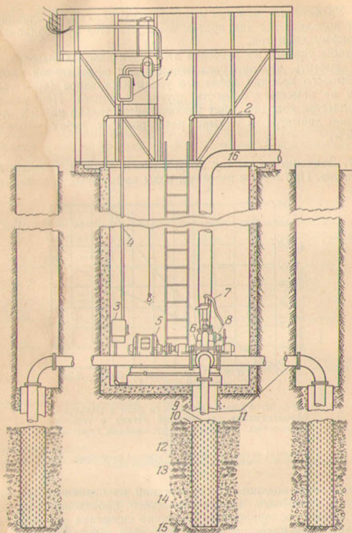
Р и с. 64. Горизонтальный центробежный насос, установленный в шахте и непосредственно соединенный с электродвигателем; насос выкачивает воду одновременно из трех колодцев.
