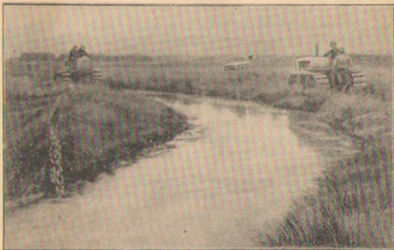
Рис. 34. Дизельные тракторы тянут большую цепь весом 1040 кг, при помощи которой дно канала очищается от мха и сорной растительности.
