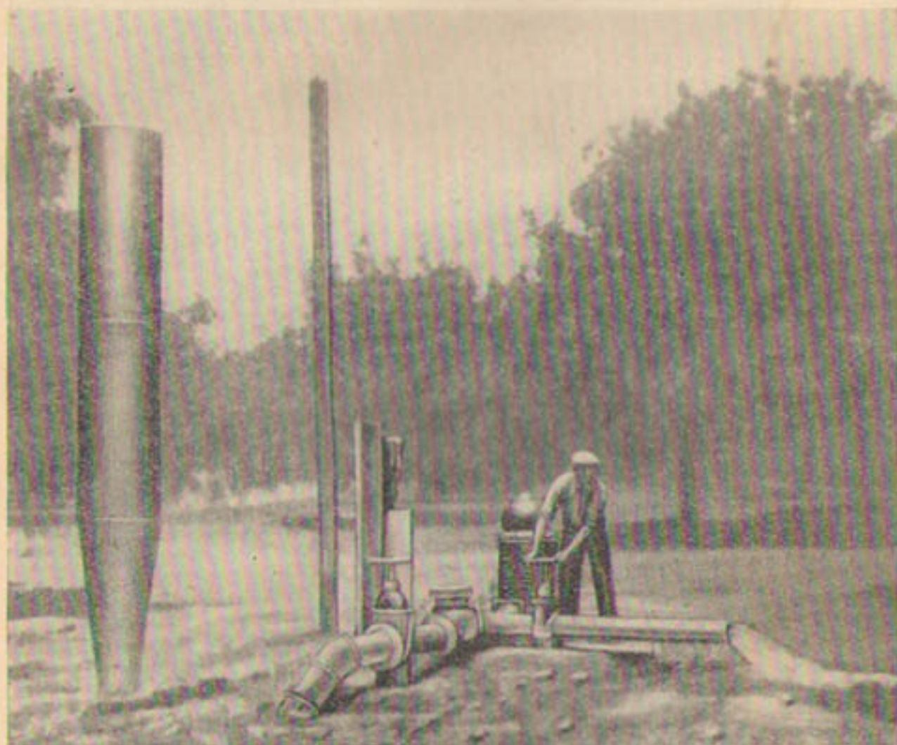
Р и с. 65. Насосная установка в саду. Глубина колодца 170 м.
