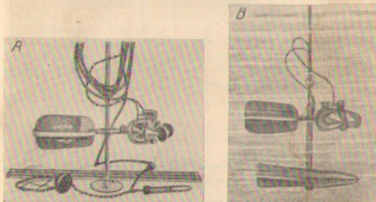
Рис. 24. А — гидрометрическая вертушка системы Лейц, подвешенная на стержне с круглым опорным диском; В — гидрометрическая вертушка системы Герли в работе.
