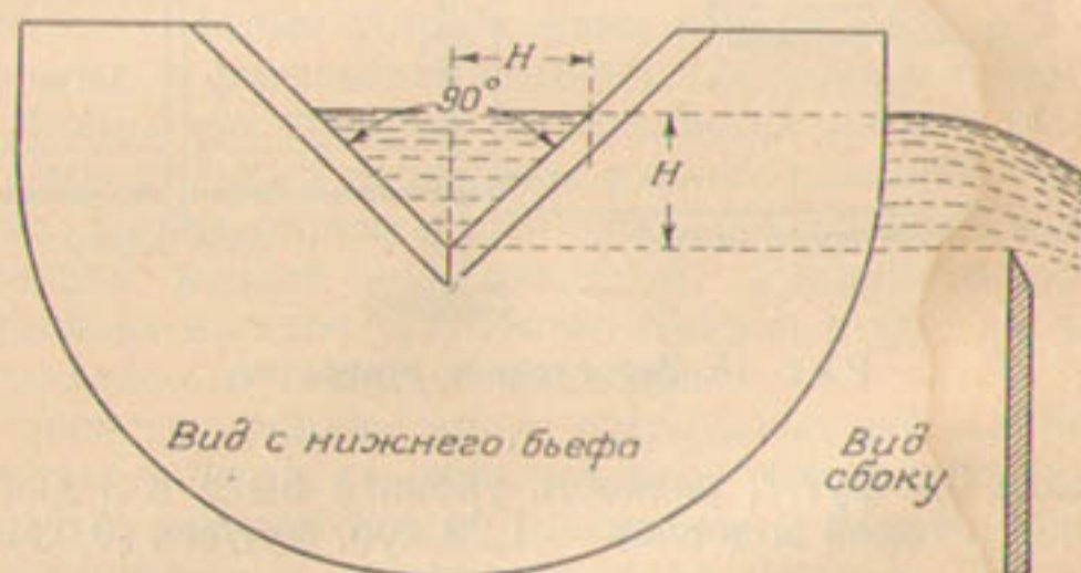
Р и с. 15. Треугольный водослив с углом выреза 90°.
