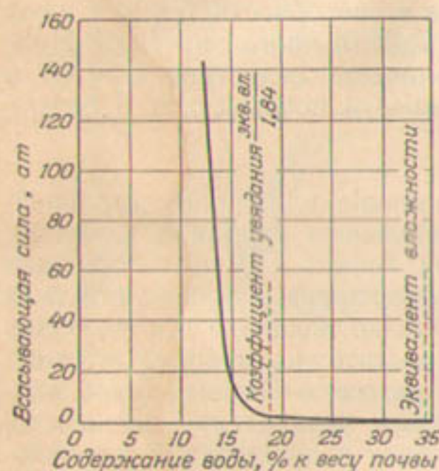
Рис. 153. Кривая всасывающей силы, удерживающей воду в илесто-глинистом суглинке при разных величинах влажности.
