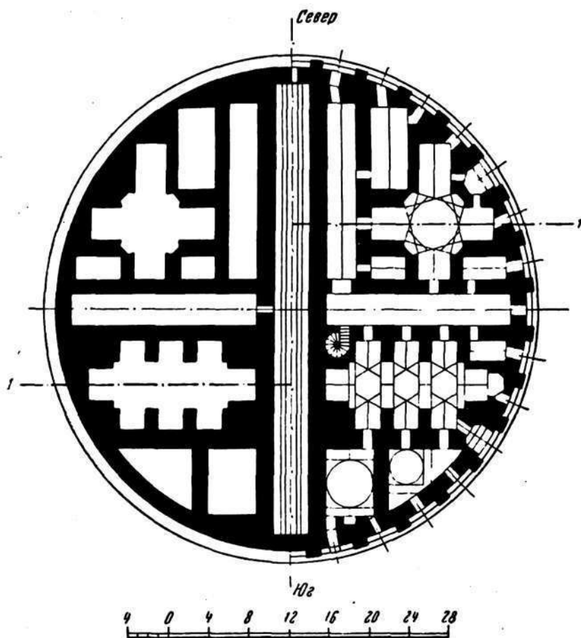
Рис. 43. Обсерватория Улугбека. План.
