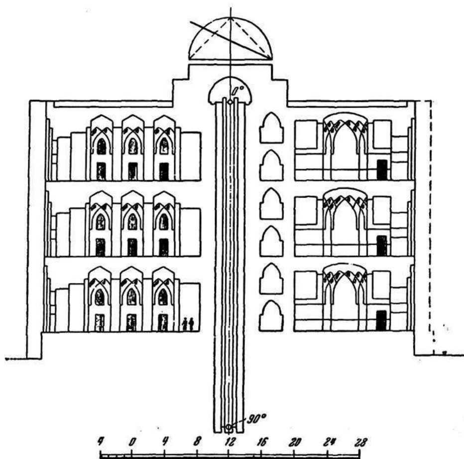
Рис. 45. Обсерватория Улугбека. Разрез 1—1.
