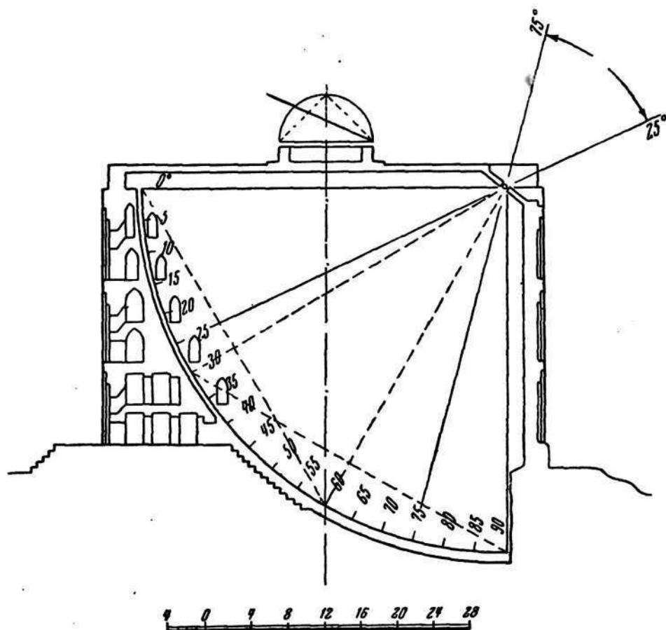
Рис. 44. Обсерватория Улутбека. Разрез север — юг.
