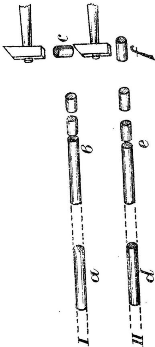
Габл 62. Техника изготовления монетных кружков.
