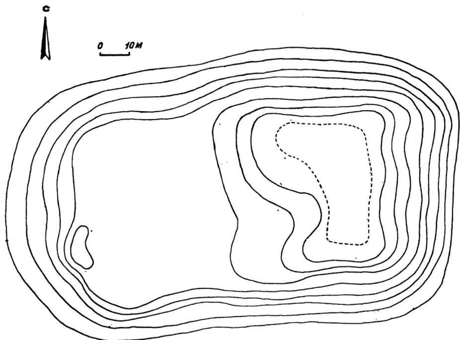
Рис. 9. Поселение Дарахша-тепе. План-схема (сечение горизонталей 1 м).
