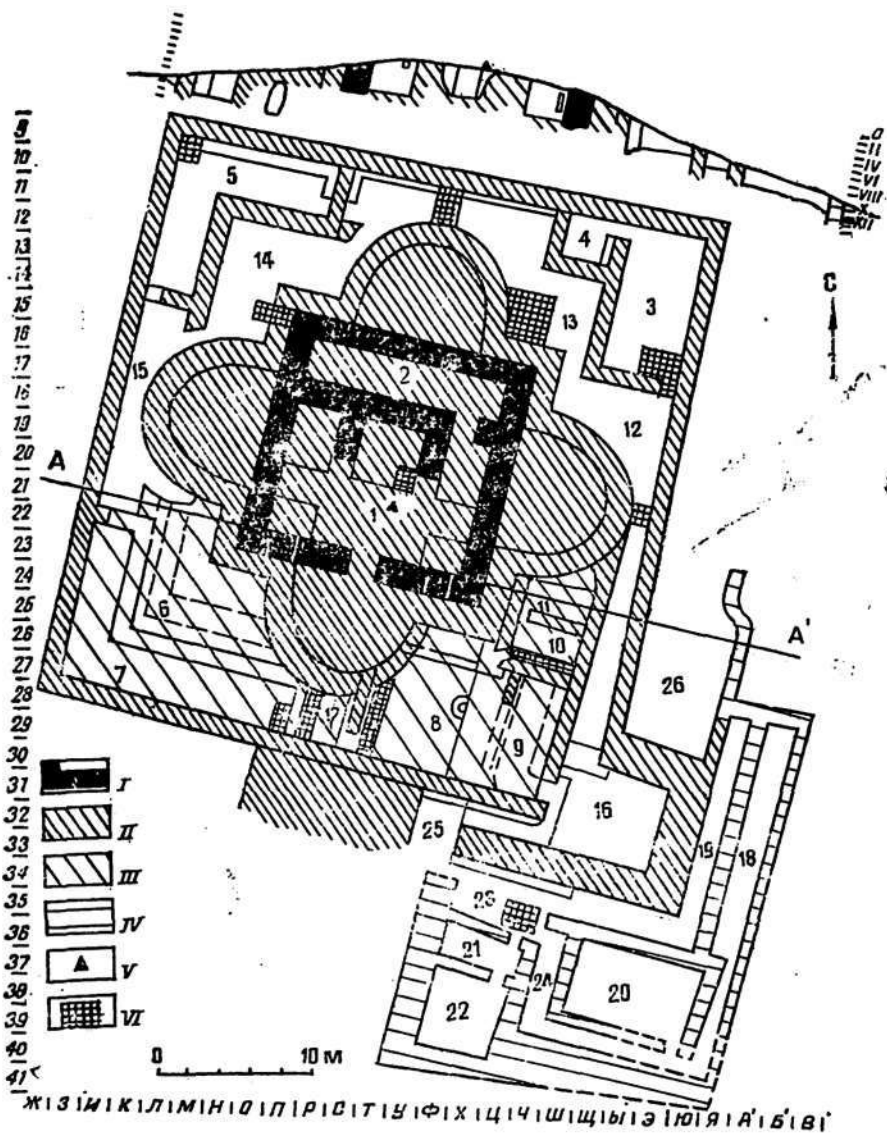
Рис. 22. Сеталак-II. Общий план и поперечный профиль по линии А—А 1 :
