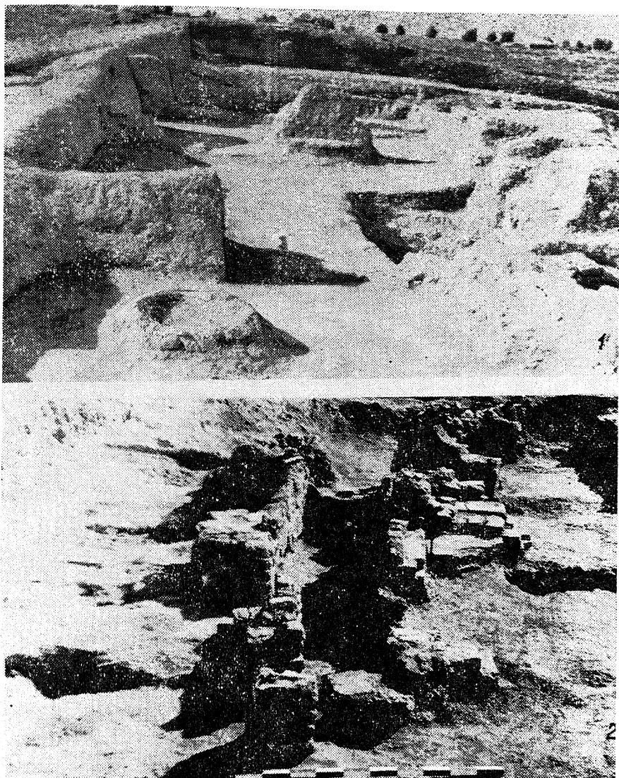
Рис. 58. Баня XI—XII вв. на городище Отрар: 1 — интерьер одного из помещений; 2 — остатки обогrevательной системы
