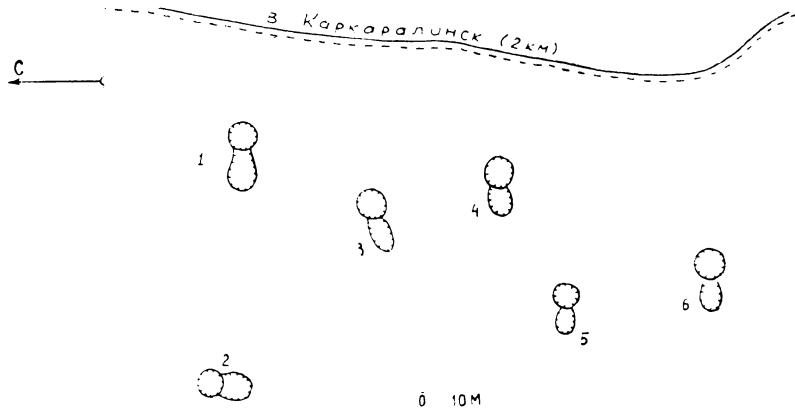
Рис. 3. План рудоплавильных печей из окрестностей Каркаралинска.
