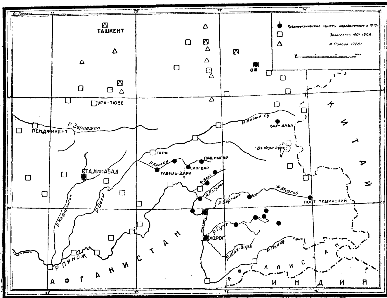
Рис. 2. Гравиметрические пункты Таджикистана.
