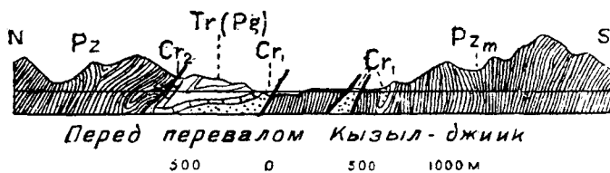
Рис. 4. Геологические разрезы.
