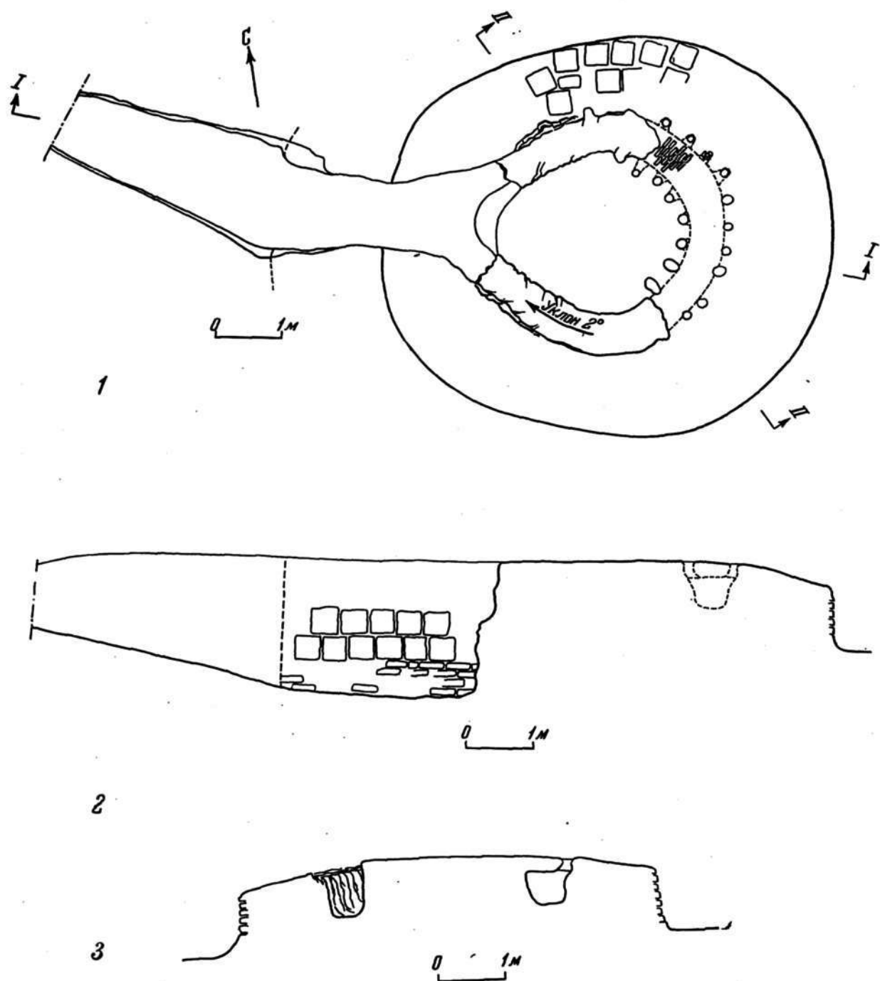
Рис. 54. Керамическая обжигательная печь VII—VIII вв. у Большой Кырк-кыз-калы 1 — план, 2 — разрез I—I, 3 — разрез II—II
