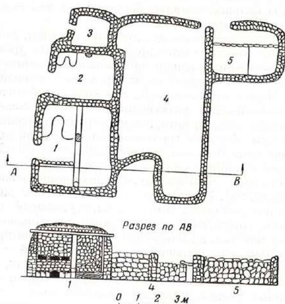
Рис. 24. План и разрез летовки «иль» в Хвауне:
