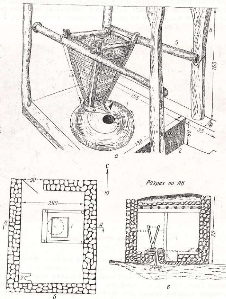
Рис. 11. Водяная мельница «хаёрт»:
