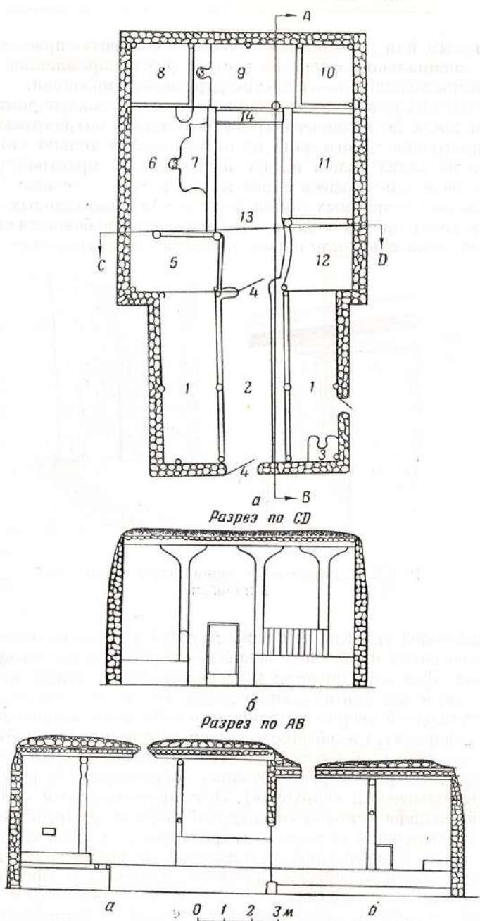
Рис. 28. План дома Худояр-бека, киил. Андербак:
