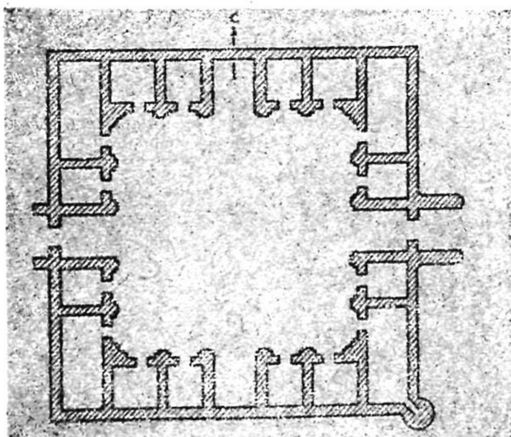
10. Оде-Мергень-кала. План.
