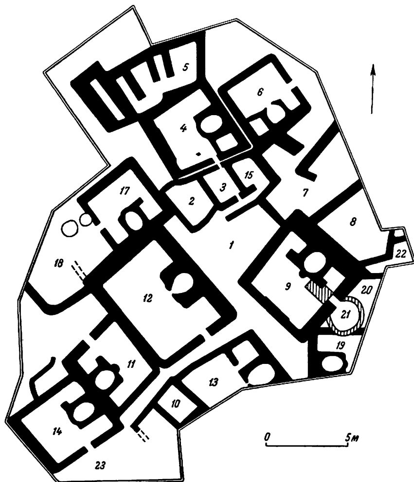
Рис. 11. План строений, вскрытых на Чагыллы-Депе на уровне третьего строительного горизонта.
