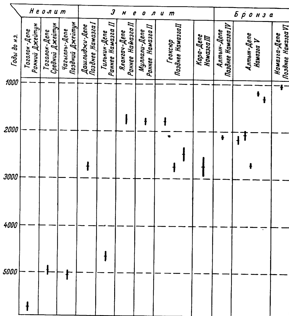
Рис. 15. Радиокарбонная хронология раннеземледельческих поселений Южного Туркменистана.
