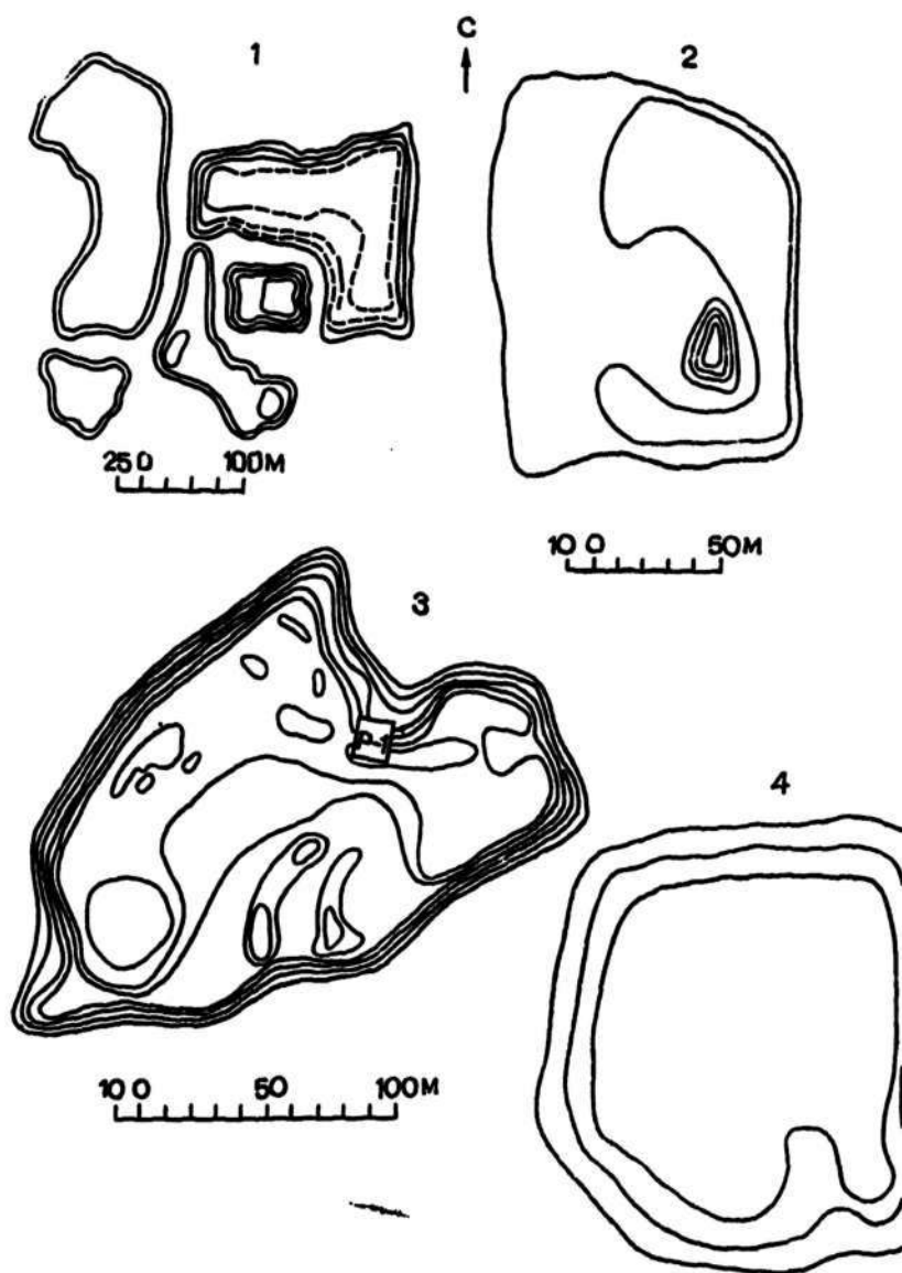
Рис. 6. Планы поселений Сарыктепе (съемка А. С. Сагдуллаева) (1), Кяндыктепе (съемка Г. Я. Дресвянской) (2), Ялпактепе (3), Бахрынтепе (4).
