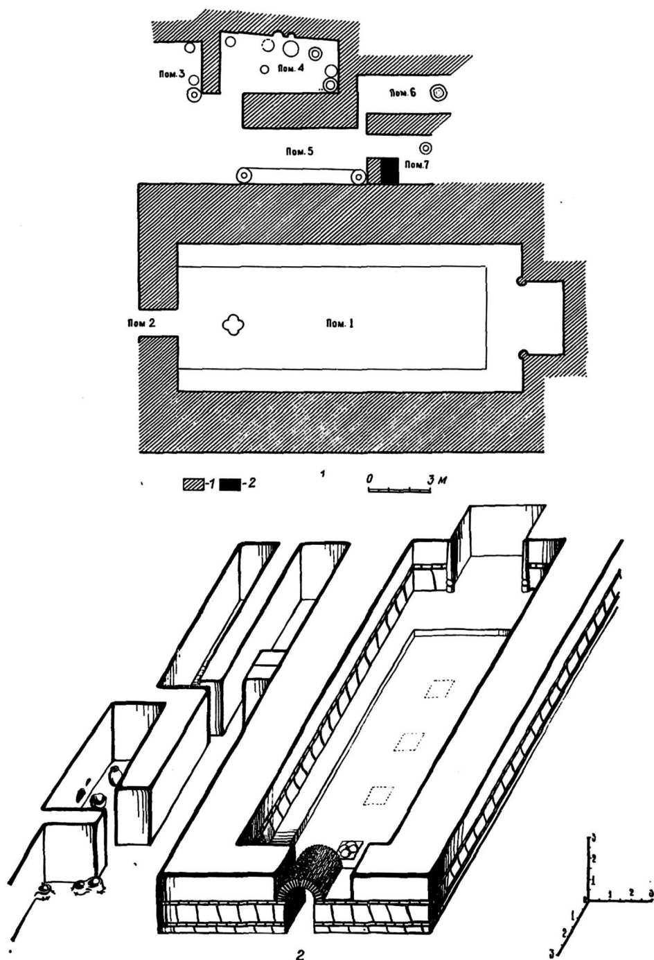
Рис. 5. Кафыркала. Жилой дом в городе: 1 — план: (1) — основные стены; (2) — ремонтные стены; 2 — аксонометрия
