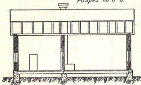
Разрез по Б-Б
