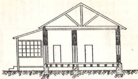
Разрез по А-А
