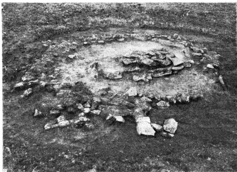
Рис. 8. Могильник Тасты-бутак 1
