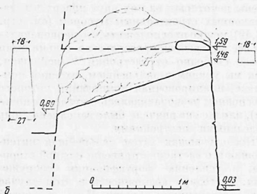
Рис. 122. Бойницы во внутренней стене стрелковой галереи внешнего кольца (у башни № 5):
