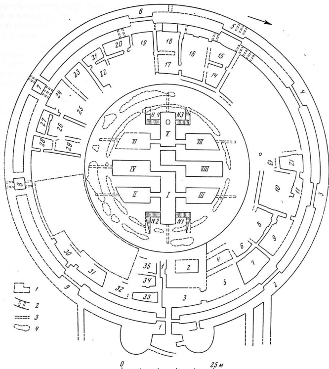
Рис. 7. План центрального здания и застройки вокруг него. Нижний горизонт 1 — неоскрытые участки; 2 — бойницы в стенах стрелковой галереи нижнего кольца; 3 — окна, прорезанные во внешней стене центрального здания; 4 — останцы стен второго этажа центрального здания; I—VIII — помещения первого этажа центрального здания; № 1—4 — лестницы. В тексте помещения нижнего горизонта обозначены с индексом Н (Н1, Н2 и т. д.), опущенным на плане
