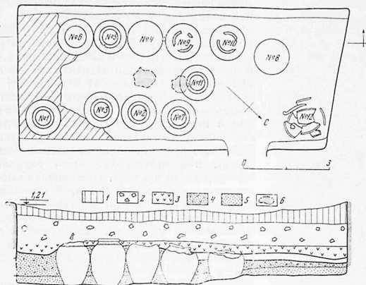
Рис. 33—34. Помещение Н20 с хумами. План и разрез
