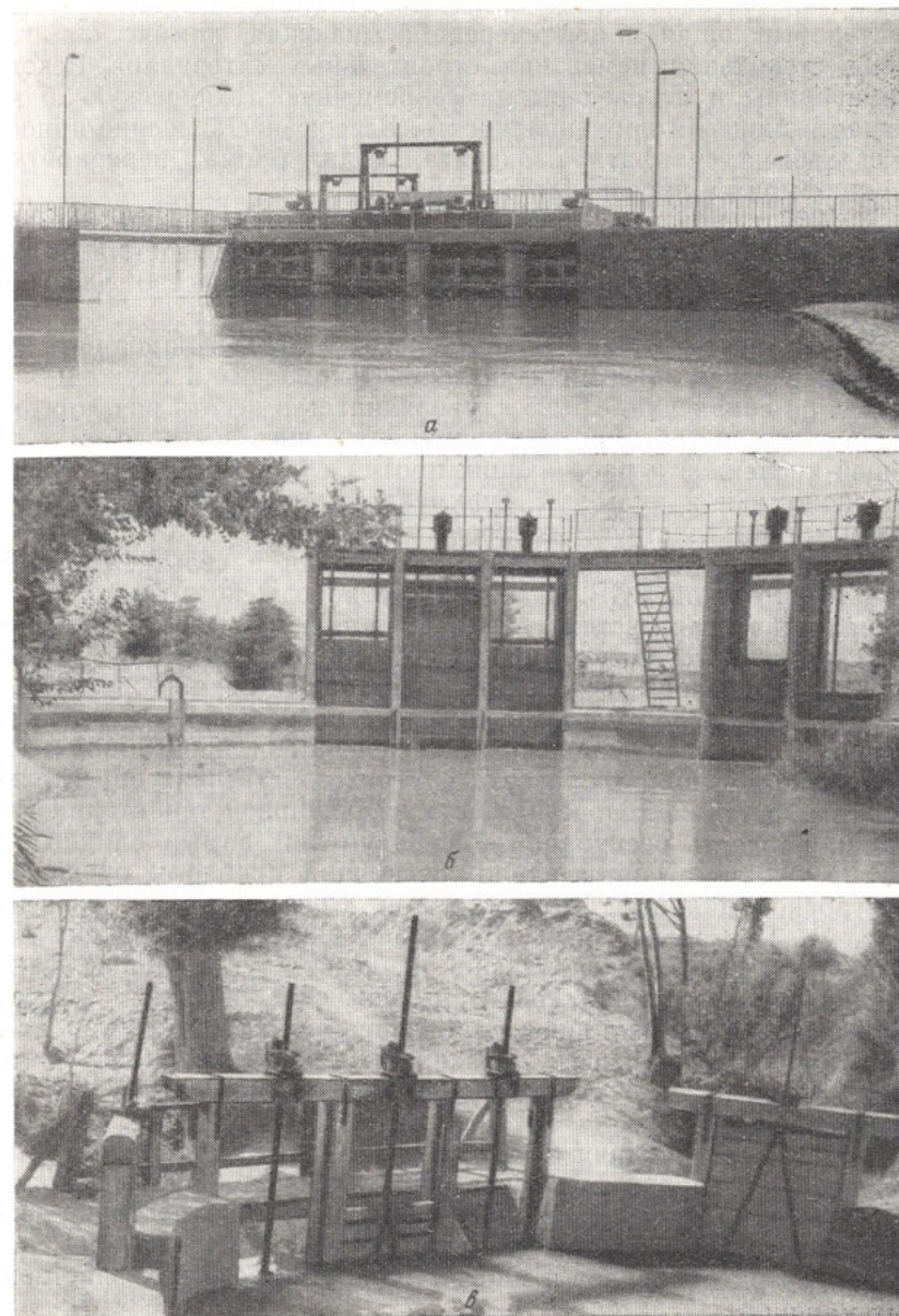
Рис. 1. Ирригационные сооружения:
