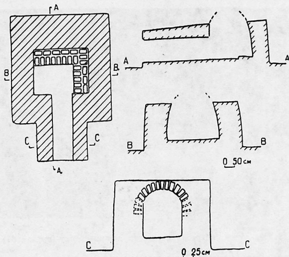
Рис. 3. План и разрезы гробницы (курган 67).
