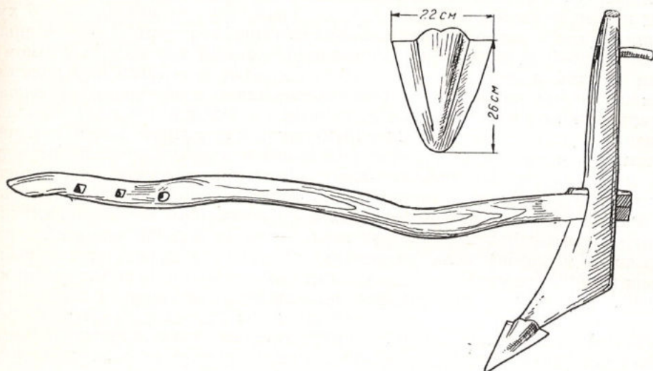
Рис. 16. Деревянная соха (умóч).
