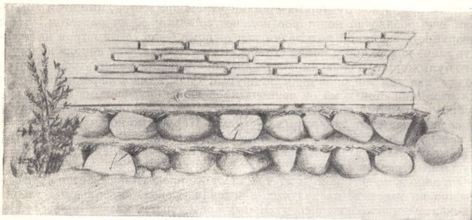
Рис. 36. Кладка цоколя и стены с перекладкой цыновками.
