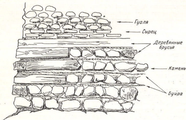
Рис. 37. Крепление углов цоколя.
