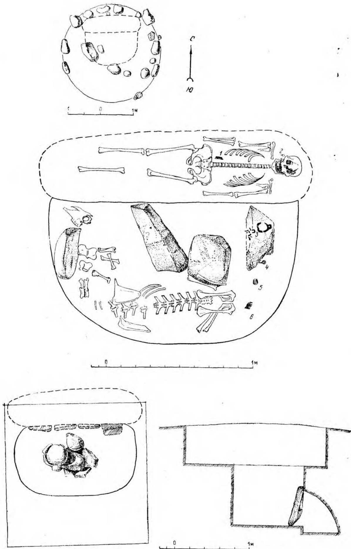
Рис. 44. Центральный Тянь-шань, Нарын, Аламышик. К 69. Планы и разрез. 1 — 3, 4, 5 — фрагменты ножей, удил, стремли и пряжек; 2 — бронзовая серьга; 6 — костяная обкладка лука.
