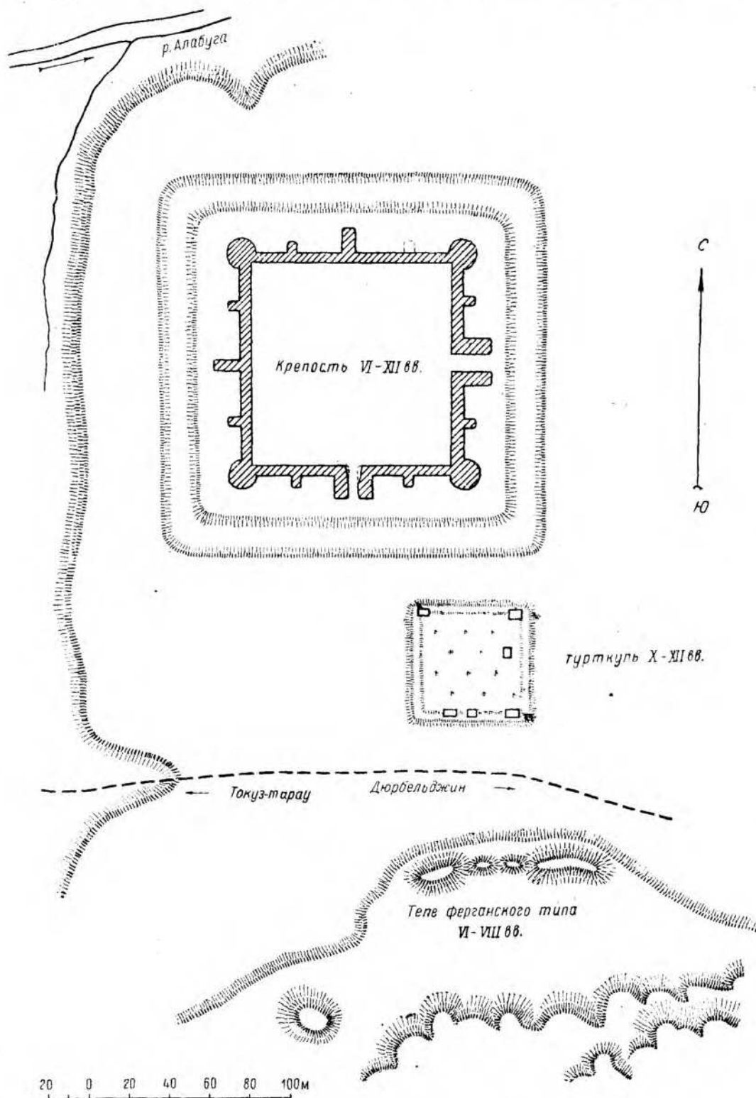
Рис. 54. Центральный Тянь-шань, долина р. Алабуки, Ширдакбек. План городища.
