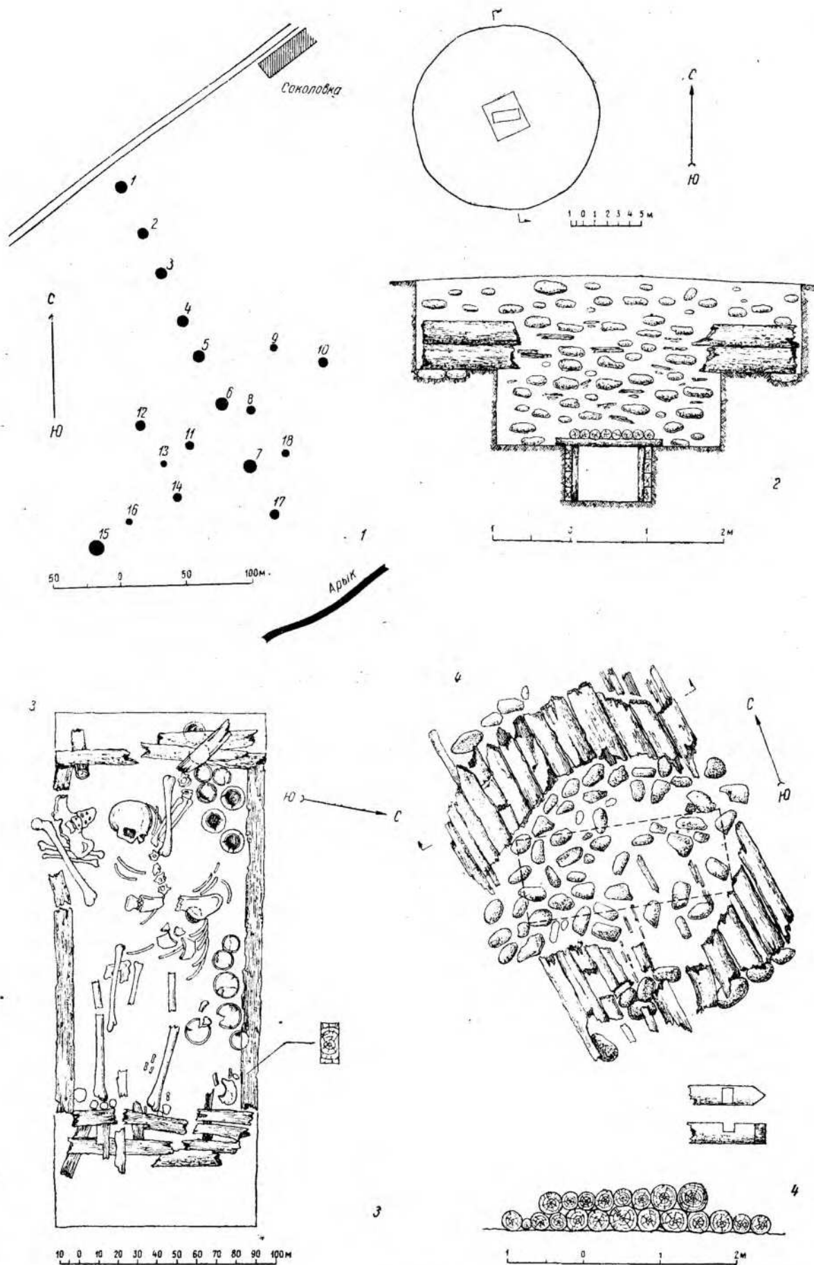
Рис. 22. Тянь-шань, долина р. Джаргелан, Соколовка. План могильника, план и разрезы К 5. 1 — план могильника; 2 — план и разрезы К 5; 3 — план погребальной камеры; 4 — бревенчатый накат.
