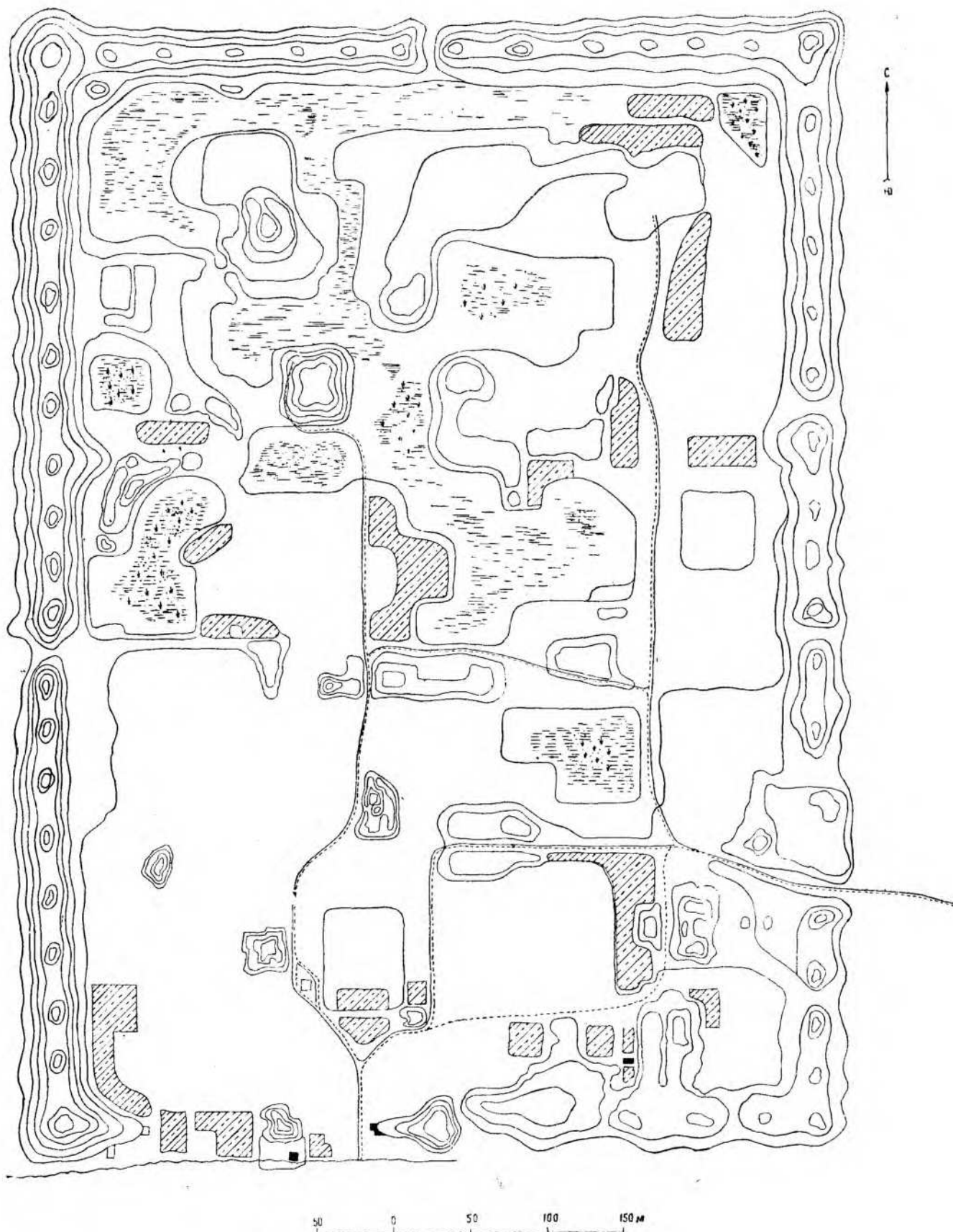
Рис. 89. Фергана, Мархаматское городище. План.
