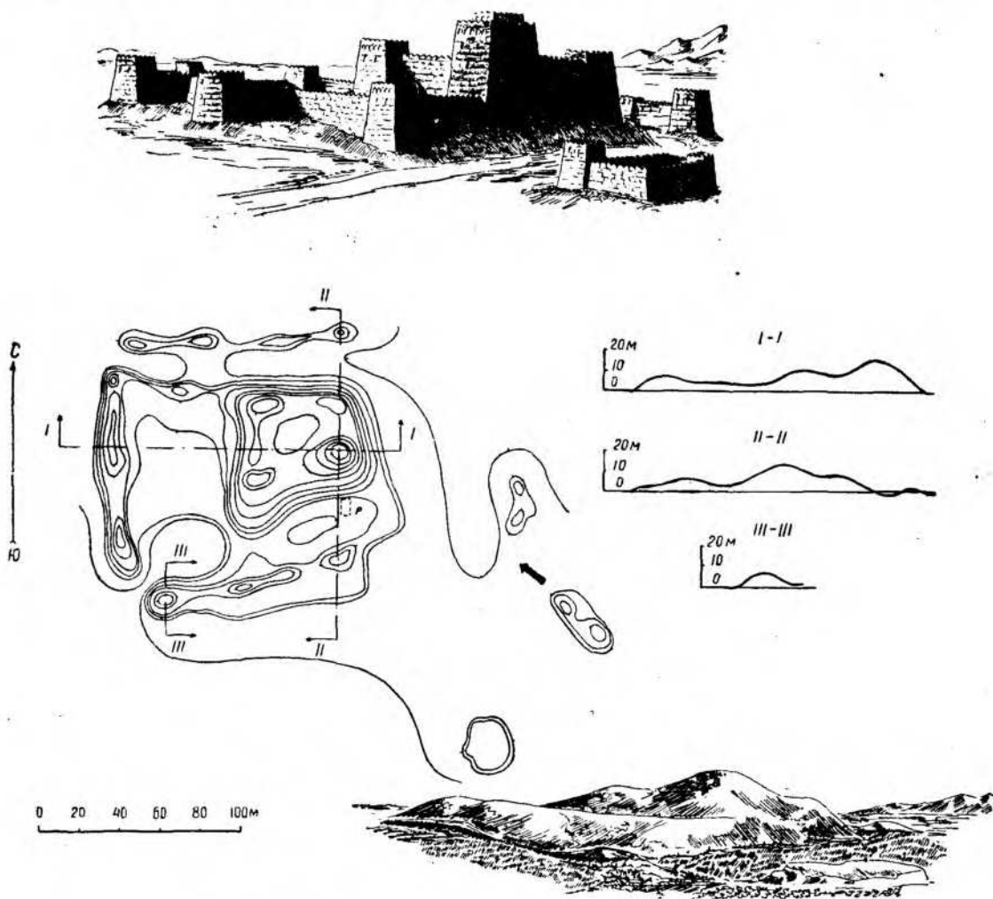
Рис. 105. Фергана, Кургаши́н-тепе. План и реконструкция.
