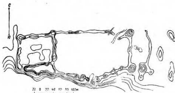
Рис. 61. Кетмень-тубе, городище Ничке. План.
