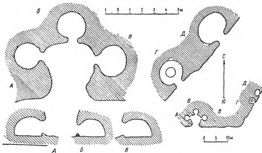
Рис. 111. Фергана, Узген. Жилые пещеры городища. План.
