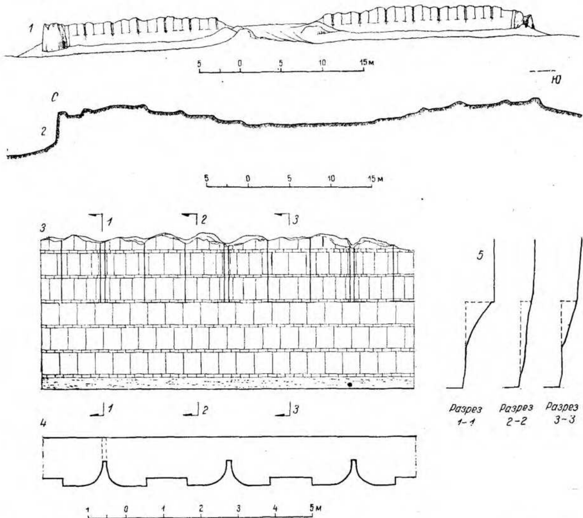
Рис. 57. Центральный Тянь-шань, долина р. Манакельды, городище Чалдывар. Разрезы и детали.
