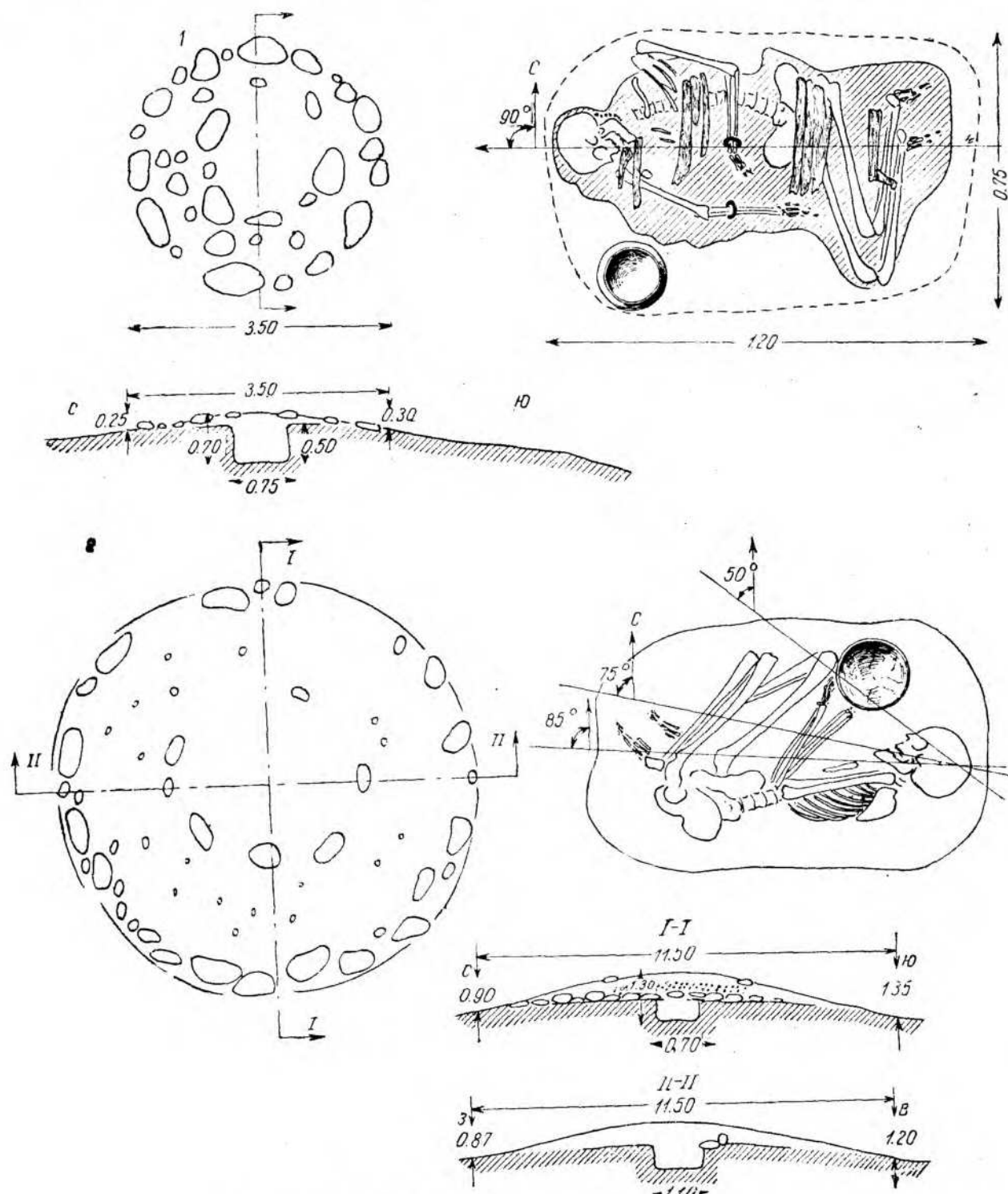
Рис. 123. Восточный Памир, Памирская I. Планы и разрезы.
