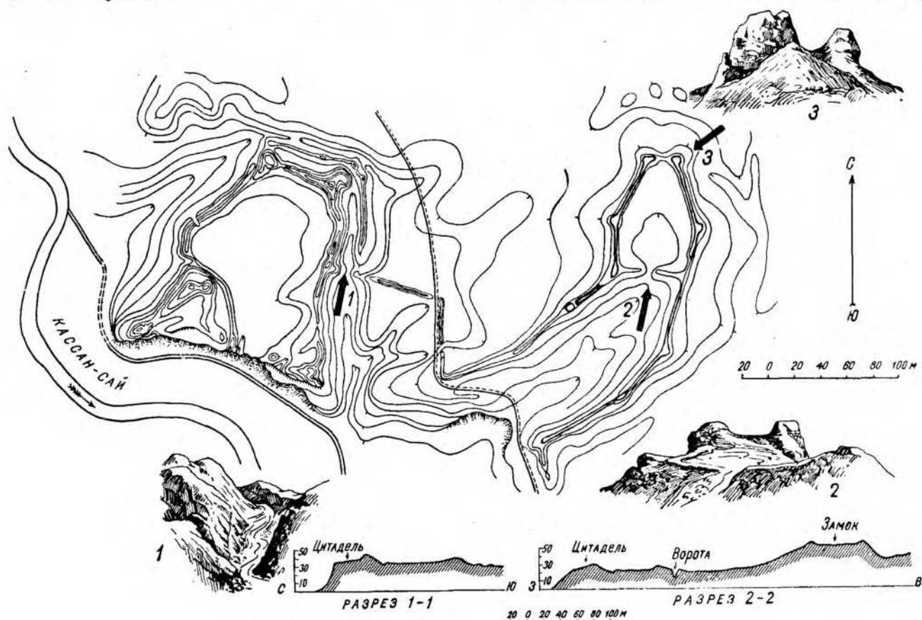
Рис. 94. Фергана, Касан. План и разрезы городища.
