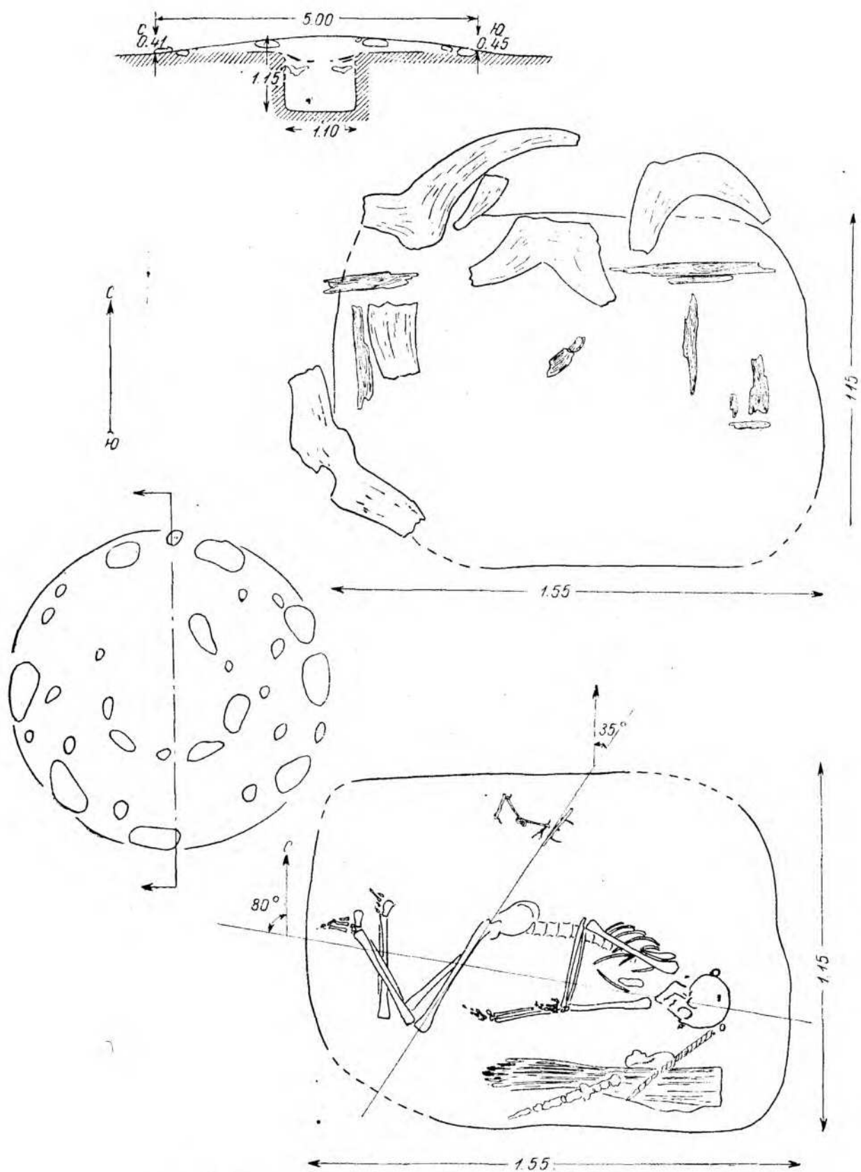
Рис. 127. Восточный Памир, Памирская I, К 10. План и разрезы.
