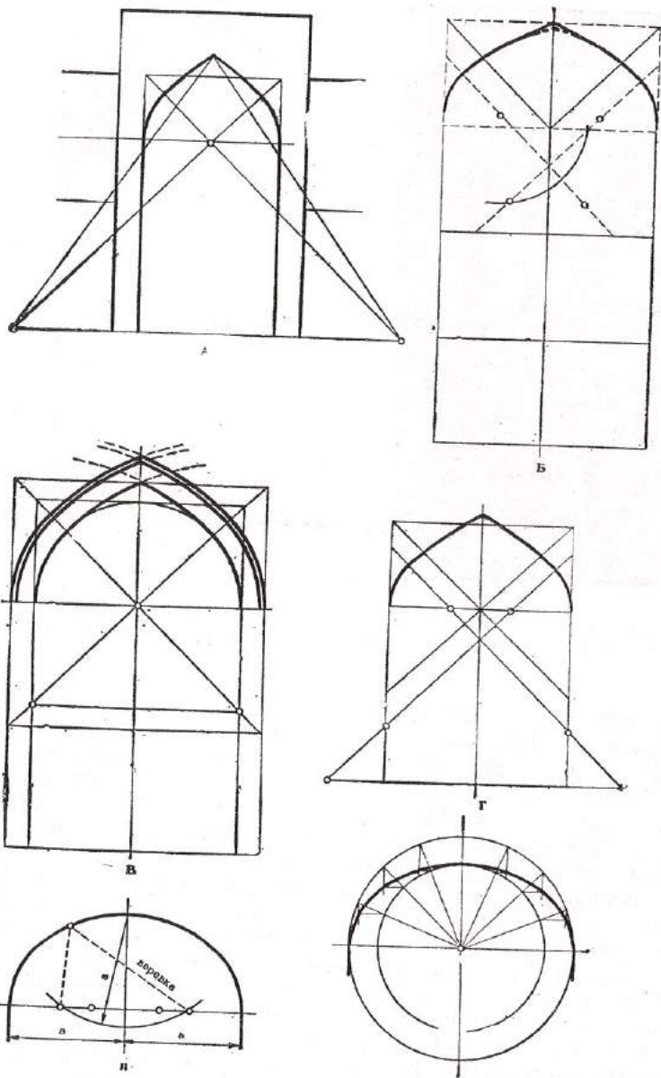
Своды: а) южный портал медресе Улугбека (XV в.) трехцентровая арка «линг тез», б) портал мавзолея Буянкулихана (XIV в.), четырехцентровая арка; в) главный портал медресе Абдулазизхана (XVII в.), трехцентровая арка; г, д, е) построения коробовой кривой «гаври линга» (эллипс).
