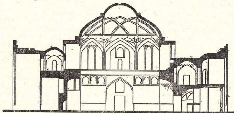
Купольные системы: а) Токи Саррофон, б) Токи Тильпакфурушон, в) Хонако Бахаведдин (XVI в.).
