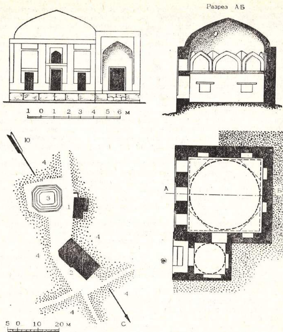
Мактаб в гузаре Кози Фойзи. План, фасад и разрез
