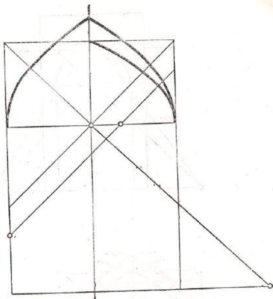
Построение арок на фасаде м. Калон (XVI в.): фотография двух арок, расчищенных на западном фасаде мечети; построение арок двух типов («лингга тез» и «лингга шалгами»).
