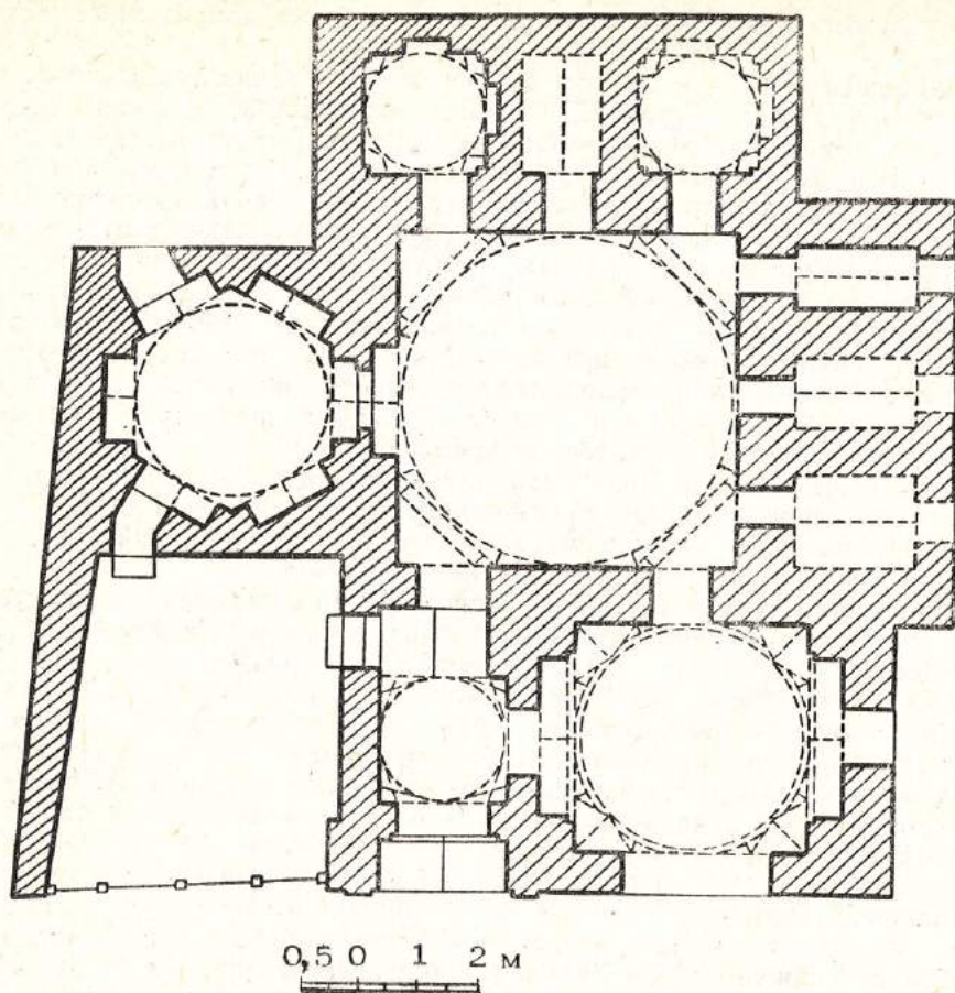
Мактаб XVI—XVII вв. План.
