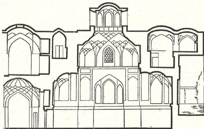
Купольные системы: медресе Мир-Араб и Кукалдош.
