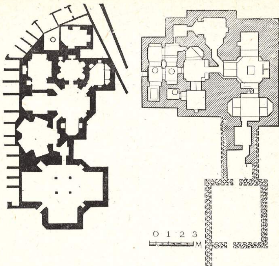
Бани Мисгарон и Чашма-Аюб. Планы.
