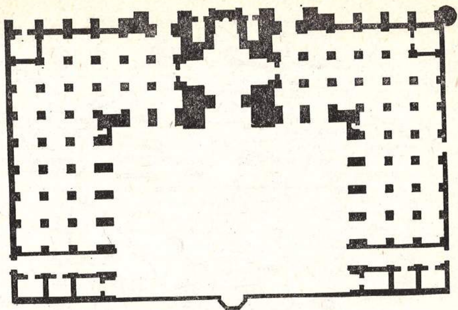
Мечеть Поянда Аталык. План.
