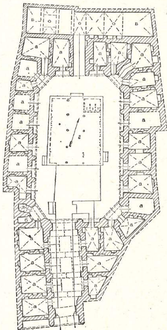
Караван-сарай Кулюта. План.
