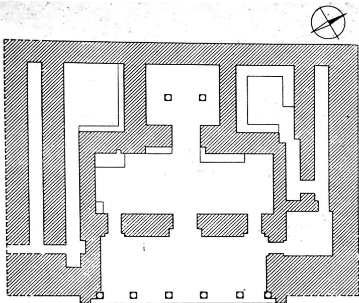
Рис. 32. План парадной постройки в Халчаяне (по Г. А. Пугаченковой)
