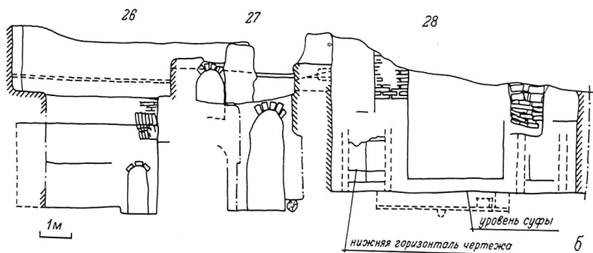
Рис. 52. Объект XXV. Дом с зернохранилищем.
