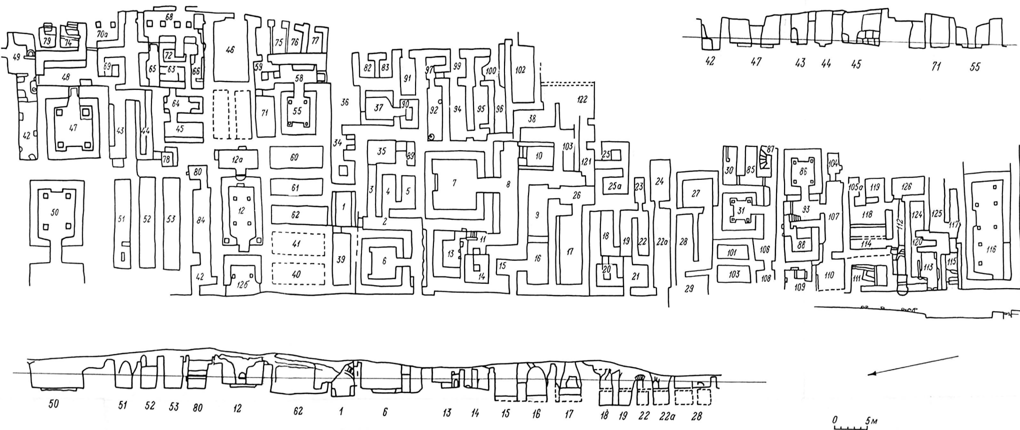
Рис. 5. Объект III. План и разрезы северной части (по: Виронина, 1964, рис. 1).
