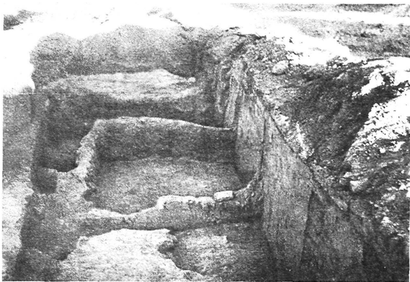
Рис. 51. Объект XXV. Остатки конструкций зернохранилища на 2-м этаже (помещение 4).
