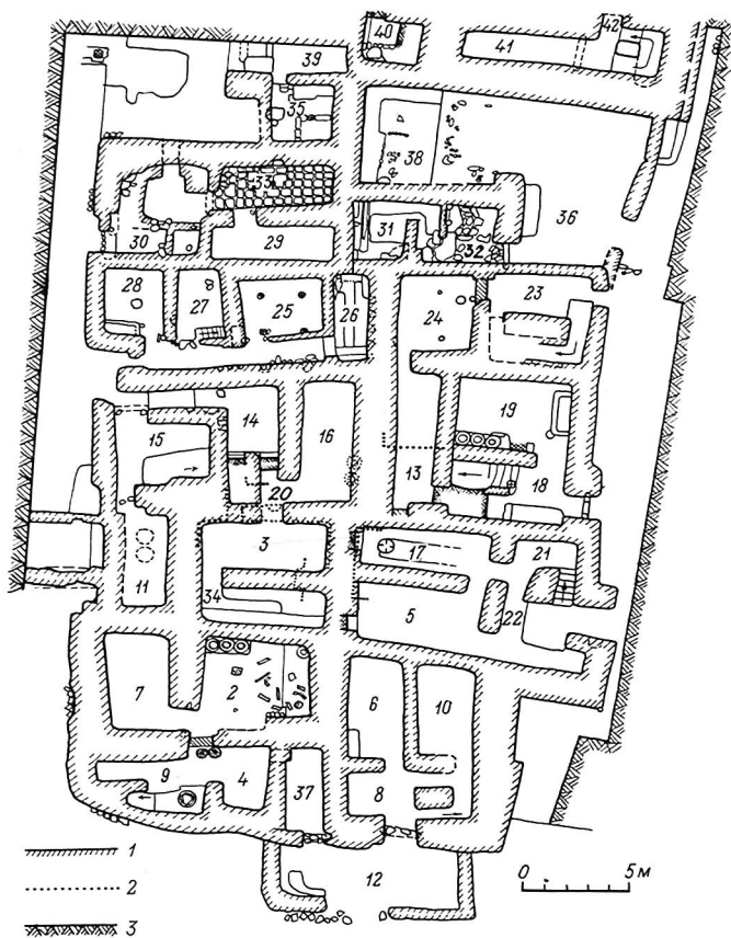
Рис. 16. Объект XII. Верхнее здание. План квартала.
