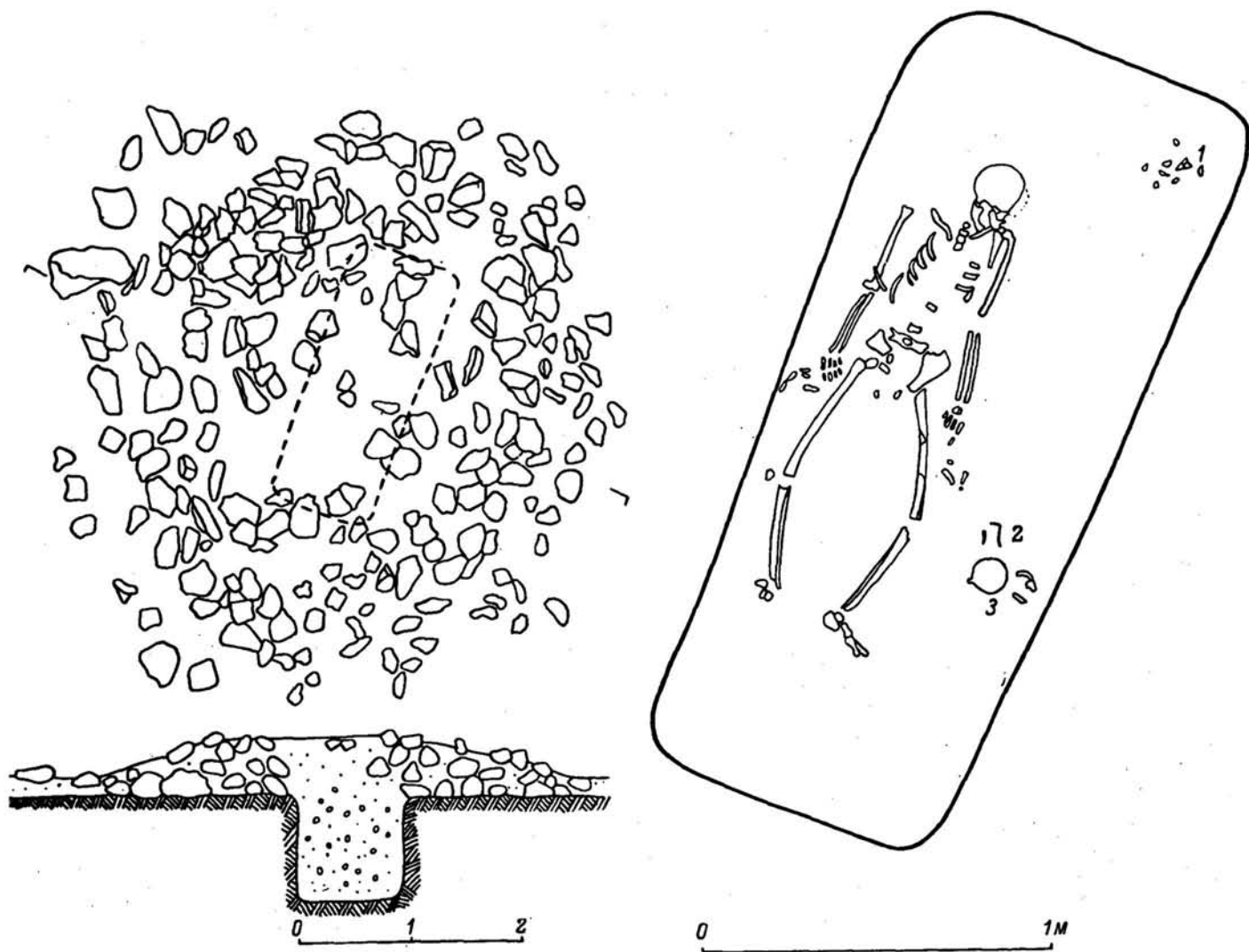
Рис. 46. Бабашовский могильник. Ограда XIII, 4 — план и разрез.
