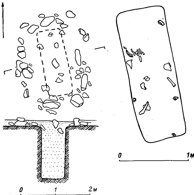
Рис. 32. Бабашовский могильник. Ограда IV, 1 — план и разрез.
