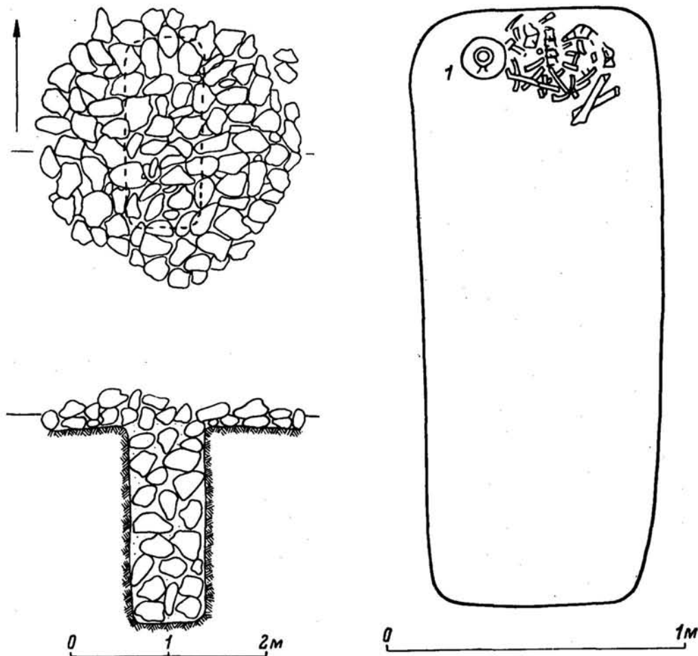
Рис. 3. Аруктауский могильник. Курган V, 1 — план и разрез.
