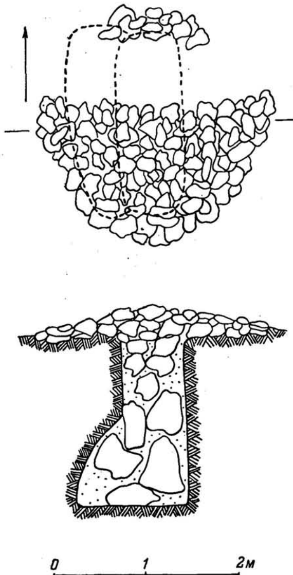
Рис. 22. Аруктауский могильник. Курган XIV, 2 — план и разрез.
