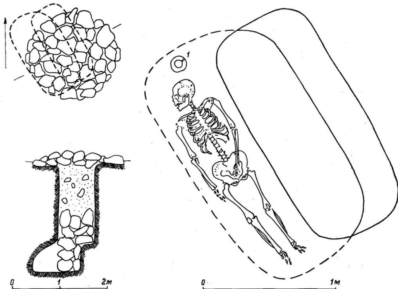
Рис. 19. Аруктауский могильник. Курган X, 5 — план и разрез.
