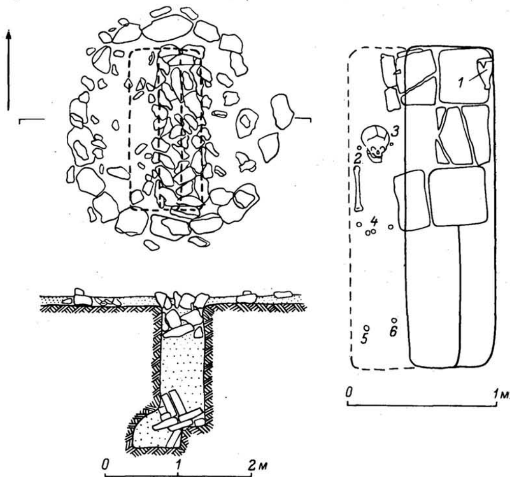
Рис. 34. Бабашовский могильник. Ограда IV, 8 — план и разрез.
