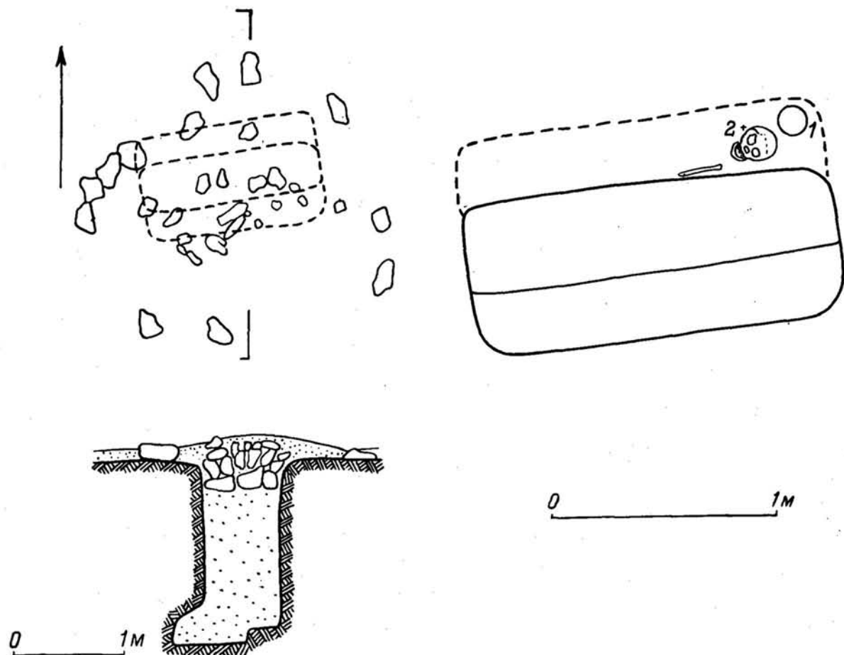
Рис. 47. Бабаховский могильник. Ограда XIV, 2 — план и разрез.
