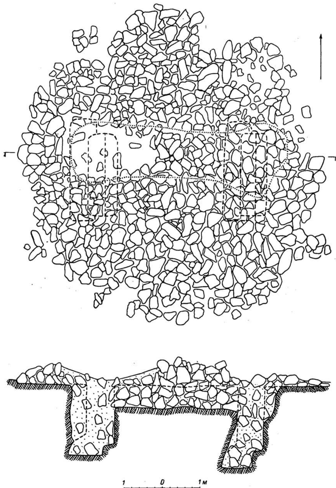
Рис. 28. Коккумский могильник. Кургan 6 — план и разрез.
