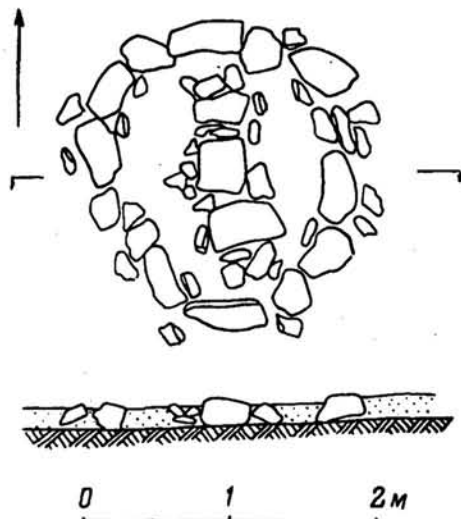
Рис. 33. Бабаховский могильник. Ограда IV, 4 — план и разрез.
