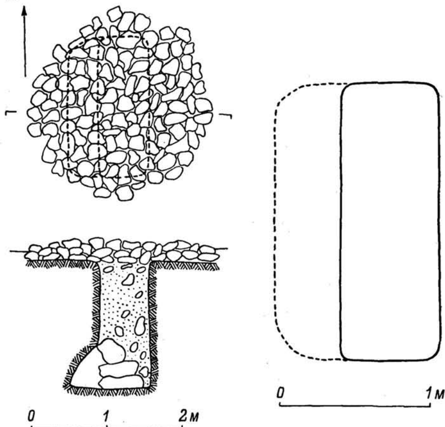
Рис. 25. Аруктауский могильник. Курган XX, 1 — план и разрез.
