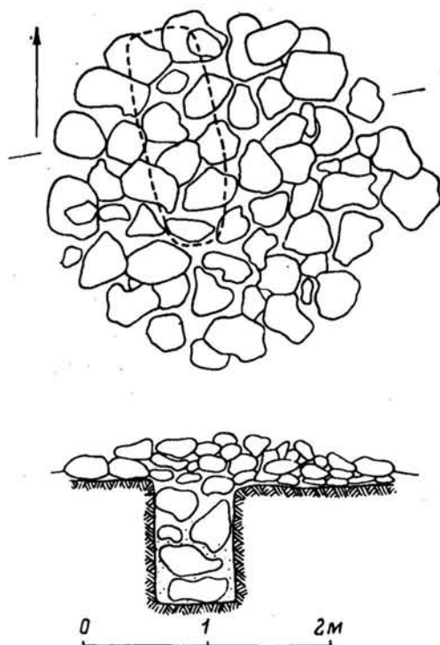
Рис. 16. Аруктауский могильник. Курган IX, 4 — план и разрез.
