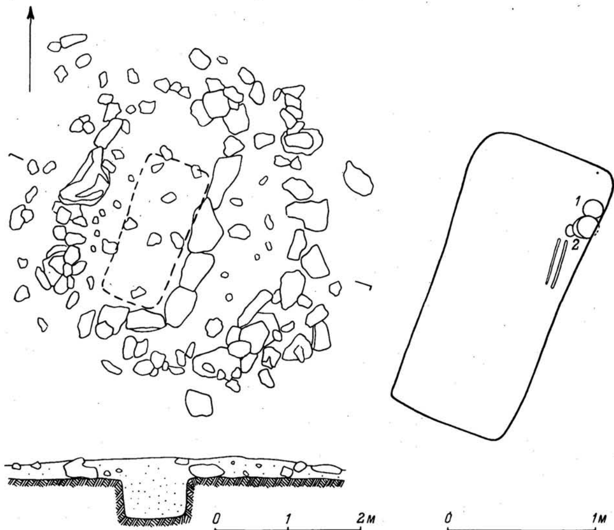
Рис. 36. Бабашовский могильник. Ограда VI, 3 — план и разрез.
