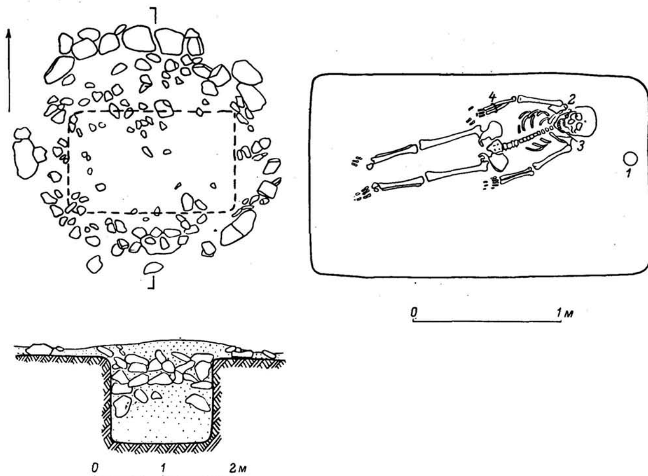
Рис. 49. Бабаховский могильник. Ограда XIV, 21 — план и разрез.
