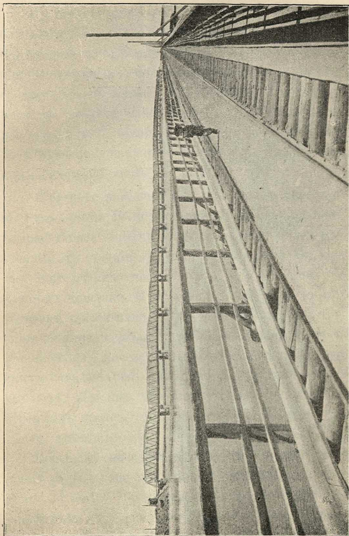
Остатки старого деревян. аму-дарьинскаго моста. Вдали новый аму-дарьинскій жел.-дор. мостъ.
