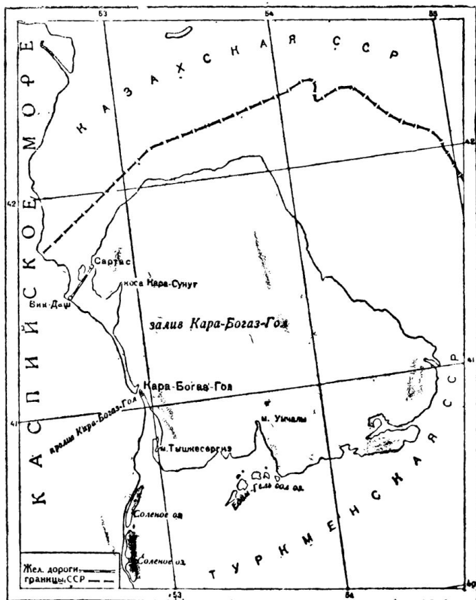
КАРТА ЗАЛИВА КАРА-БОГАЗ-ГОЛ
