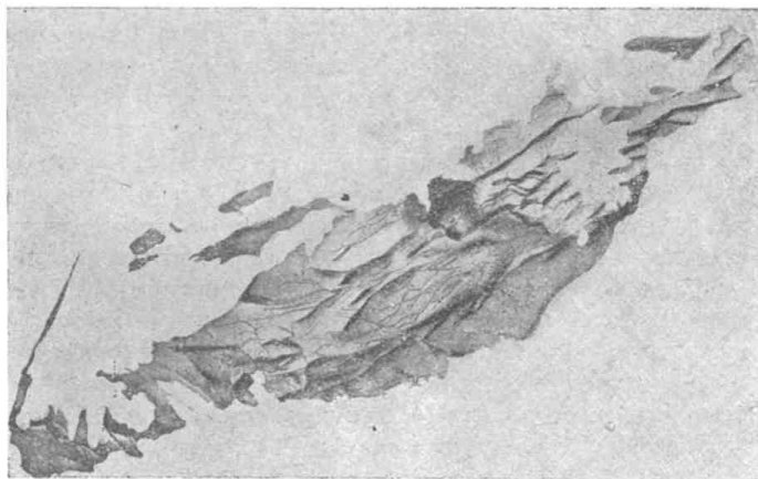
Рис. 29. Схема тектоники Челекена.
