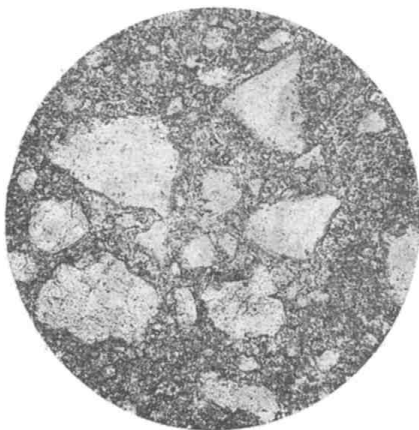
Рис. 46. Рудная брекчия с цементом из кварцплавикового агрегата.
