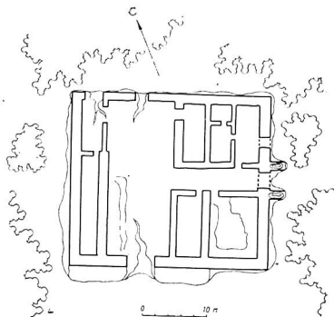
Рис. 30. Усадьба «б» близ Аяз-калы II
