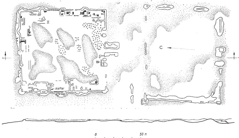
Рис. 35. Усадьба № 5 в Якке-Парасанском оазисе
