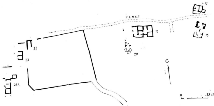
Рис. 78. Комплекс III в поселении Акча-Гелин I
