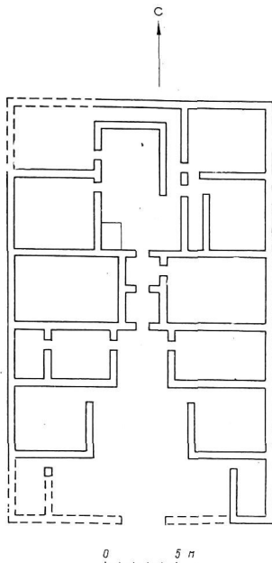
Рис. 44. Безымянный дом в 4,5 км от Джилдымк-калы
