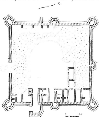
Рис. 37. Безамынный замок в 7,5 км к северо-востоку от Даудан-калы
