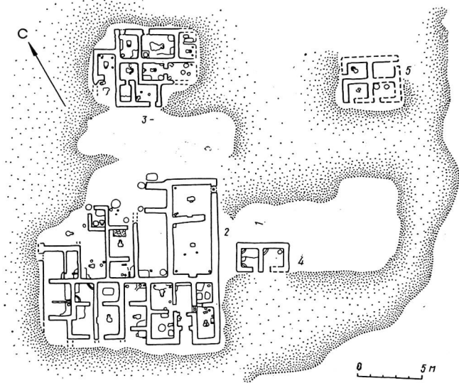
Рис. 57. Группа домов (№ 2, № 3, № 4, № 5) в поселении в урочище Дарьялык-куль
