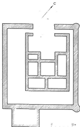
Рис. 6. Здание Турпак-кала III
