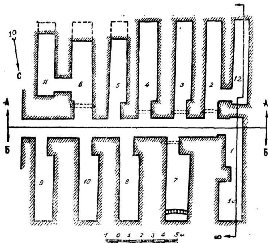
Рис. 12. Городище Калаи Кяхкаха I. Юго-западное здание. Нижний этаж. План.
