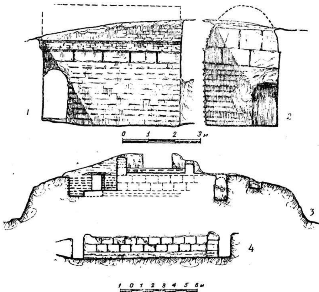
Рис. 25. Городище Калан Кахкаха II. Замок. 1 и 2—разрезы через «Вестибюль» (Е—Е и Ж—Ж); 3—разрез по западной группе помещений и пандусу (Б—Б); 4—разрез по коридору среднего яруса (Г—Г).
