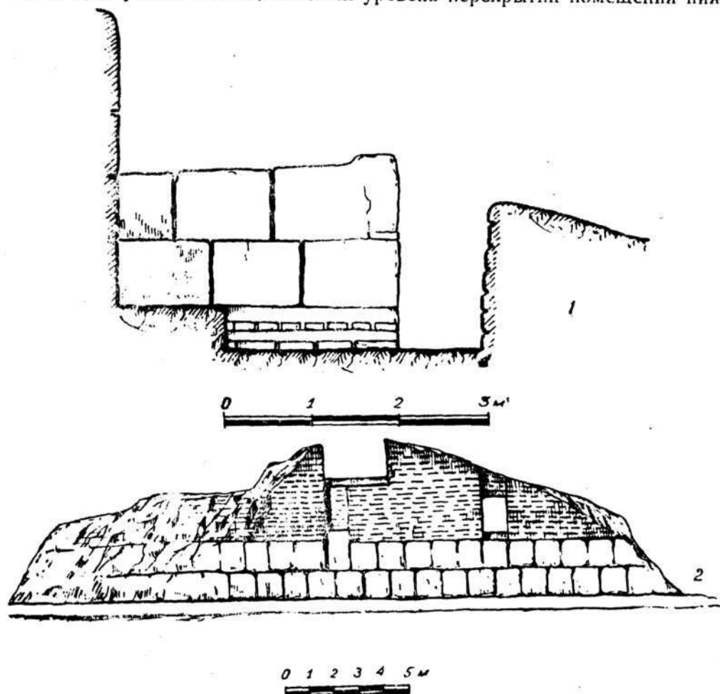
Рис. 40. Городище Калаи Кяхка II. Замок. 1—разрез через помещение № 8; 2—западный фасад.
