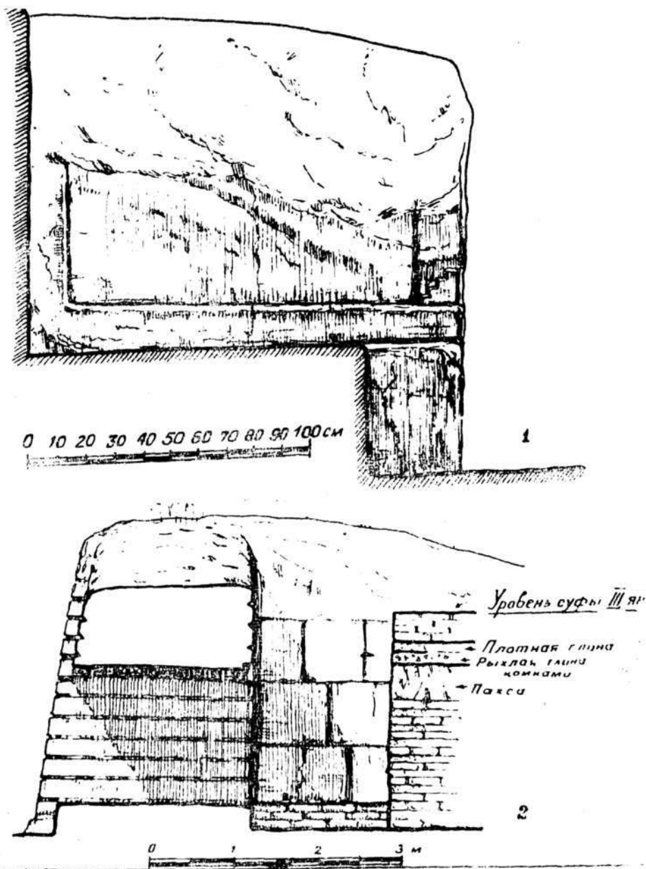
Рис. 33. Городище Калаи Кахкаха II. Замок. 1—помещение № 3. Стенка—ширма. 2—разрез 3—В (И—И) через окно и помещение № 8.
