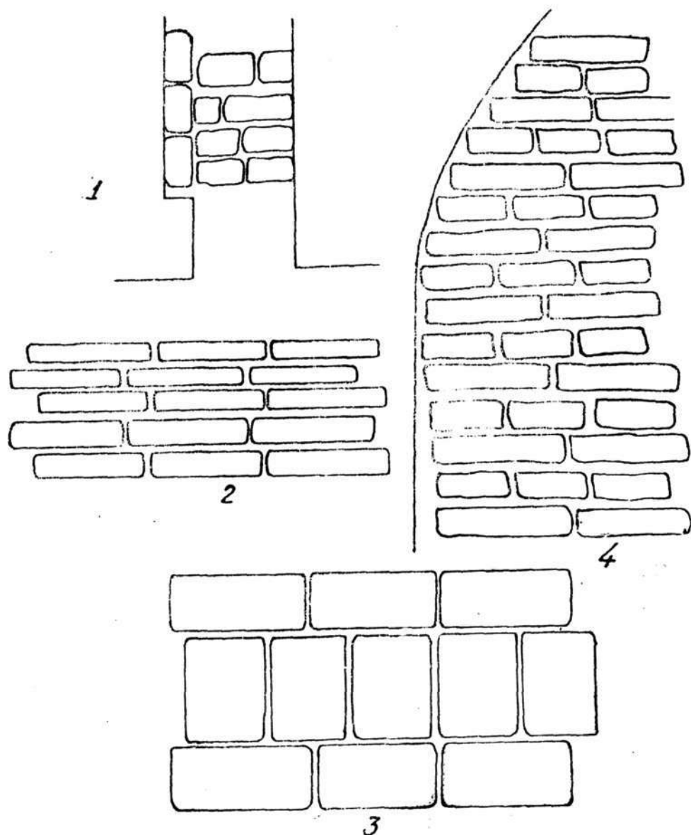
Рис. 14. Городище Калан Кахкаха I. Юго-западное здание. Нижний этаж. Система кладок: 1—горизонтальный срез закладки помещения № 9; 2 и 3—вертикальный и горизонтальный разрезы закладки проема помещения № 10; 4—южная торцовая стена помещения № 1.
