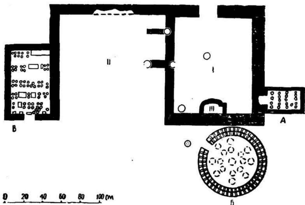
Рис. 4. План керамической мастерской:
