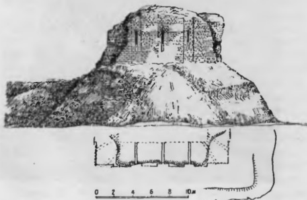
Рис. 35. Угловая северо-восточная башня крепостной стены Топрак-кала (современное состояние)
