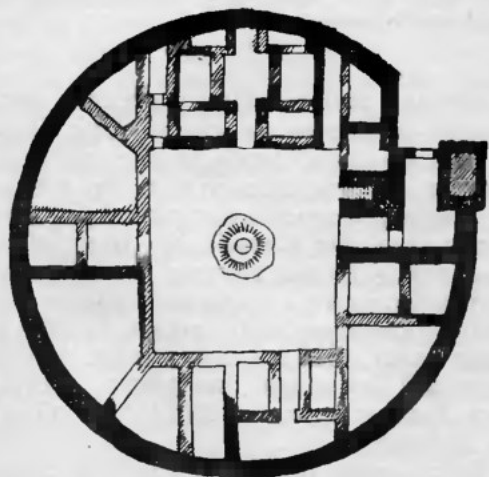
Рис. 186. План пограничной крепости древнего Хорезма Дэу-кала
