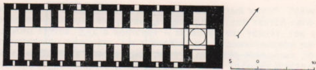
Рис. 27. Окрестности Мерва. Поселение в Дус-Чакын. Постройка «Хароба-Кошук». План по Г. Я. Дресвянской с реконструкцией автора
