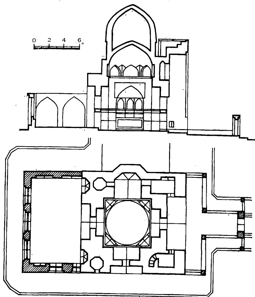
Мавзолей Каффаль Шахи. Разрез, план.
