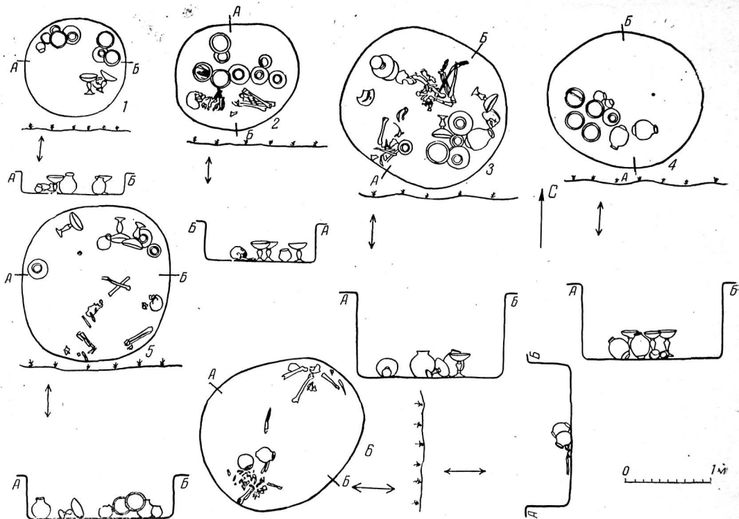
Табл. XII. Планы и разрезы могил, кузалинский этап: 1—мог. 686; 2—697; 3—687; 4—708; 5—679; модалный этап: 6—714.
