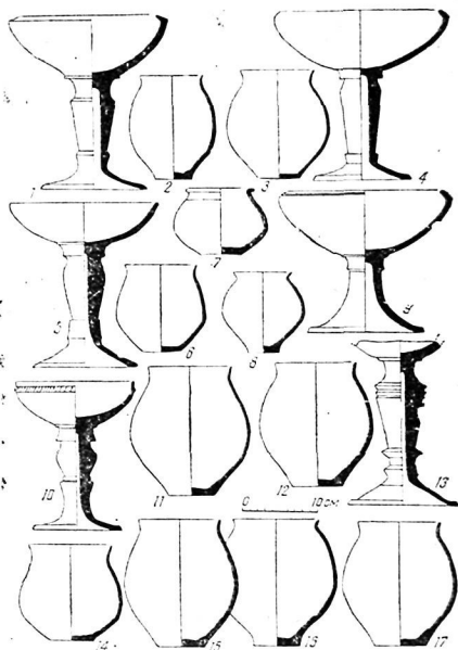
Табл. XLII. Керамика. Комплекс кузалинского этапа: 1—мог. 51; 2, 14—101; 3—484; 4—533; 5—212; 6—201; 7—597; 8—112; 9—3; 10—618; 11—344; 12, 17—453; 13—378; 15—610; 16—697.
