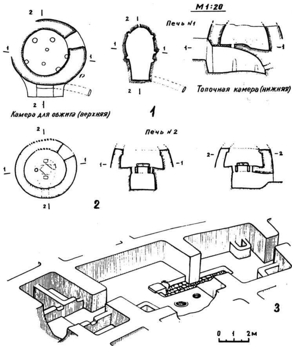
Рис. 33. 1, 2 — керамические печи; 3 — аксонометрия дома в квартале «ЕІ»
