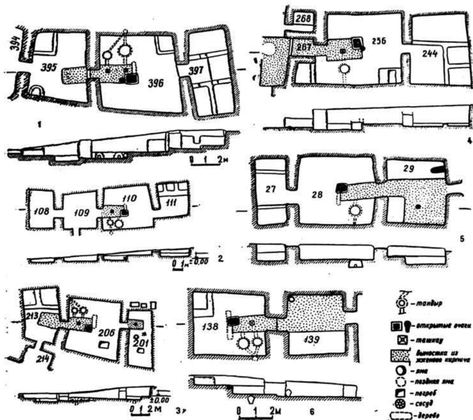
Рис. 24. Планы и разрезы домов: 1 — квартал «ЕI», дом 1; 2 — квартал «Е», дом 1; 3 — квартал «И», дом 3; 4 — квартал «Р», дом 14; 5 — квартал «М», дом 2; 6 — квартал «П», дом 2
