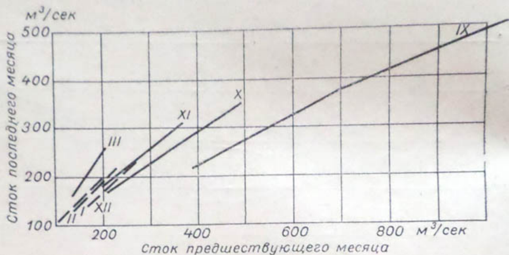
Рис. 46. Зависимость средних месячных расходов воды меженного периода от расходов предшествующего месяца, р. Нарын — пост Уч-Курган.
