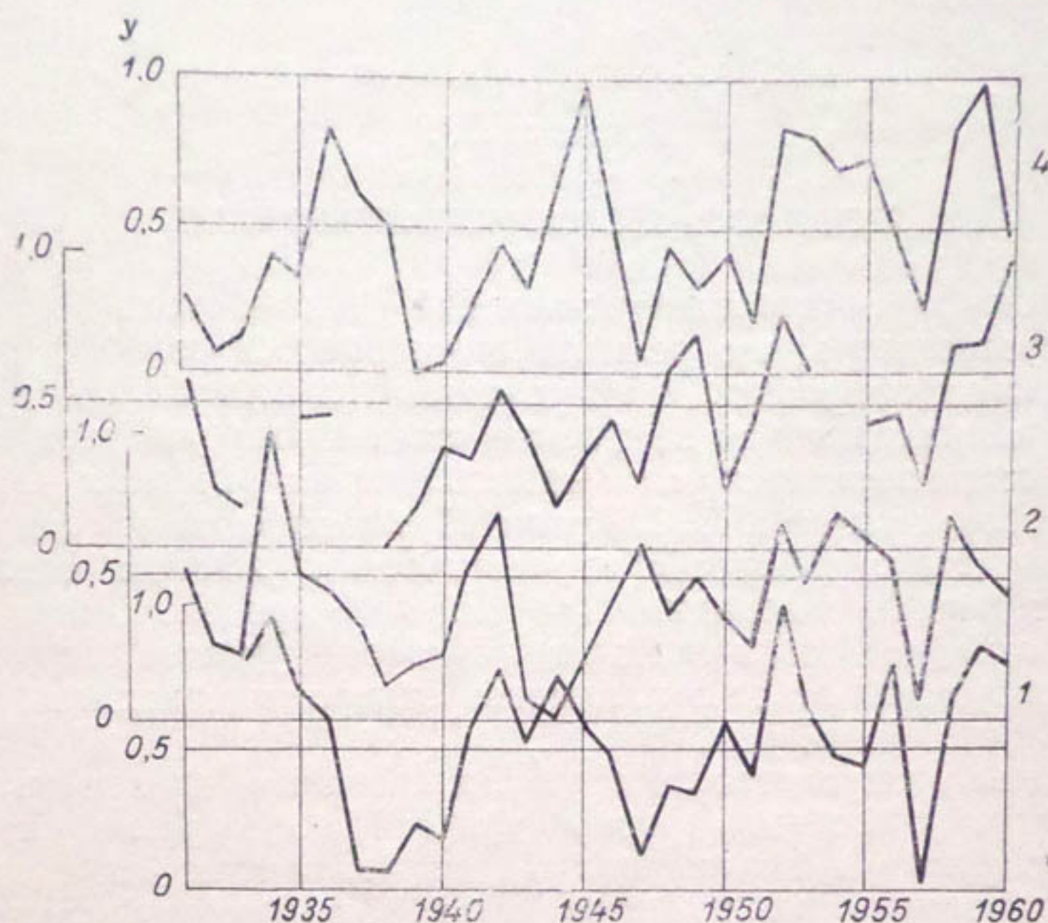
Рис. 55. Хронологический ход годового стока ряда рек.
