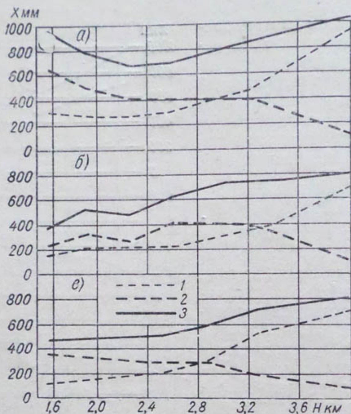
Рис. 24. Распределение зимних (1), летних (2) и суммарных годовых (3) осадков по высотному простиранию бассейна за 1957-58 (а), 1958-59 (б), 1959-60 (в) гг. в рамках естественных осадковых циклов.
