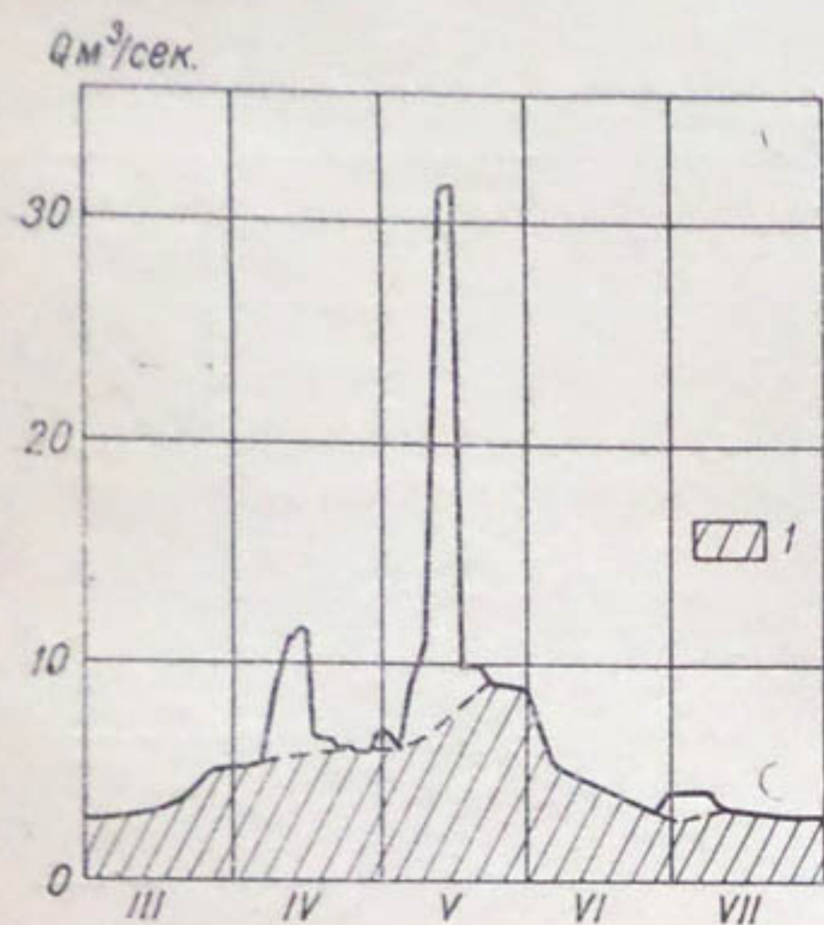
Рис. 16. Сглаженный по скользящим пентадам гидрограф р. Гузардарья за летние месяцы 1951 г. с выделением подземного питания (1).
