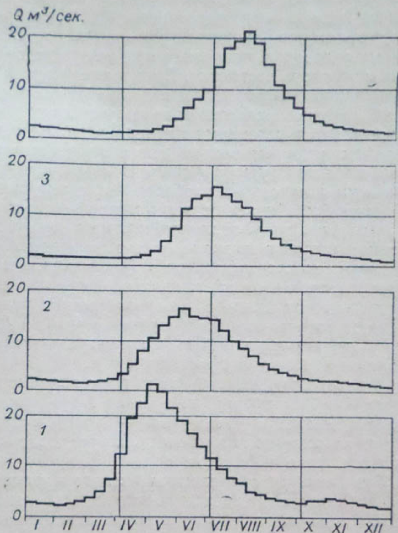
Рис. 41. Гидрографы средних многолетних расходов воды (1936—1960 гг.) рек снего-дождевого (1—Майлису), снегового (2—Падшаата), снего-ледникового (3—Карабалты) и ледникового (4—Джуука) питания.
