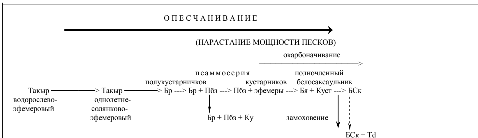
Рис.15. Схема динамических рядов опесчанивания и замоховения
