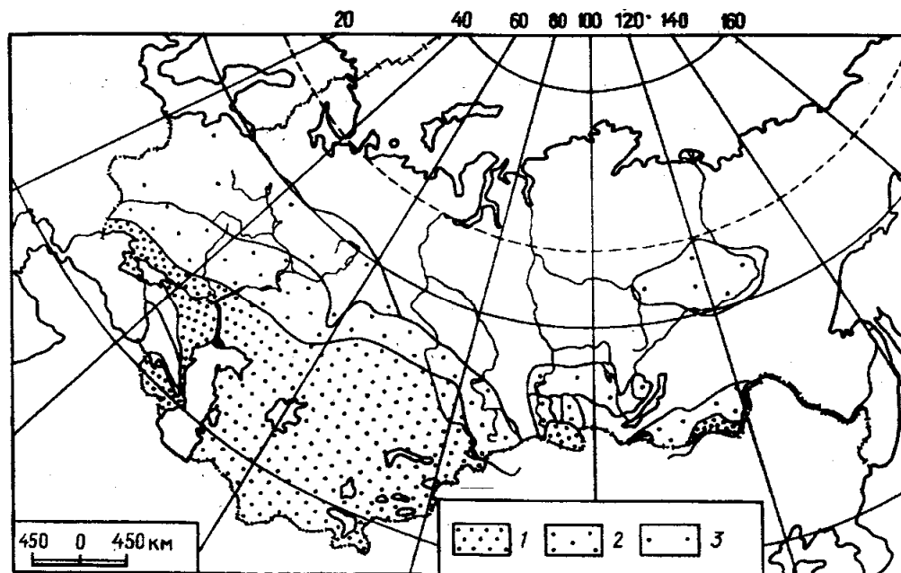
Рис. 57а. Распространение засух, сухие и засушливые регионы на территории бывшего СССР (по Н.Ф.Глазовскому и Н.С.Орловскому, 1996) 1 – регионы с отношением осадков к потенциальной эвапотранспирации < 0.65 , 2 – регионы с частотой засух > 25\% , 3 – регионы с частотой засух < 25\%
