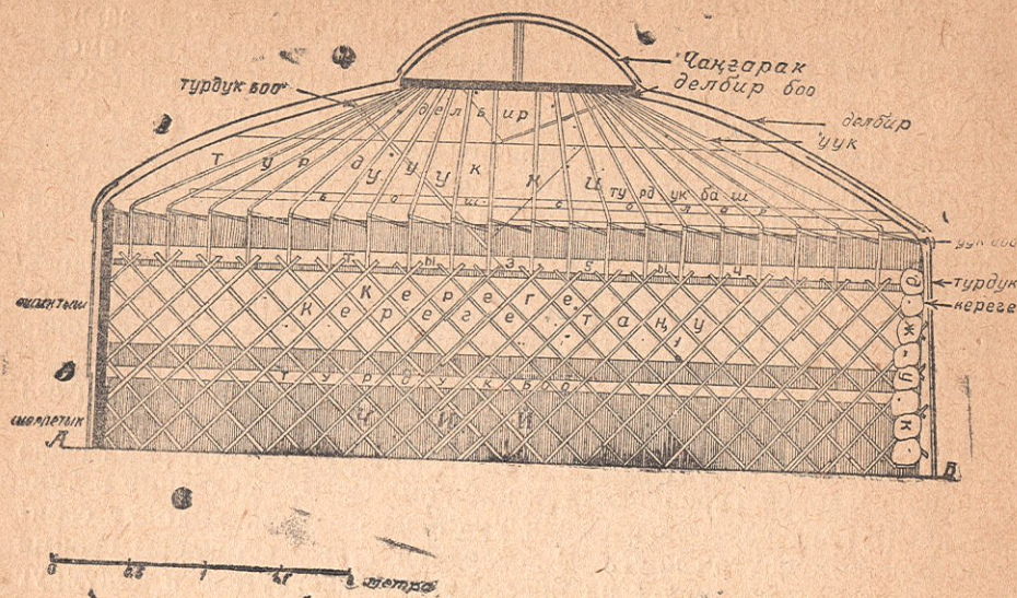
Рис. 3. Разрез юрты Алопаева.
