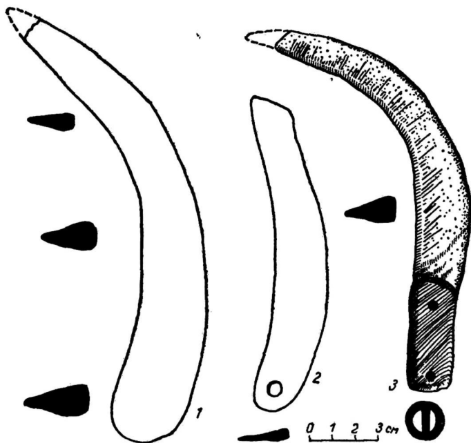
Рис. 30. Каменные орудия:
